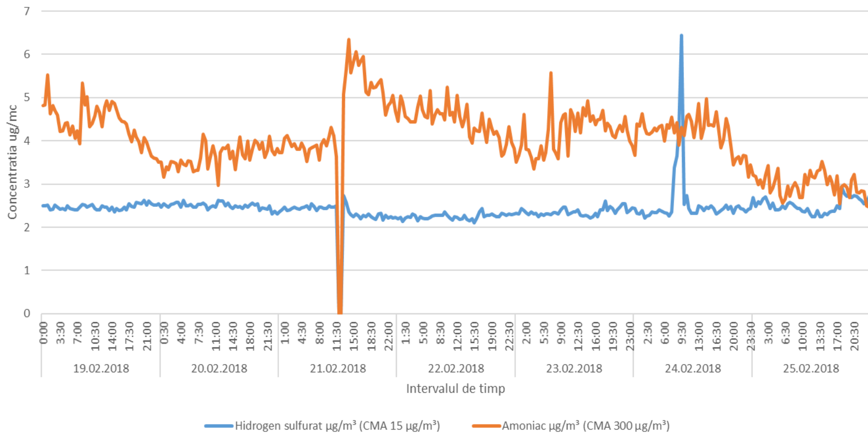
Variatia indicatorilor hidrogen sulfurat si amoniac in perioada 19.02.2018-25.02.2018 in zona de nord/vest a platformei industriale Brazi
