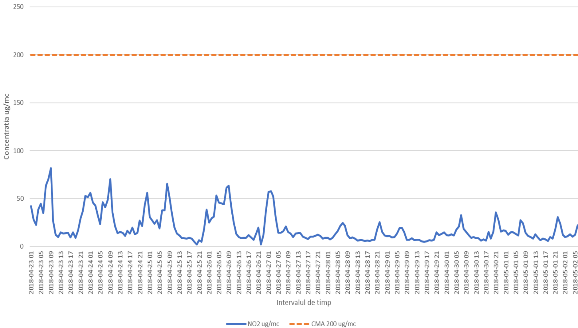
Variatia indicatorului NO2 in intervalul 23.04.2018 - 29.04.2018 in zona de E a platformei industriale Brazi
