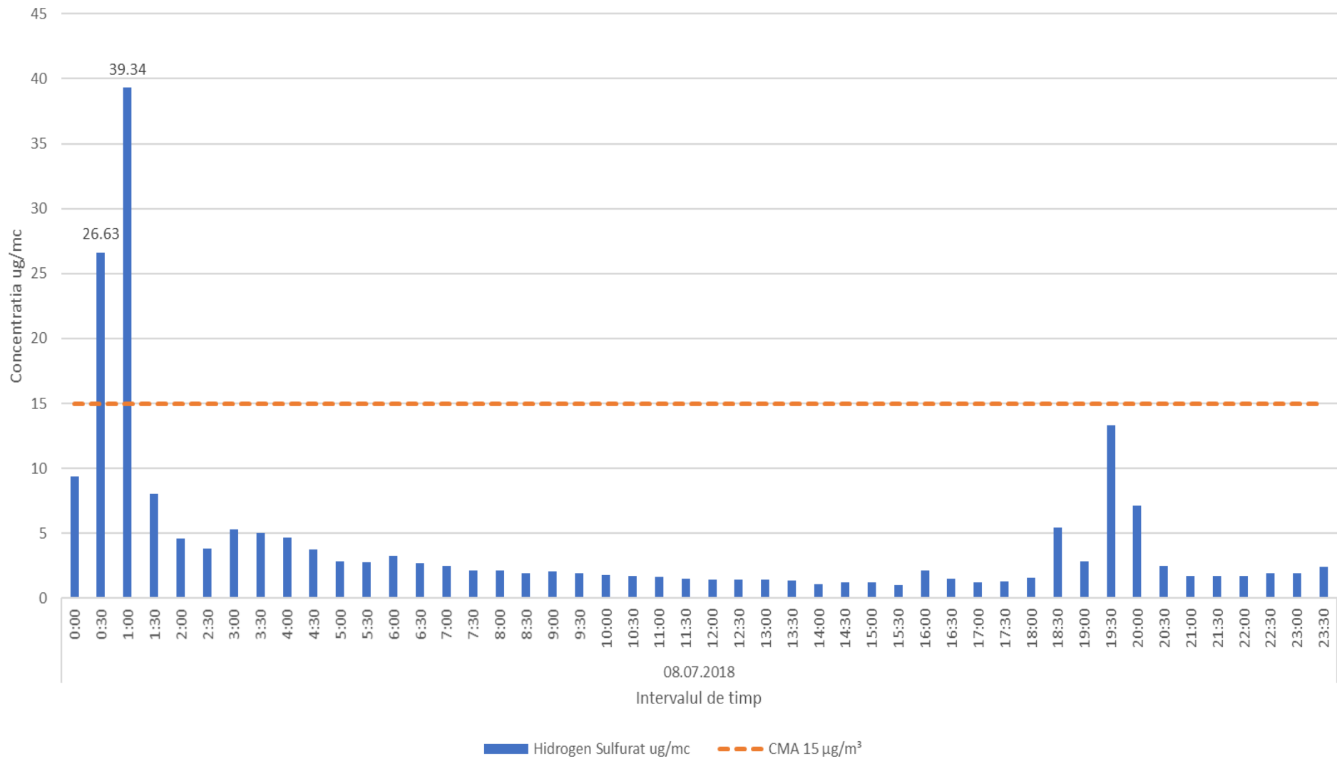
Variatia indicatorului H2S in data de 08.07.2018 in zona de nord a platformei industriale Lukoil
