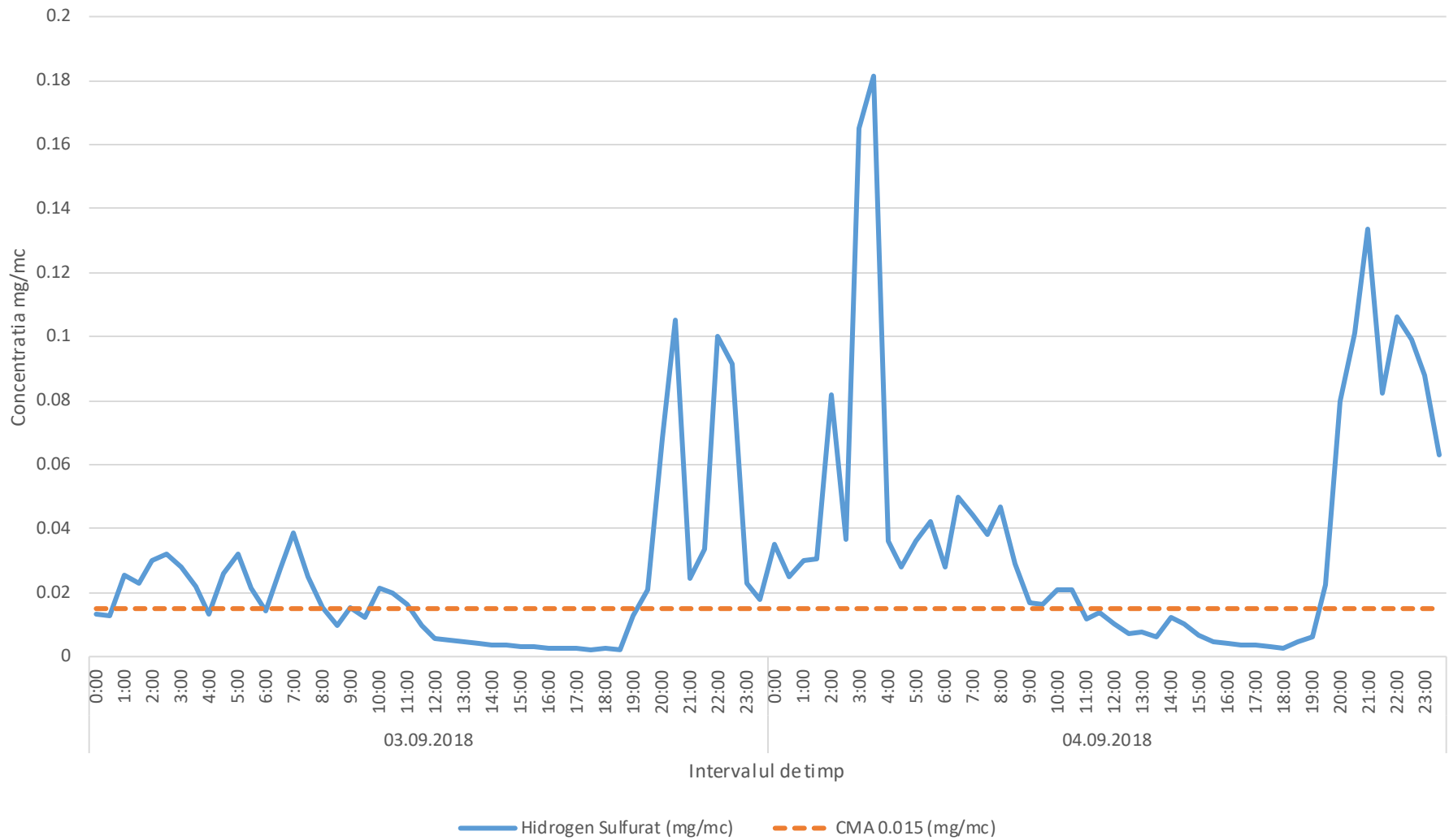
Variatia indicatorului H2S in intervalul 03.09.2018-04.09.2018 in zona platformei ecologice Boldesti Scaieni
