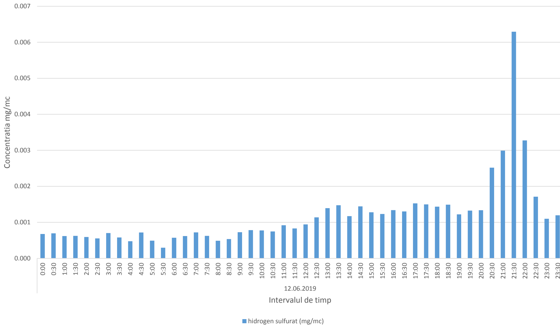
Variatia momentana a indicatorului H2S in data de 12.06.2019 - oras Baicoi, cartier Tintea (Parc 2 Padure)
