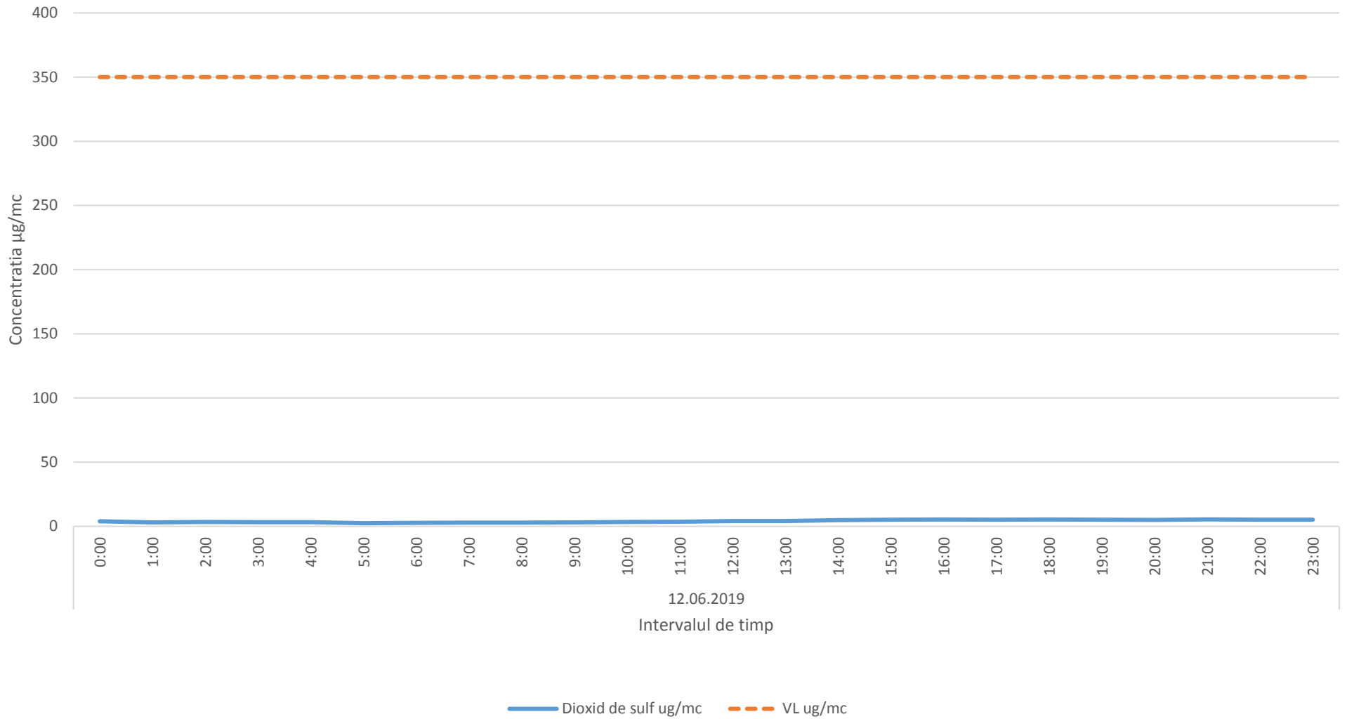
Variatia momentana a indicatorului SO2 in data de 12.06.2019 - oras Baicoi, cartier Tintea (Parc 2 Padure)
