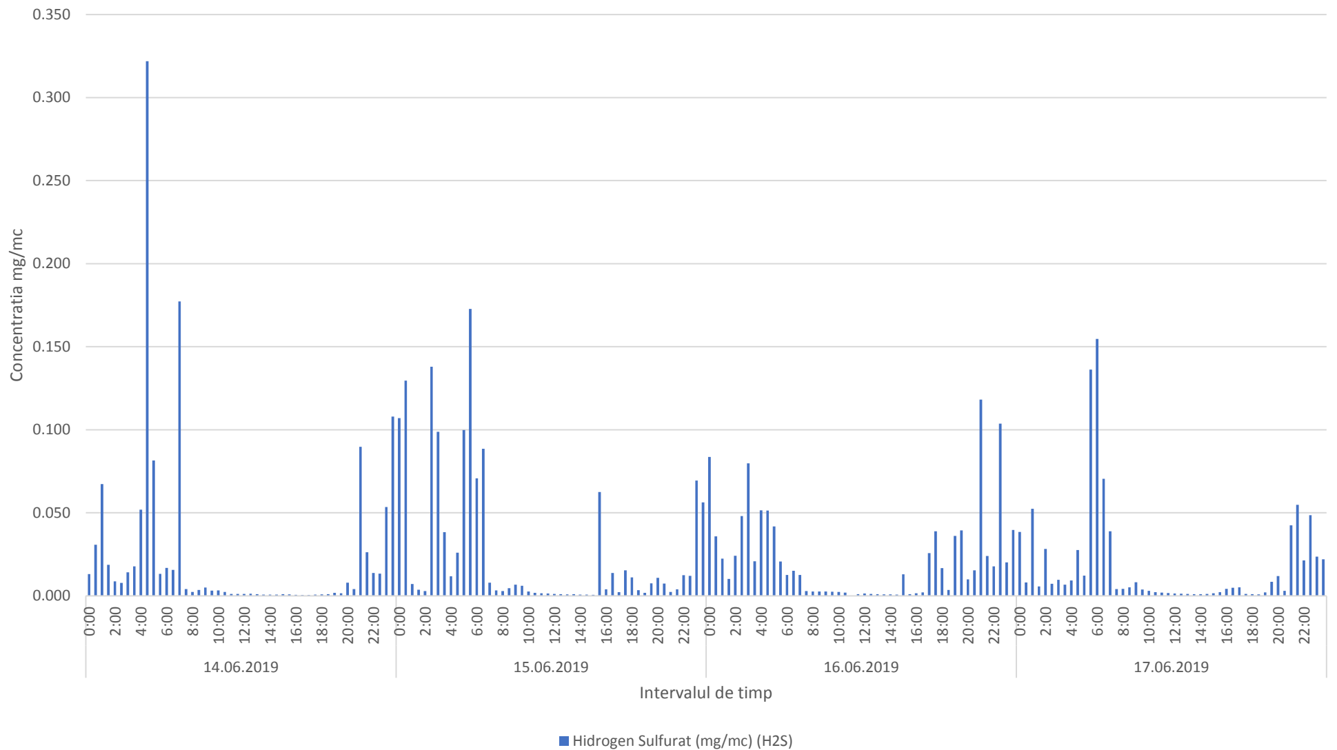
Variatia momentana a indicatorului H2S - intervalul 14.06.2019-17.06.2019 in zona cartierului Tintea, oras Baicoi (Class Beton)
