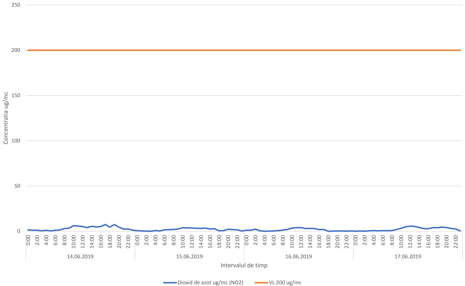
Variatia indicatorului NO2 - intervalul 14.06.2019-17.06.2019 in zona cartierului Tintea, oras Baicoi (Class Beton)
