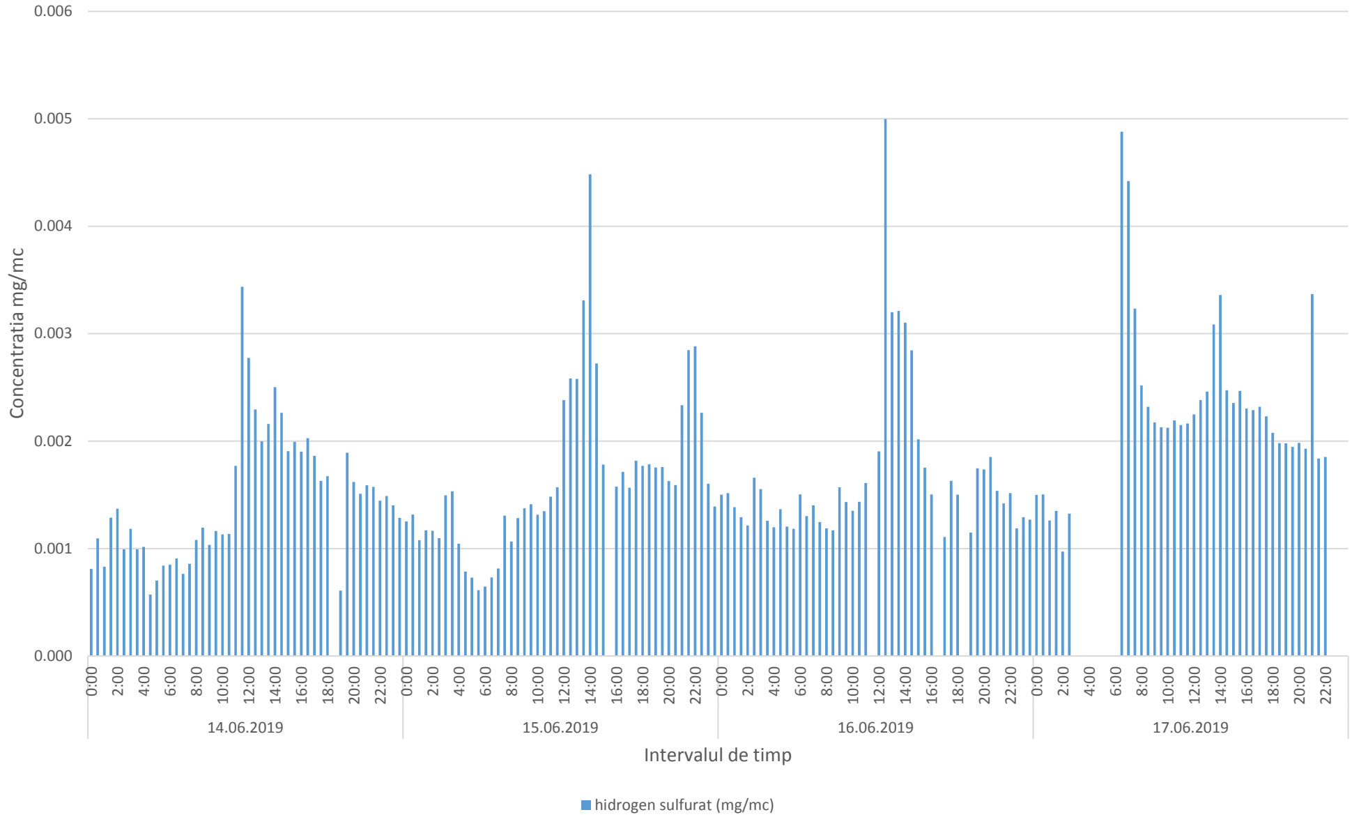
Variatia momentana a indicatorului H2S in intervalul 14.06.2019-17.06.2019- oras Baicoi, cartier Tintea (Parc 2 Padure)
