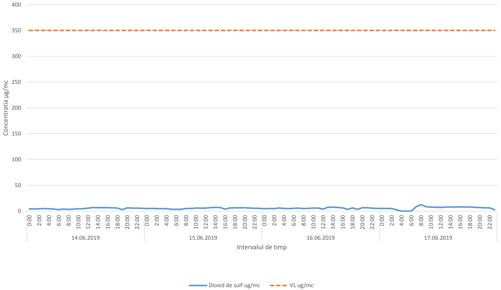
Variatia indicatorului SO2 in intervalul 14.06.2019-17.06.2019- oras Baicoi, cartier Tintea (Parc 2 Padure)
