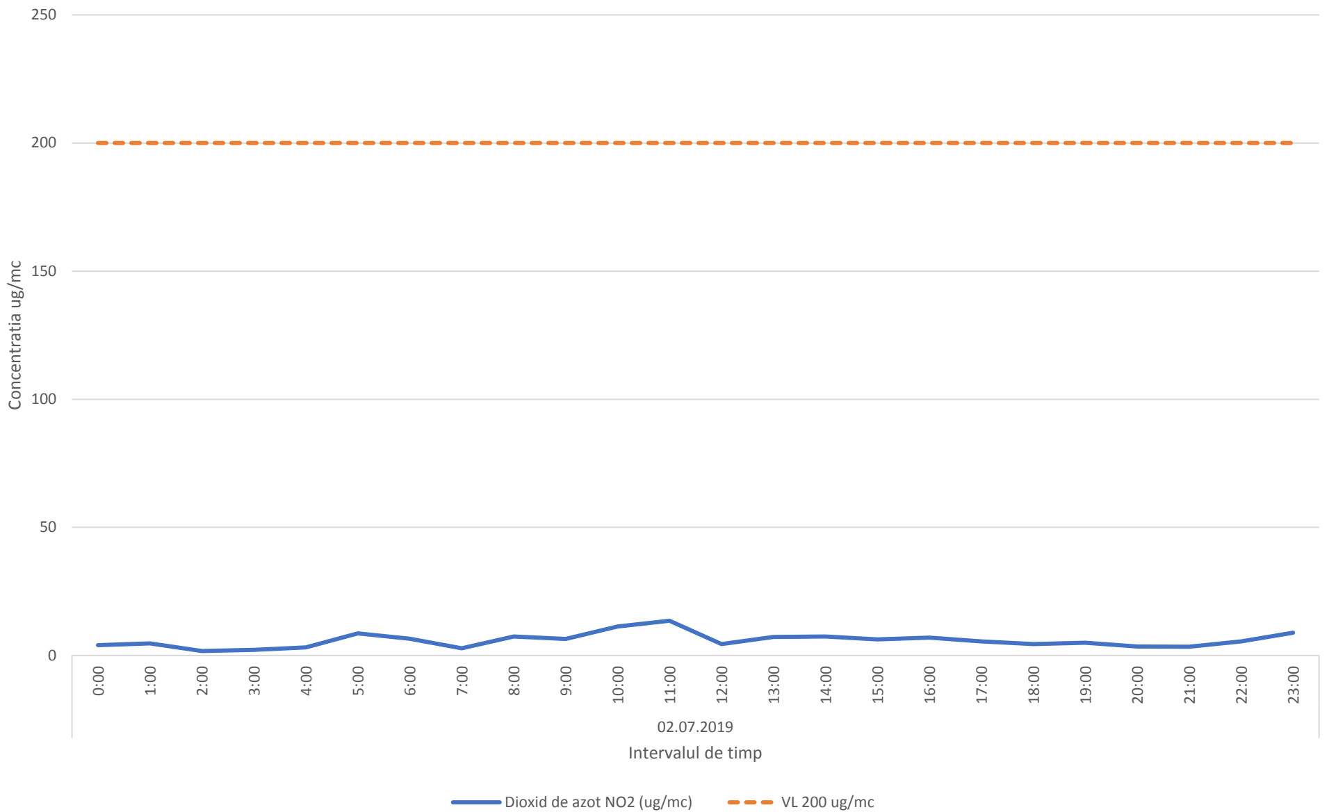
Variatia medilor orare ale indicatorului NO2 in data de 02.07.2019 - zona de nord-vest a platformei industriale Brazi
