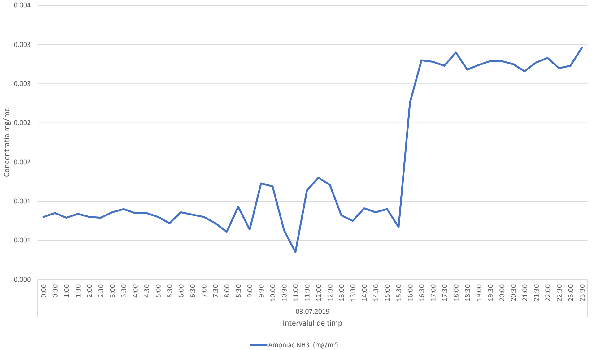
Variatia momentana (30 min.) a indicatorului NH3 in data de 03.07.2019 - zona de nord-vest a platformei industriale Brazi
