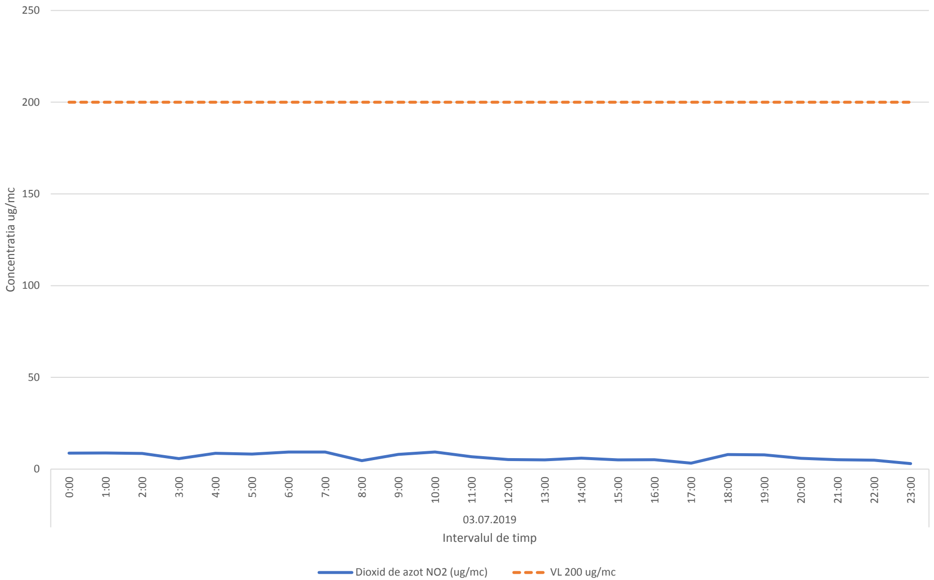
Variatia medilor orare ale indicatorului NO2 in data de 03.07.2019 - zona de nord-vest a platformei industriale Brazi
