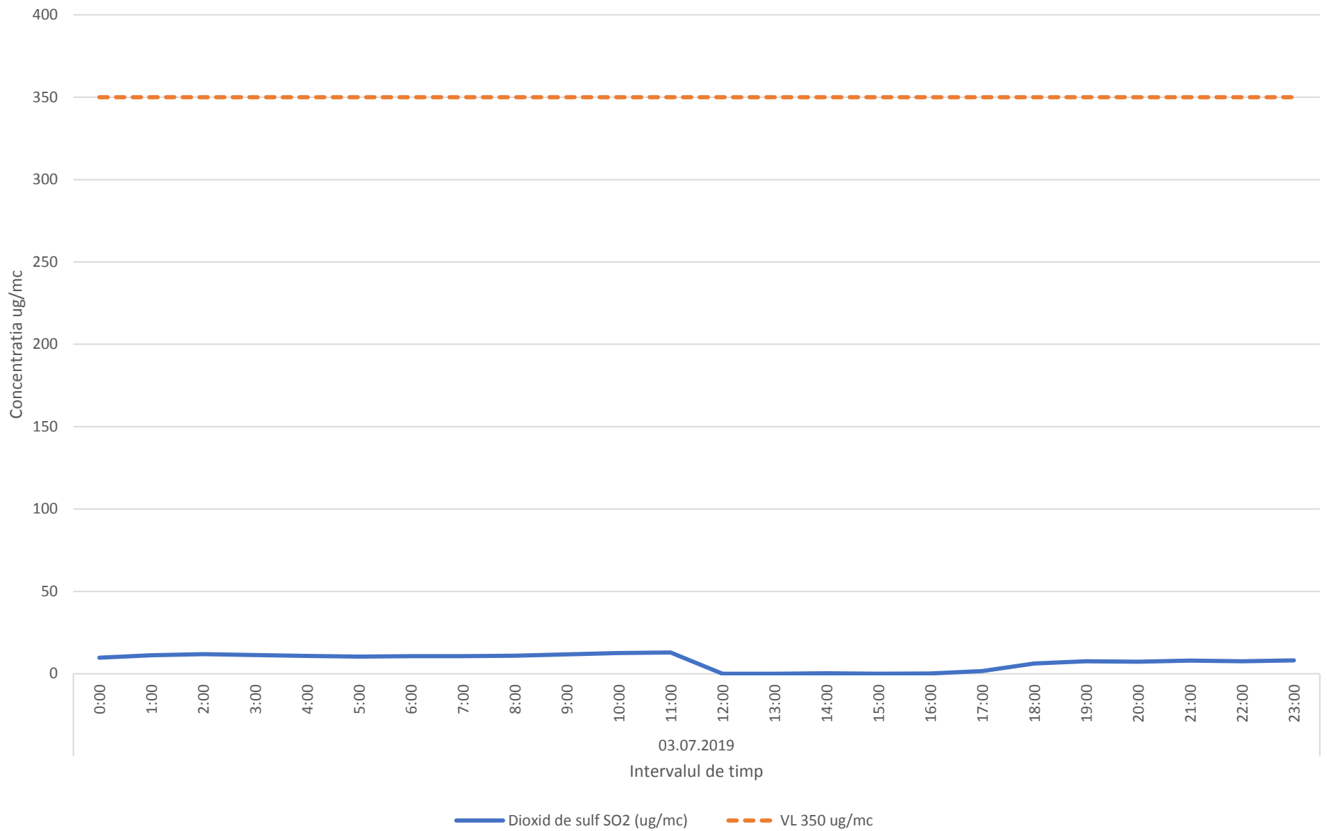
Variatia medilor orare ale indicatorului SO2 in data de 03.07.2019 - zona de nord-vest a platformei industriale Brazi
