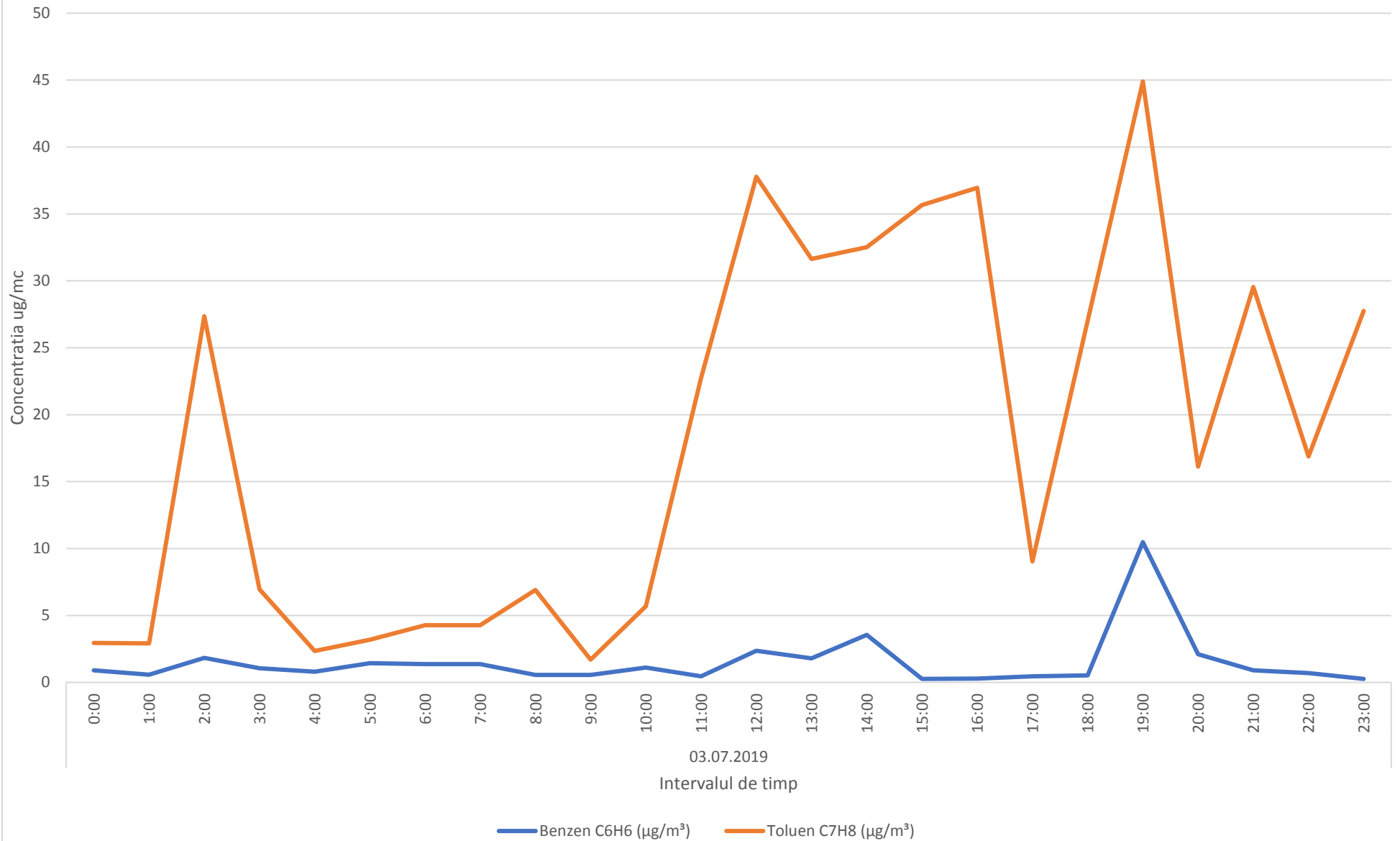
Variatia medilor orare a indicatorilor C6H6,C7H8 in data de 03.07.2019 - zona de nord-vest a platformei industriale Brazi
