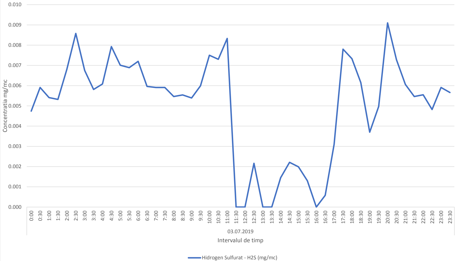
Variatia momentana (30 min.) a indicatorului H2S in data de 03.07.2019 - zona de nord-vest a platformei industriale Brazi
