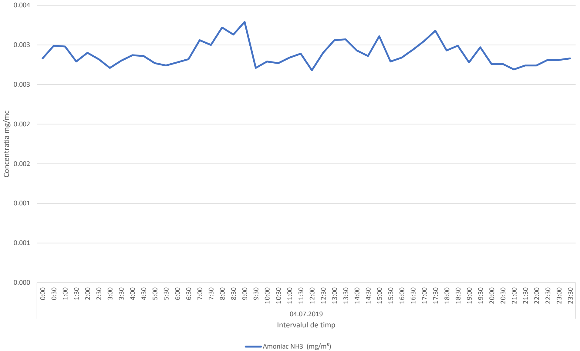
Variatia momentana (30 min.) a indicatorului NH3 in data de 04.07.2019 - zona de nord-vest a platformei industriale Brazi
