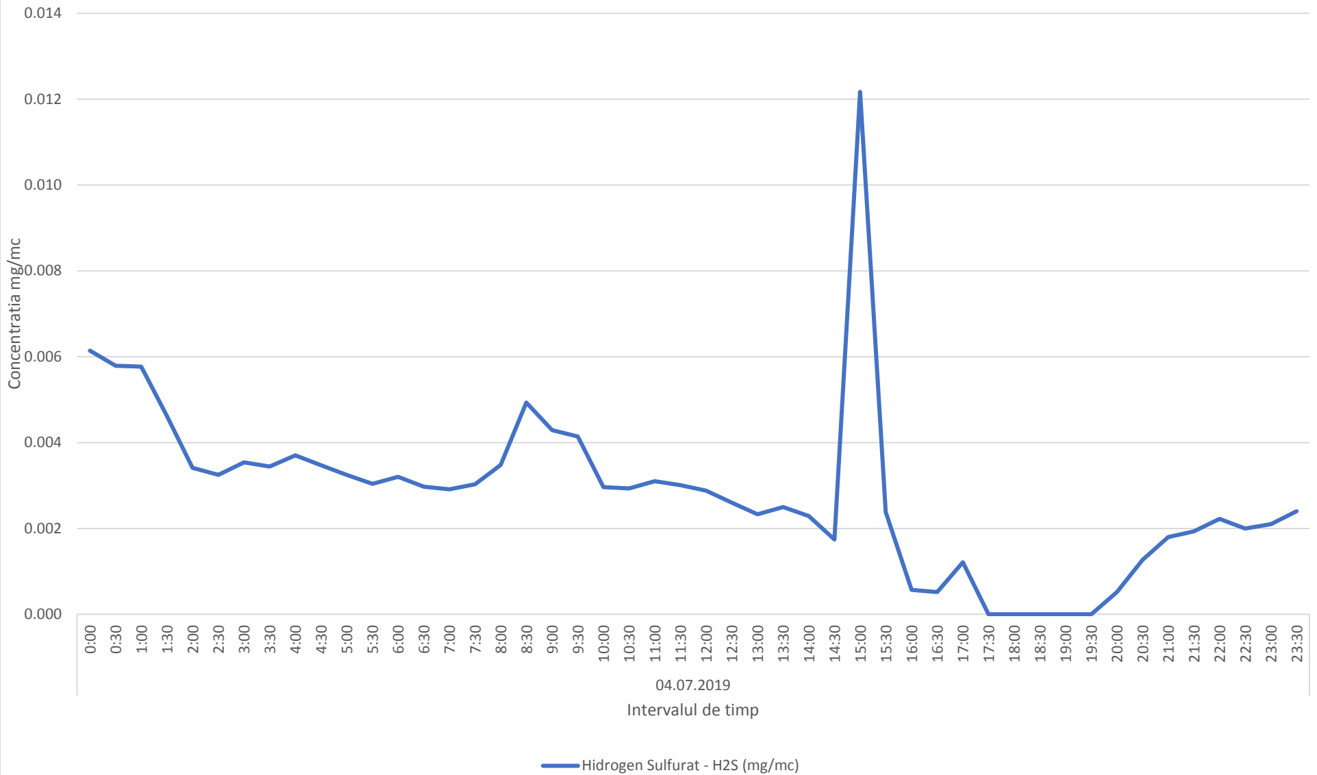
Variatia momentana (30 min.) a indicatorului H2S in data de 04.07.2019 - zona de nord-vest a platformei industriale Brazi
