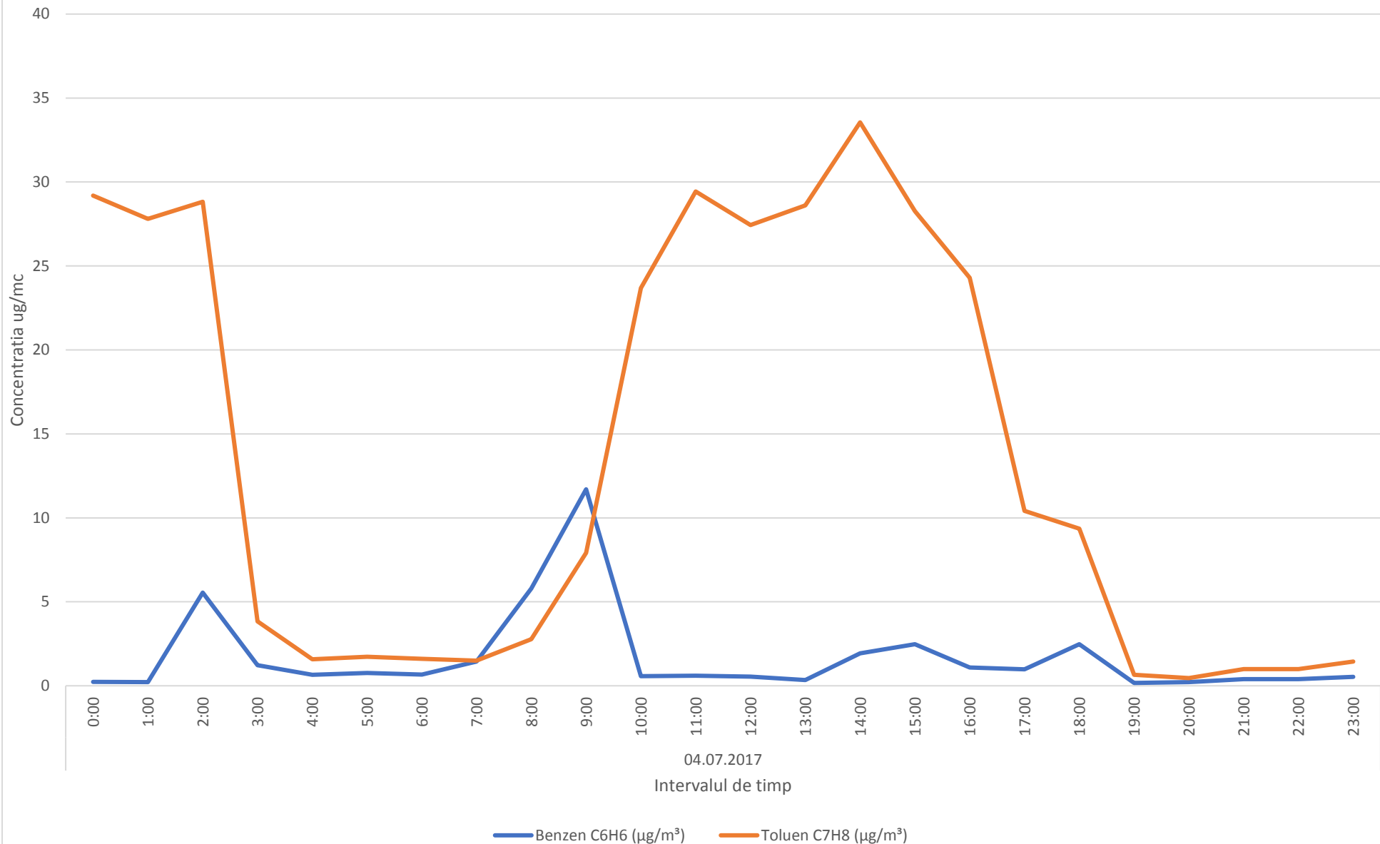
Variatia medilor orare a indicatorilor C6H6,C7H8 in data de 04.07.2019 - zona de nord-vest a platformei industriale Brazi
