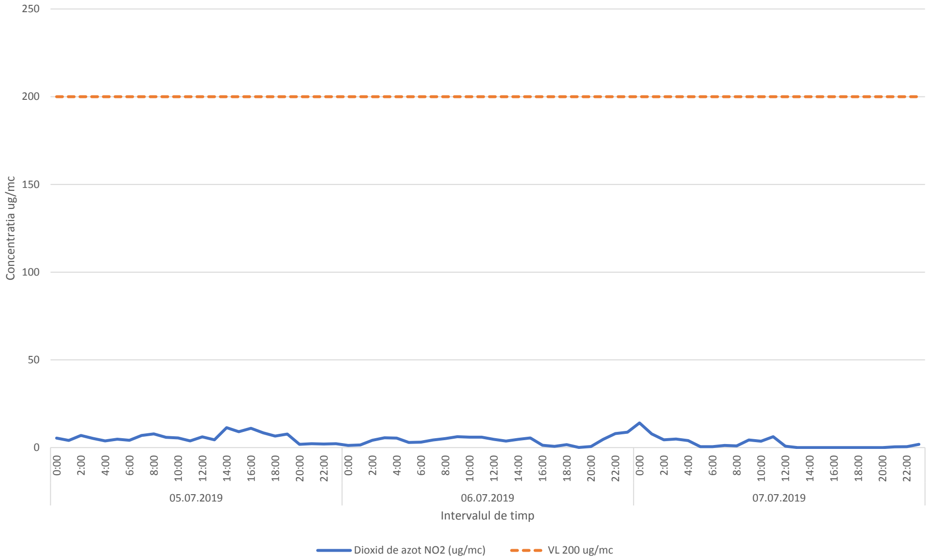
Variatia medilor orare ale indicatorului NO2 in perioada 05.07.2019-07.07.2019- zona de nord-vest a platformei industriale Brazi
