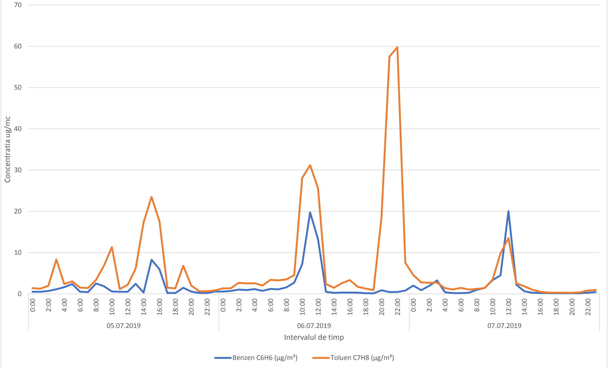
Variatia medilor orare a indicatorilor C6H6,C7H8 in perioada 05.07.2019-07.07.2019- zona de nord-vest a platformei industriale Brazi
