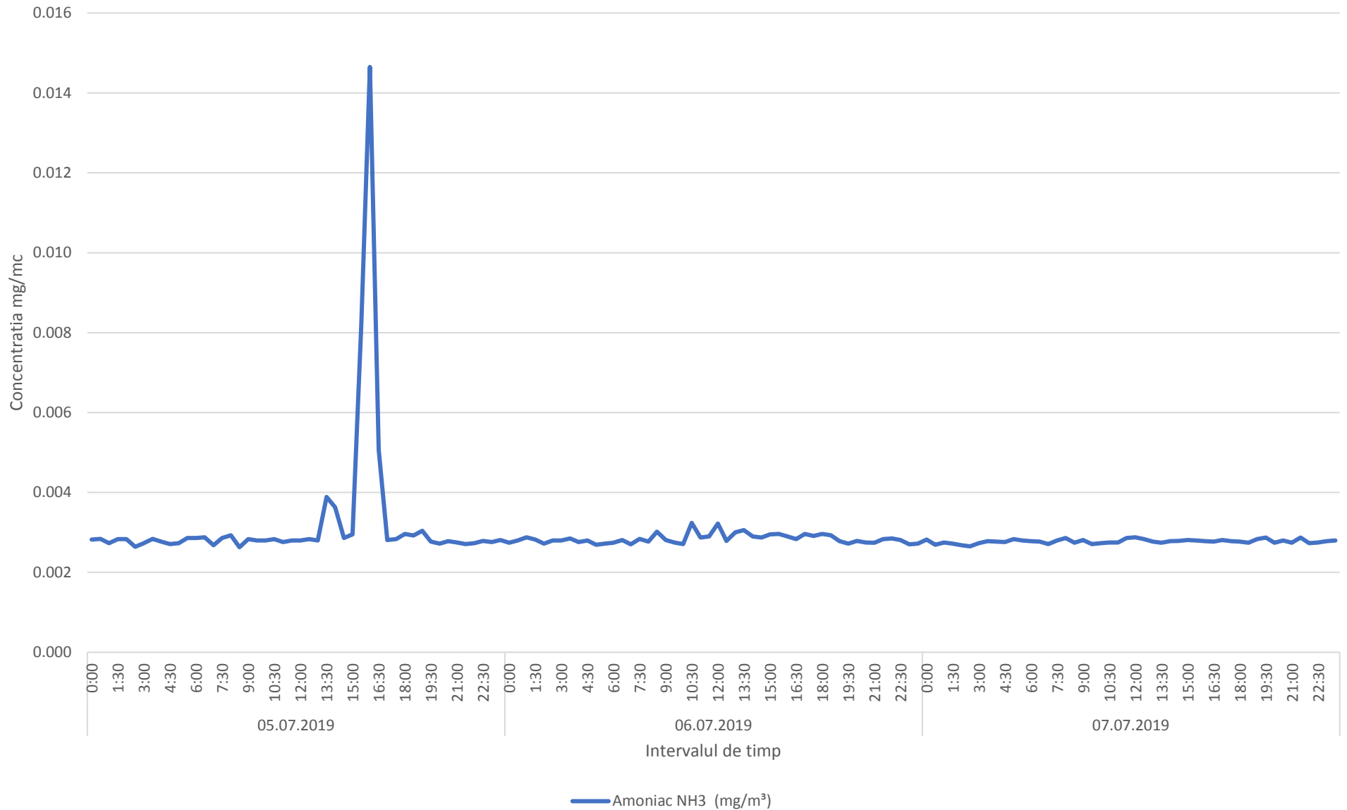
Variatia momentana (30 min.) a indicatorului NH3 in perioada 05.07.2019-07.07.2019- zona de nord-vest a platformei industriale Brazi
