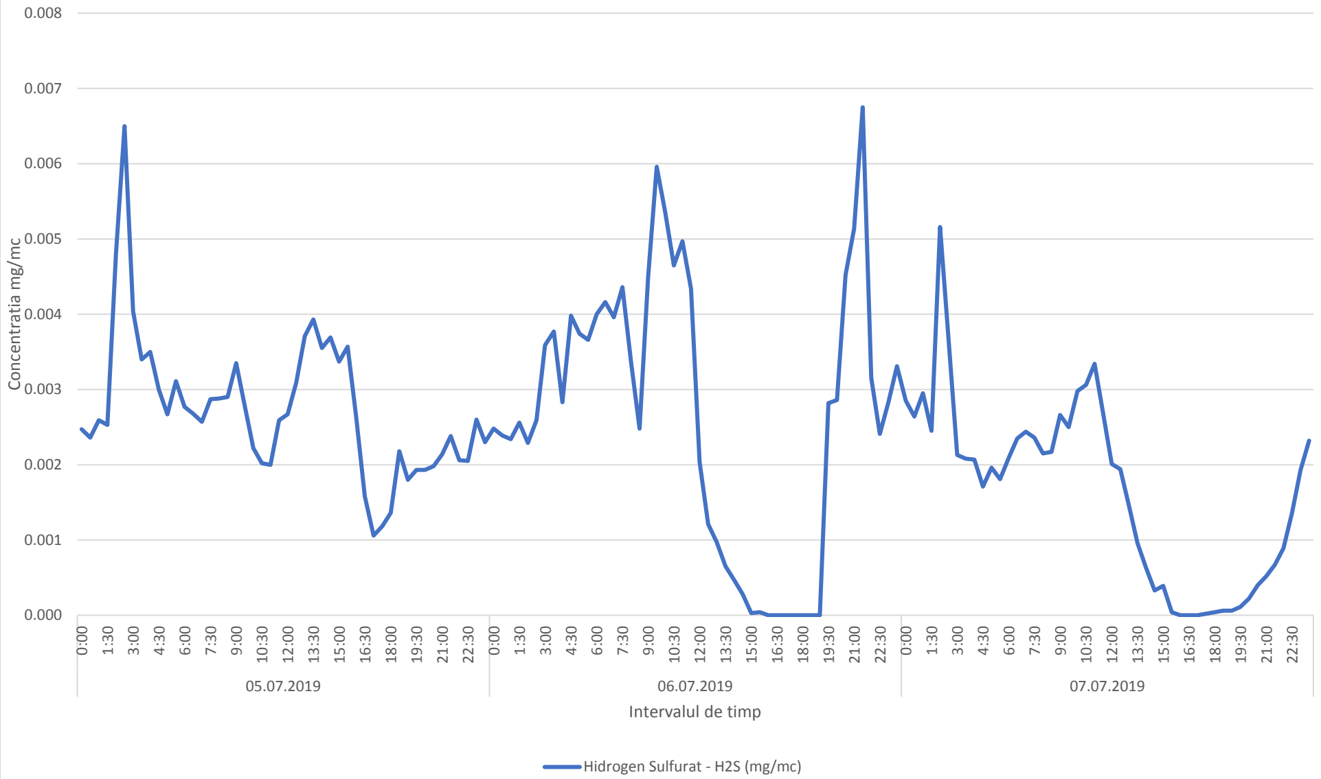
Variatia momentana (30 min.) a indicatorului H2S in perioada 05.07.2019-07.07.2019- zona de nord-vest a platformei industriale Brazi
