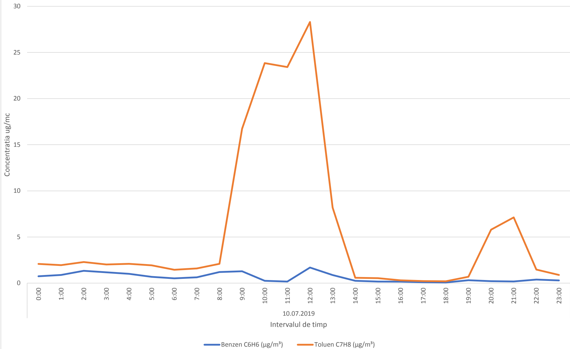
Variatia medilor orare a indicatorilor C6H6,C7H8 in data de 10.07.2019- zona de nord-vest a platformei industriale Brazi
