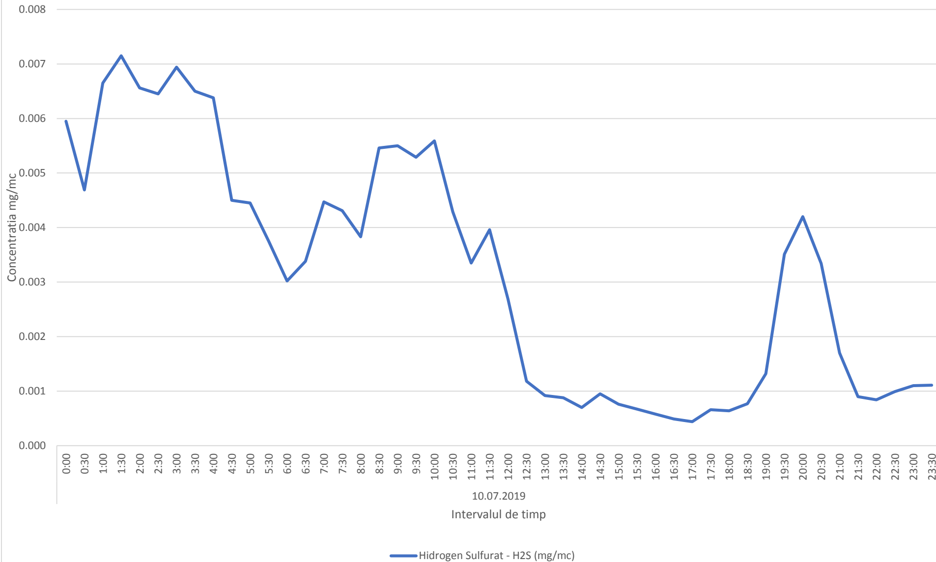
Variatia momentana (30 min.) a indicatorului H2S in data de 10.07.2019- zona de nord-vest a platformei industriale Brazi
