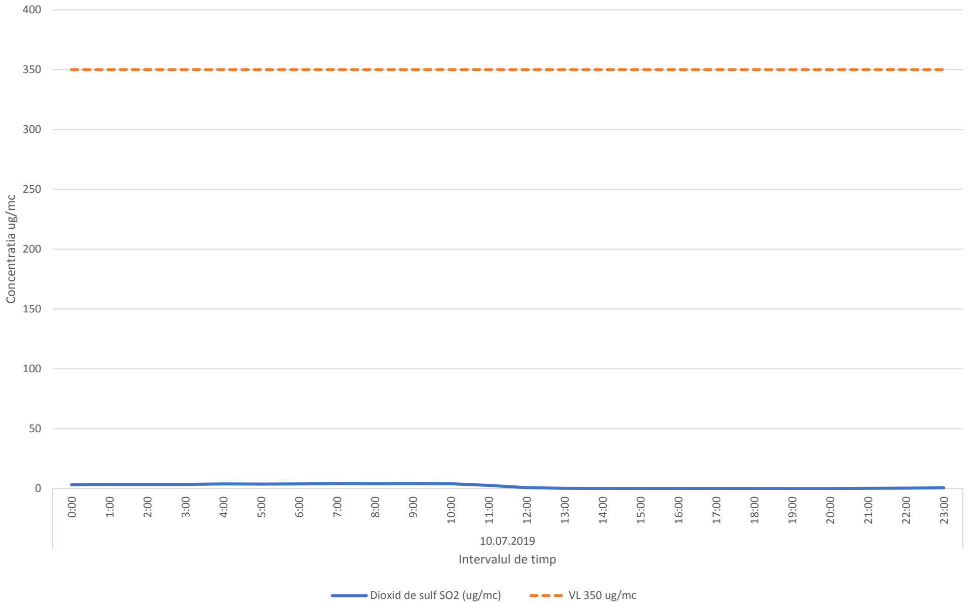
Variatia medilor orare ale indicatorului SO2 in data de 10.07.2019- zona de nord-vest a platformei industriale Brazi
