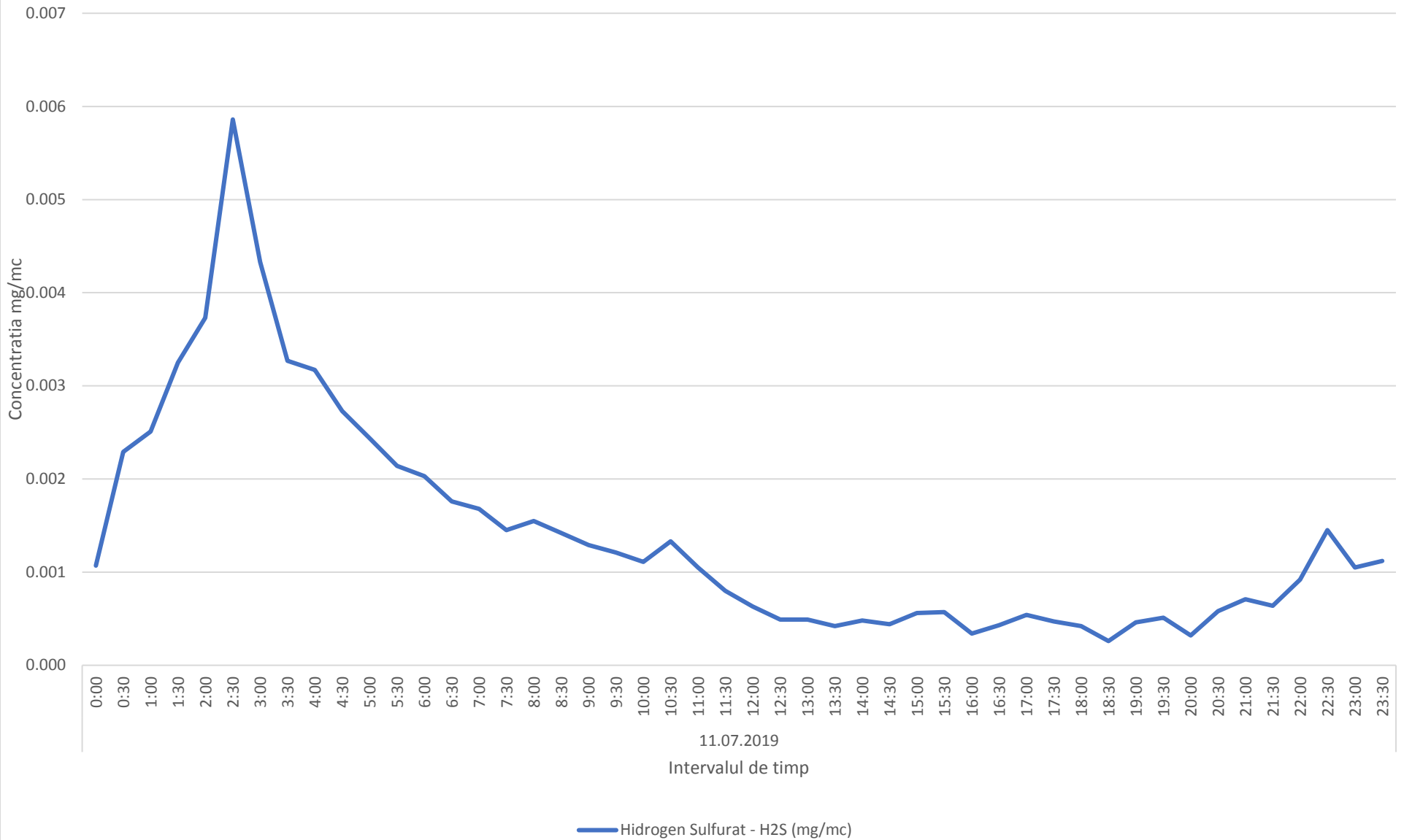
Variatia momentana (30 min.) a indicatorului H2S in data de 11.07.2019- zona de nord-vest a platformei industriale Brazi
