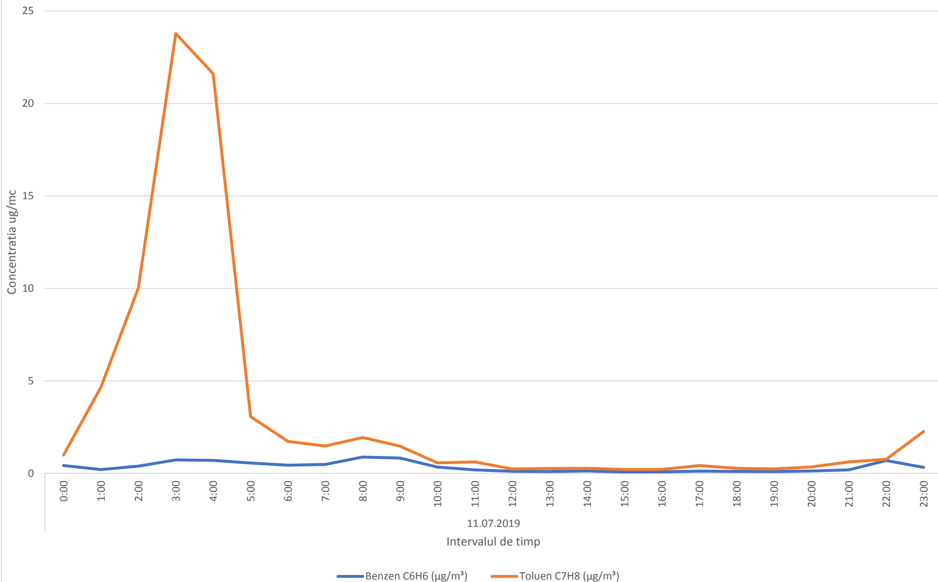
Variatia medilor orare a indicatorilor C6H6,C7H8 in data de 11.07.2019- zona de nord-vest a platformei industriale Brazi
