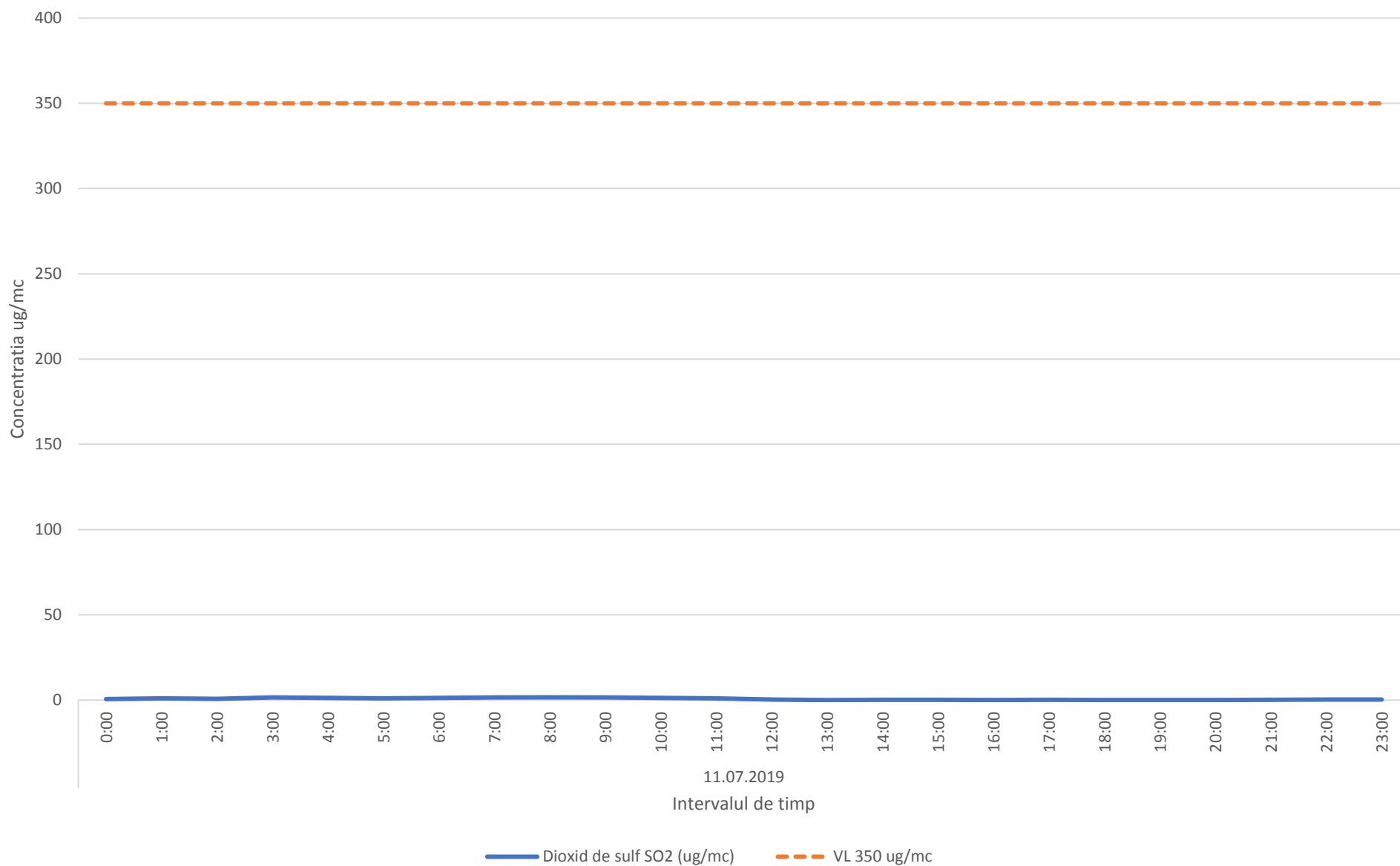
Variatia medilor orare ale indicatorului SO2 in data de 11.07.2019- zona de nord-vest a platformei industriale Brazi
