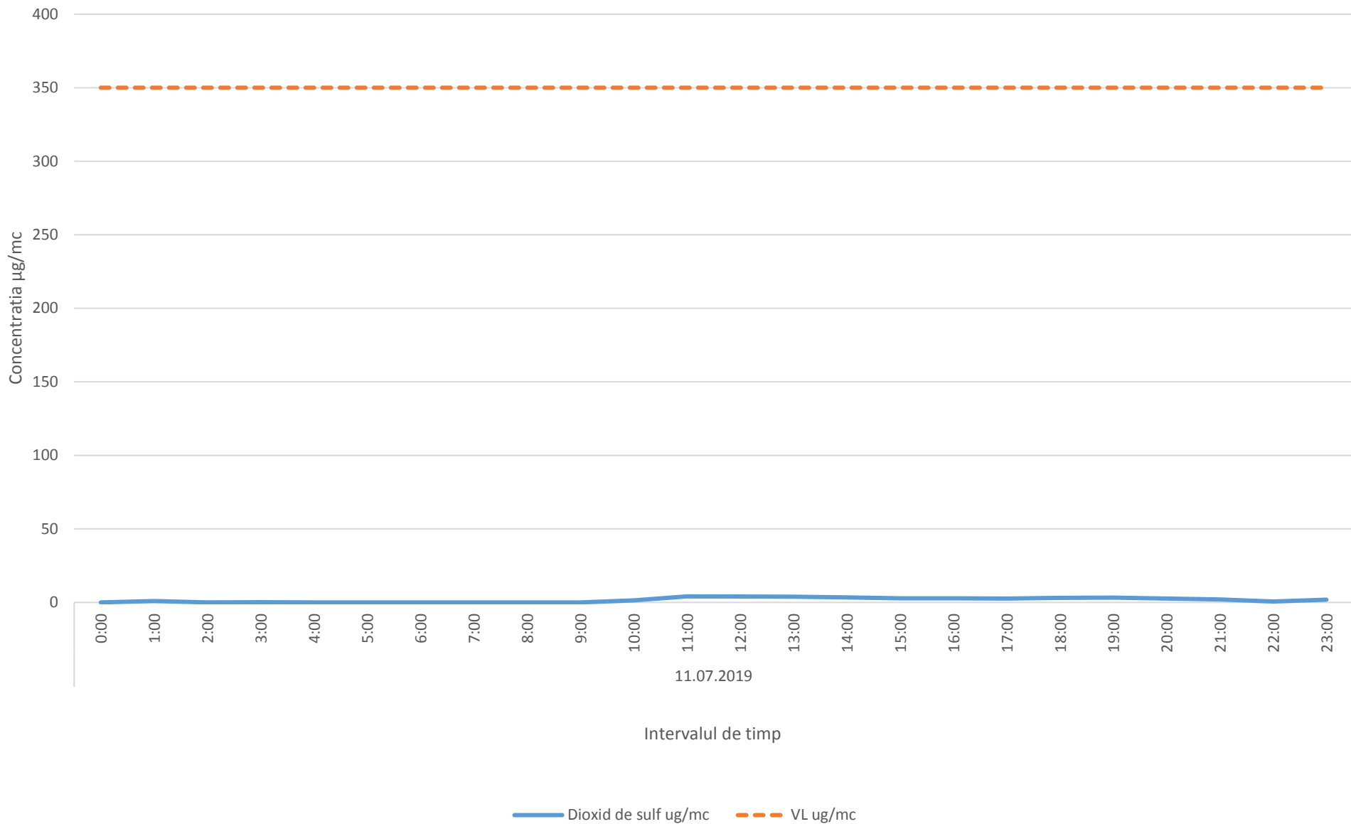
Variatia orara a indicatorului SO2 in data de 11.07.2019 - zona de nora a platformei industriale Brazi
