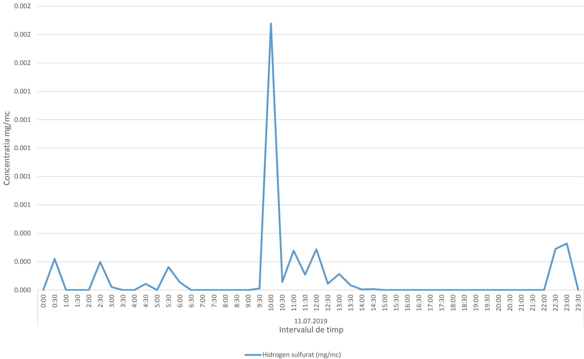
Variatia momentana (30 min.) a indicatorului H2S in data de 11.07.2019 - zona de nora a platformei industriale Brazi
