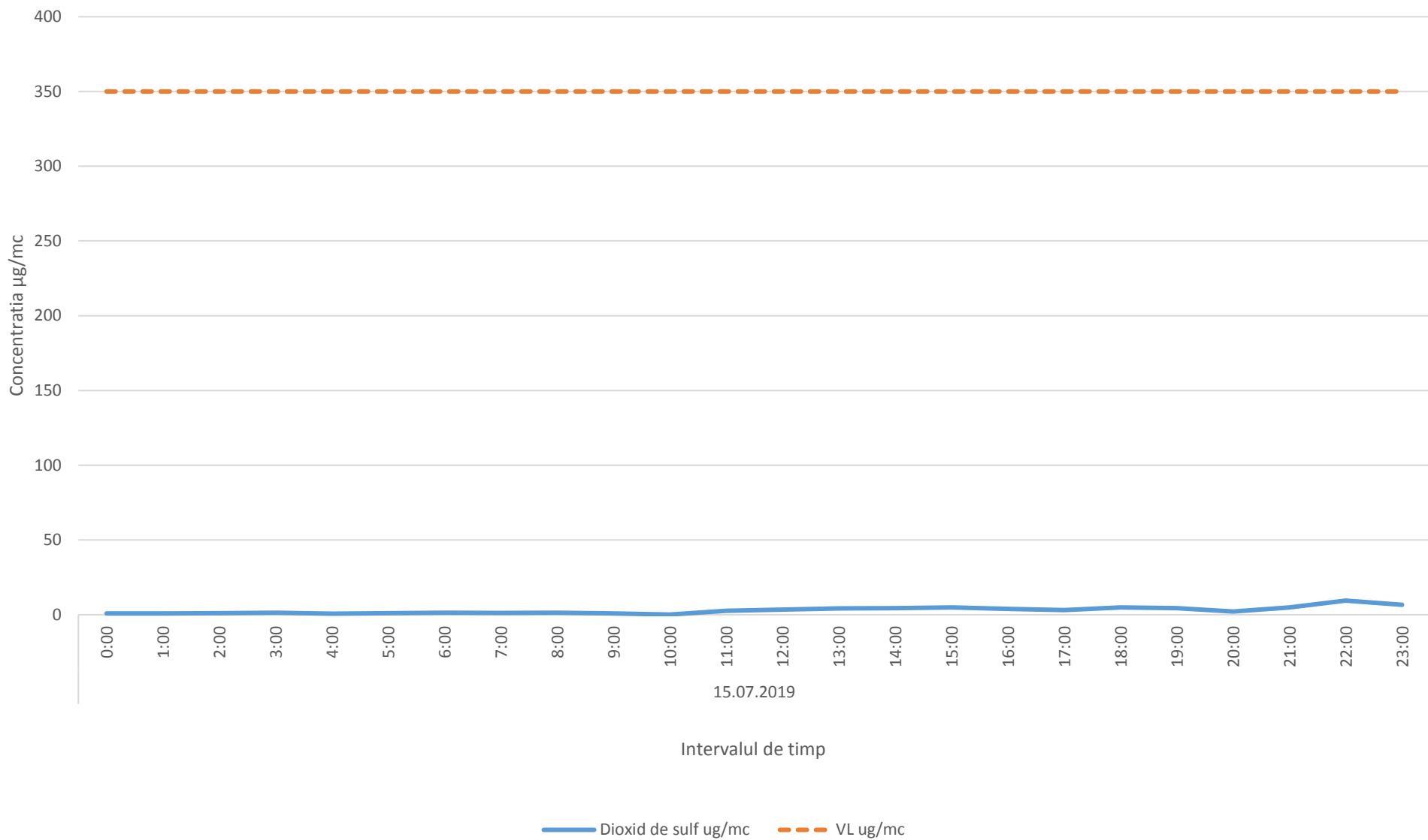
Variatia orara a indicatorului SO2 in data de 15.07.2019- zona de nora a platformei industriale Brazi
