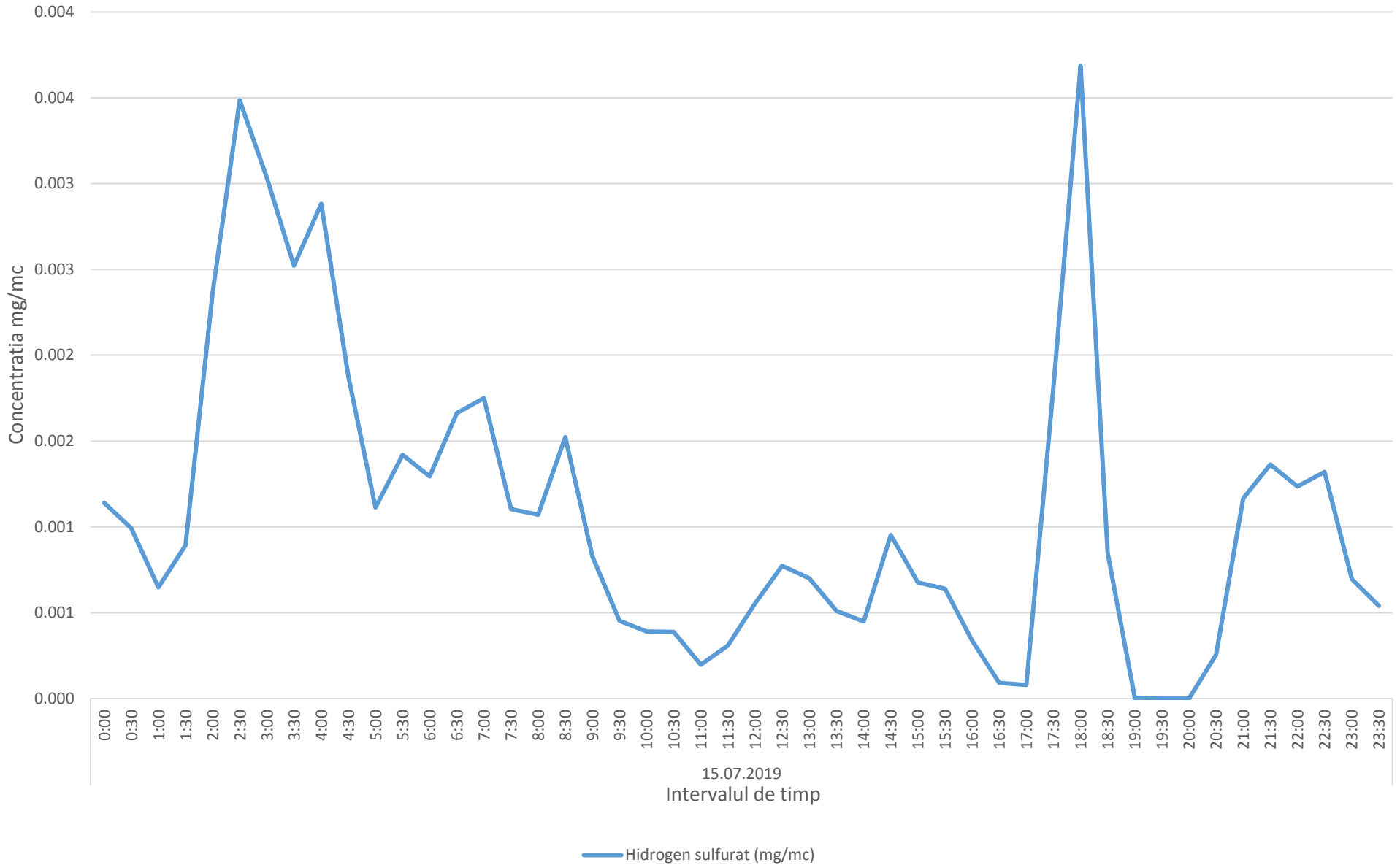
Variatia momentana (30 min.) a indicatorului H2S in data de 15.07.2019- zona de nora a platformei industriale Brazi
