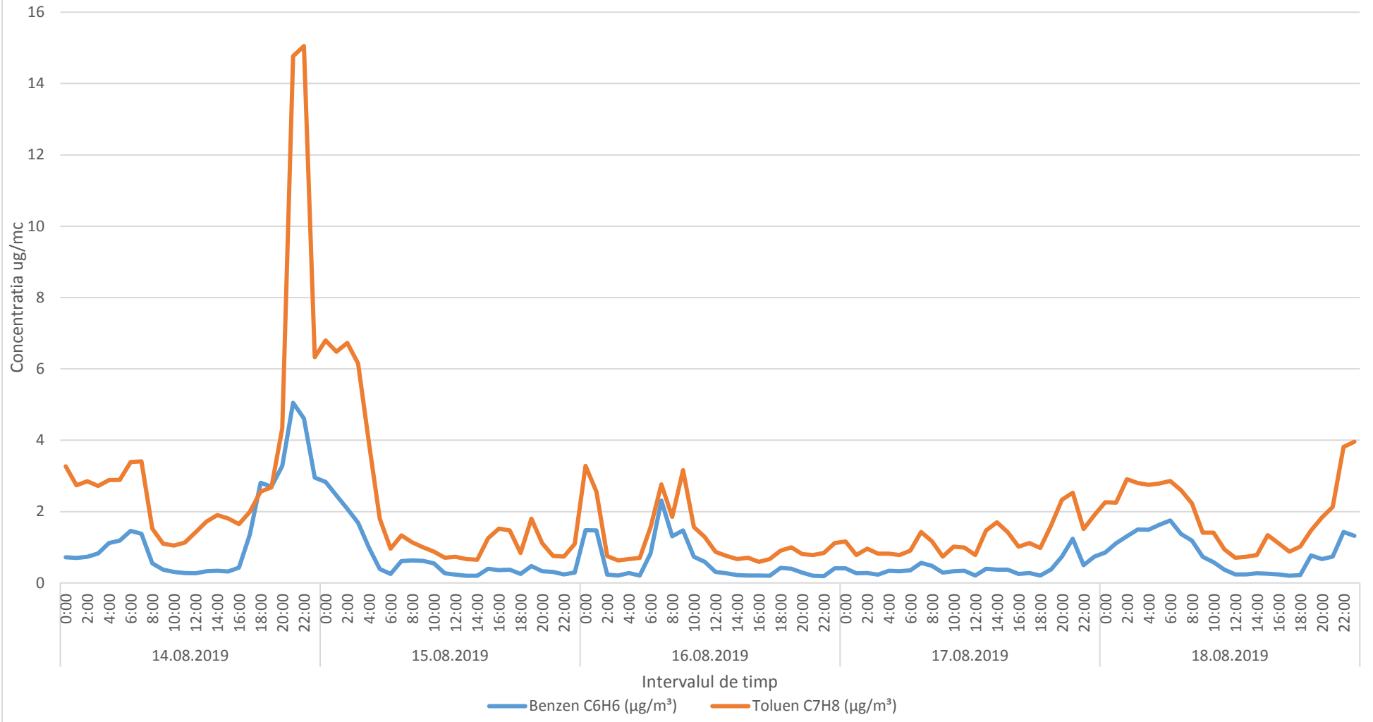
Variatia mediilor orare a indicatorilor C6H6,C7H8 in perioada 14.08.2019 - 18.08.2019- zona Oras Ploeni
