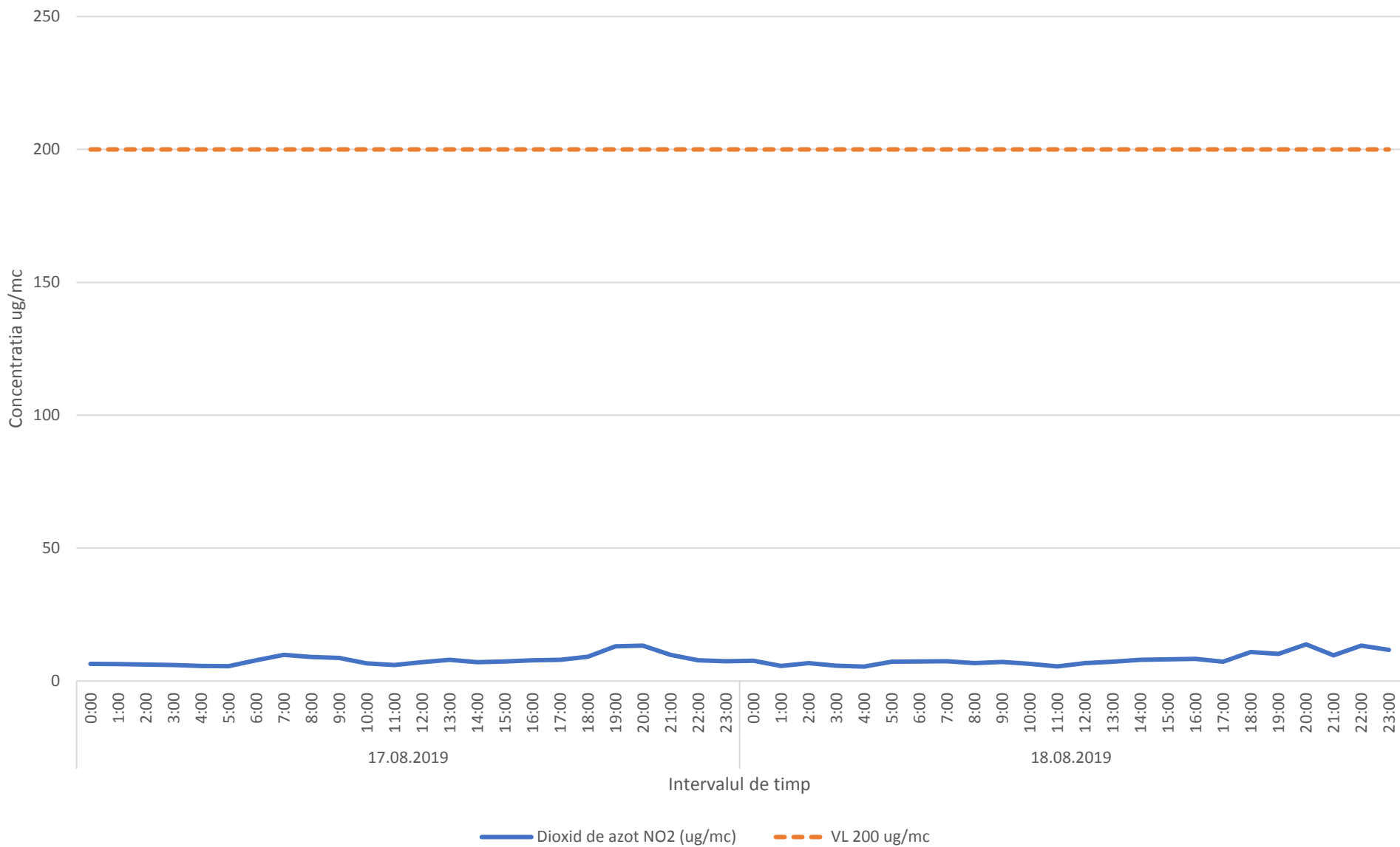
Variatia mediilor orare ale indicatorului NO2 in perioada 14.08.2019-18.08.2019- zona Oras Plopeni
