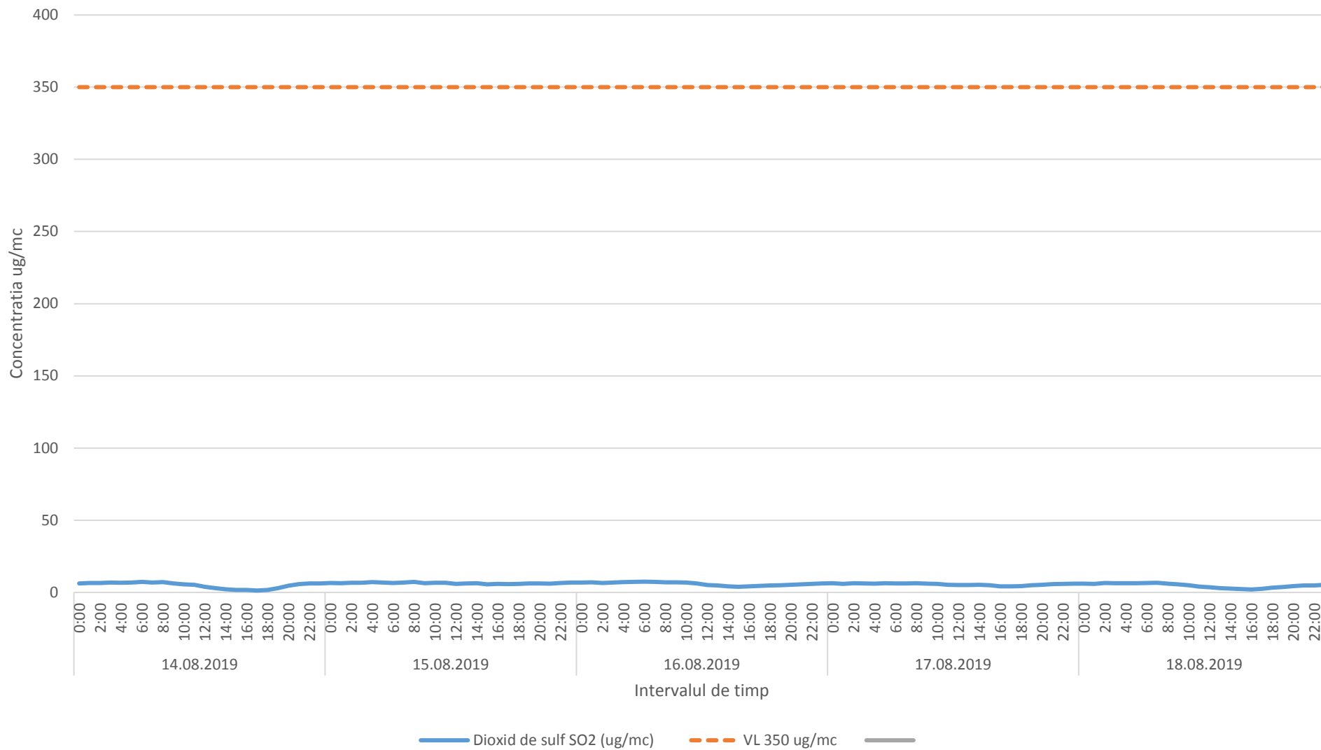
Variatia mediilor orare ale indicatorului SO2 in perioada 14.08.2019 - 18.08.2019 - zona Oras Plopeni
