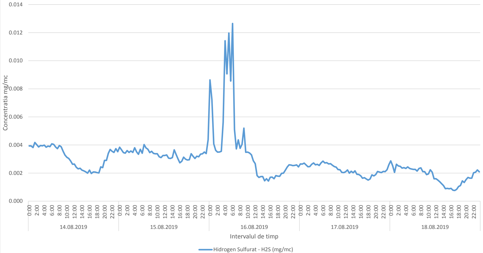
Variatia momentana (30 min.) a indicatorului H2S in perioada 14.08.2019 - 18.08.2019 - zona Oras Plopeni
