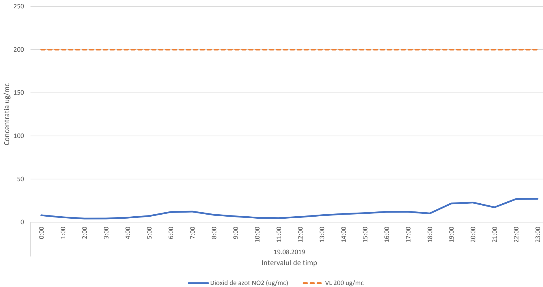
Variatia mediilor orare ale indicatorului NO2 in data de 19.08.2019- zona Oras Plopeni
