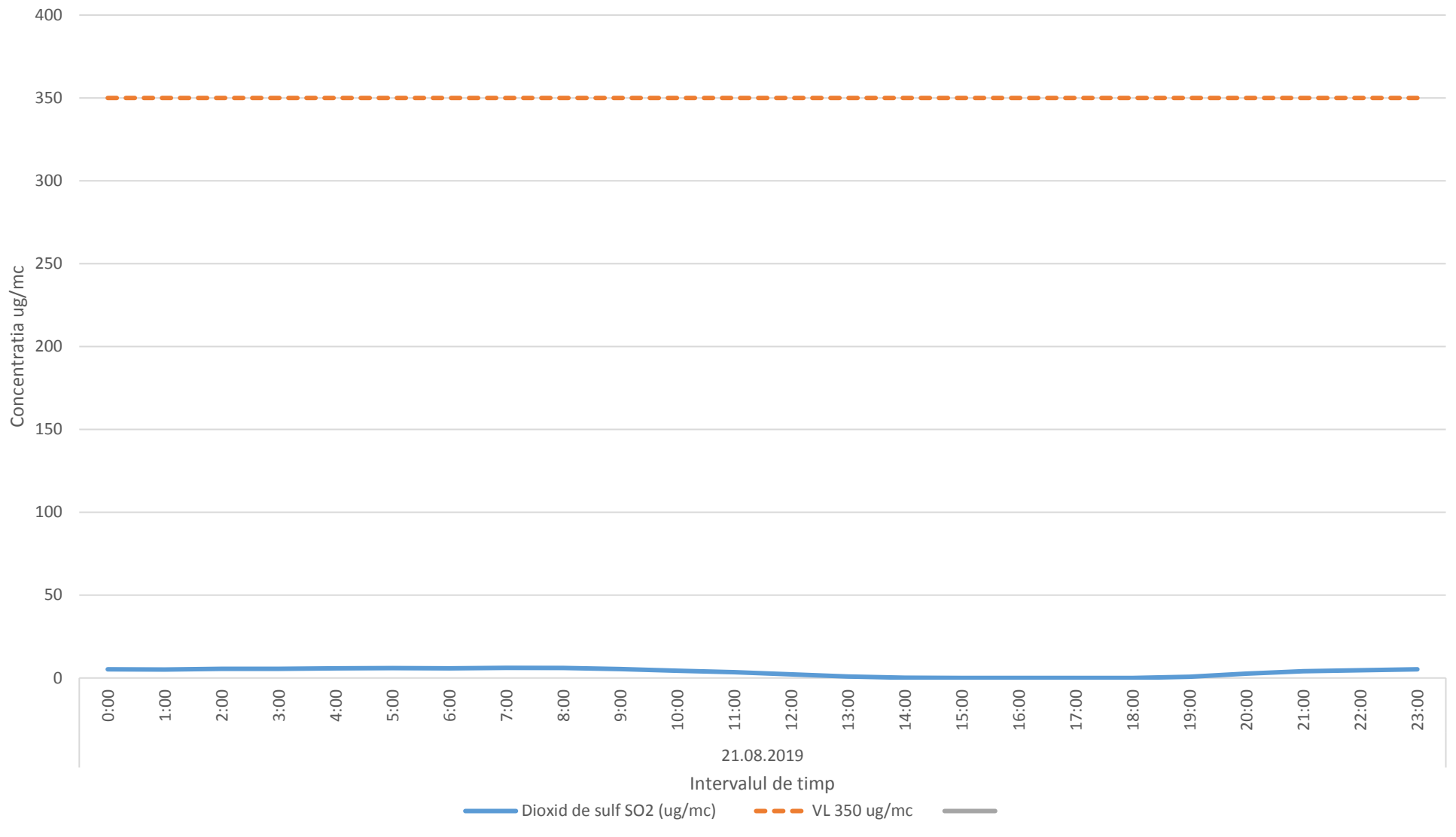
Variatia mediilor orare ale indicatorului SO2 in data de 21.08.2019 - zona Oras Plopeni
