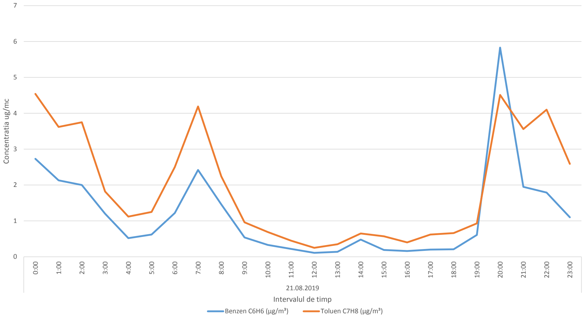
Variatia mediilor orare a indicatorilor C6H6,C7H8 in data de 21.08.2019 - zona Oras Plopeni
