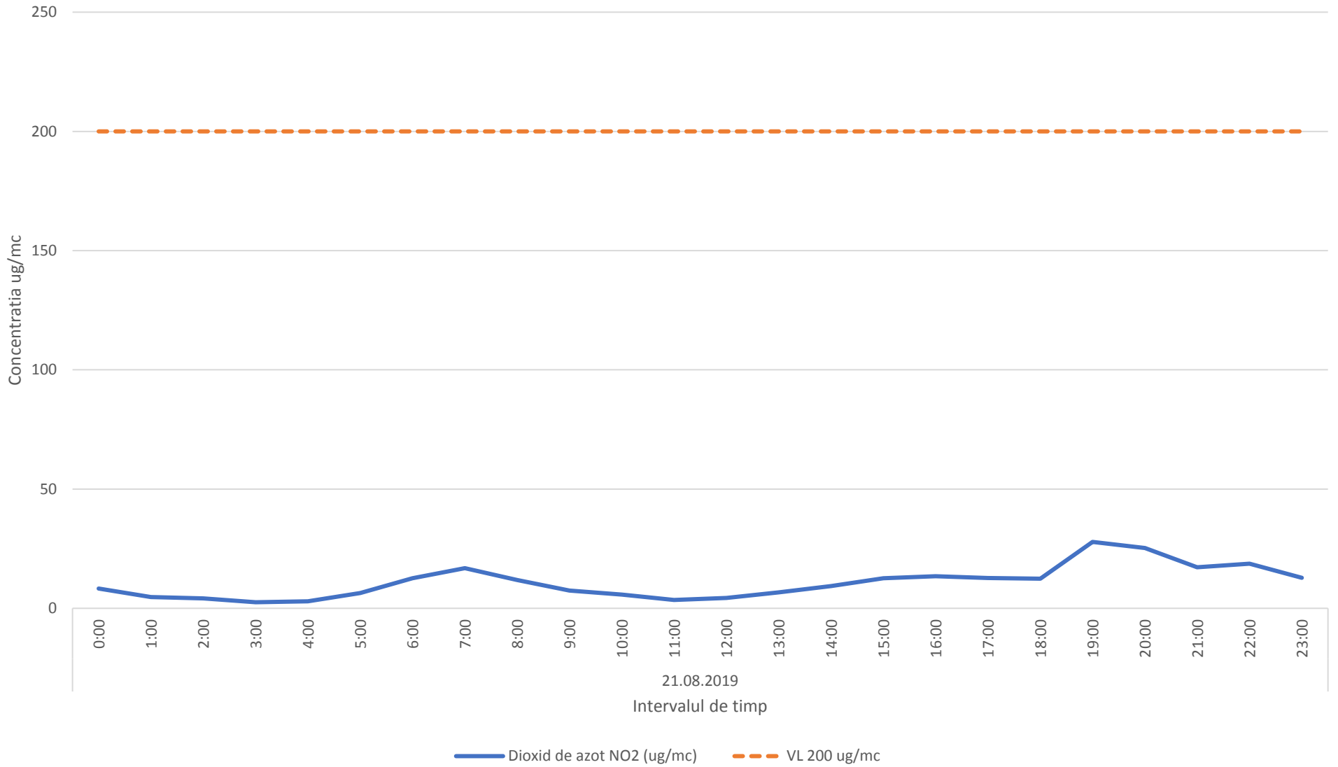
Variatia mediilor orare ale indicatorului NO2 in data de 21.08.2019- zona Oras Plopeni
