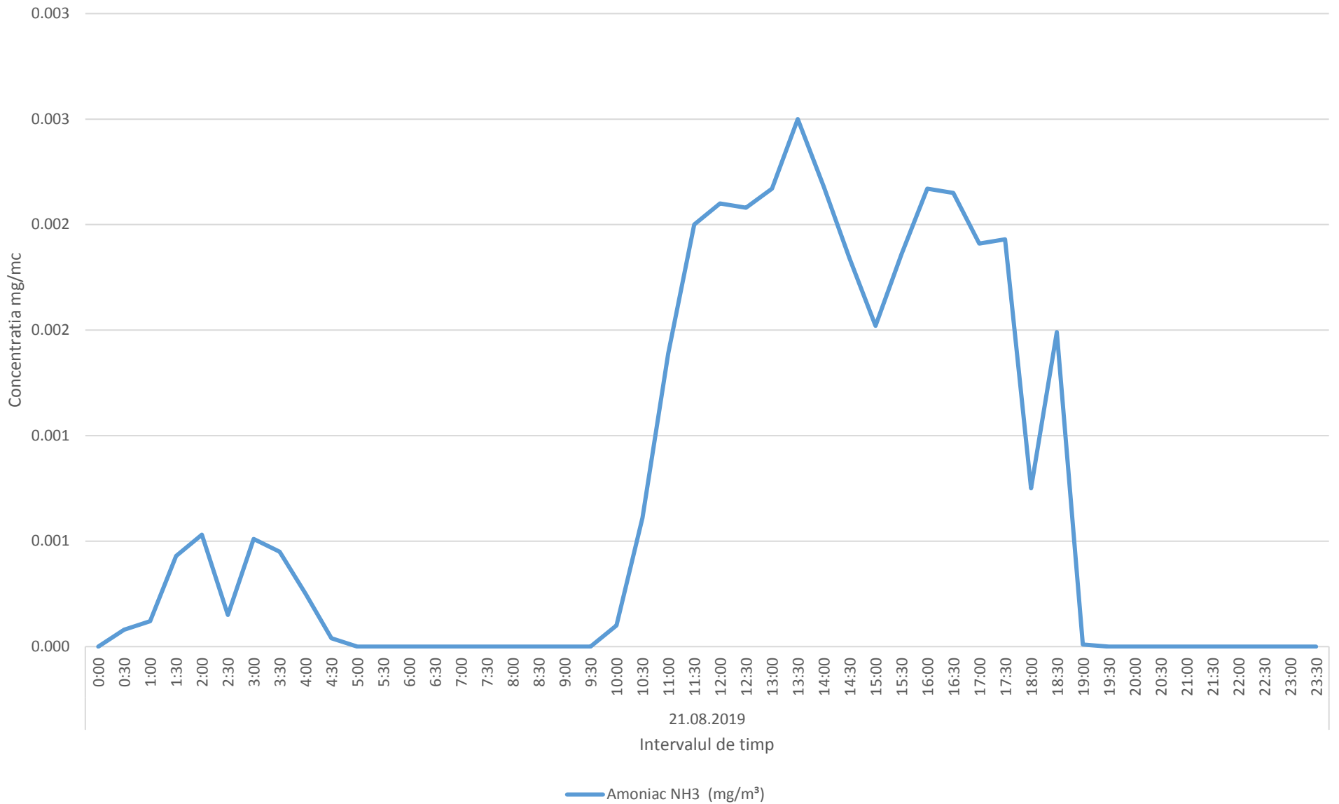
Variatia momentana (30 min.) a indicatorului NH3 in data de 21.08.2019 - zona Oras Plopeni
