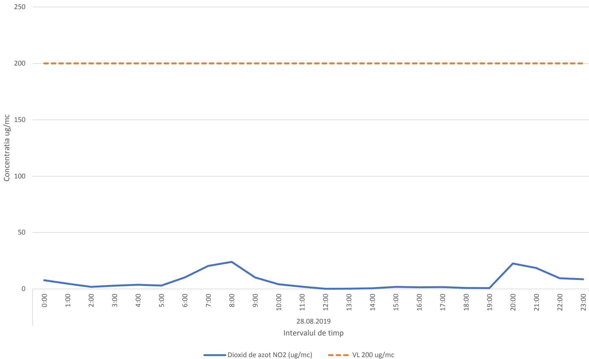
Variatia mediilor orare ale indicatorului NO2 in data de 28.08.2019 - zona Oras Plopeni
