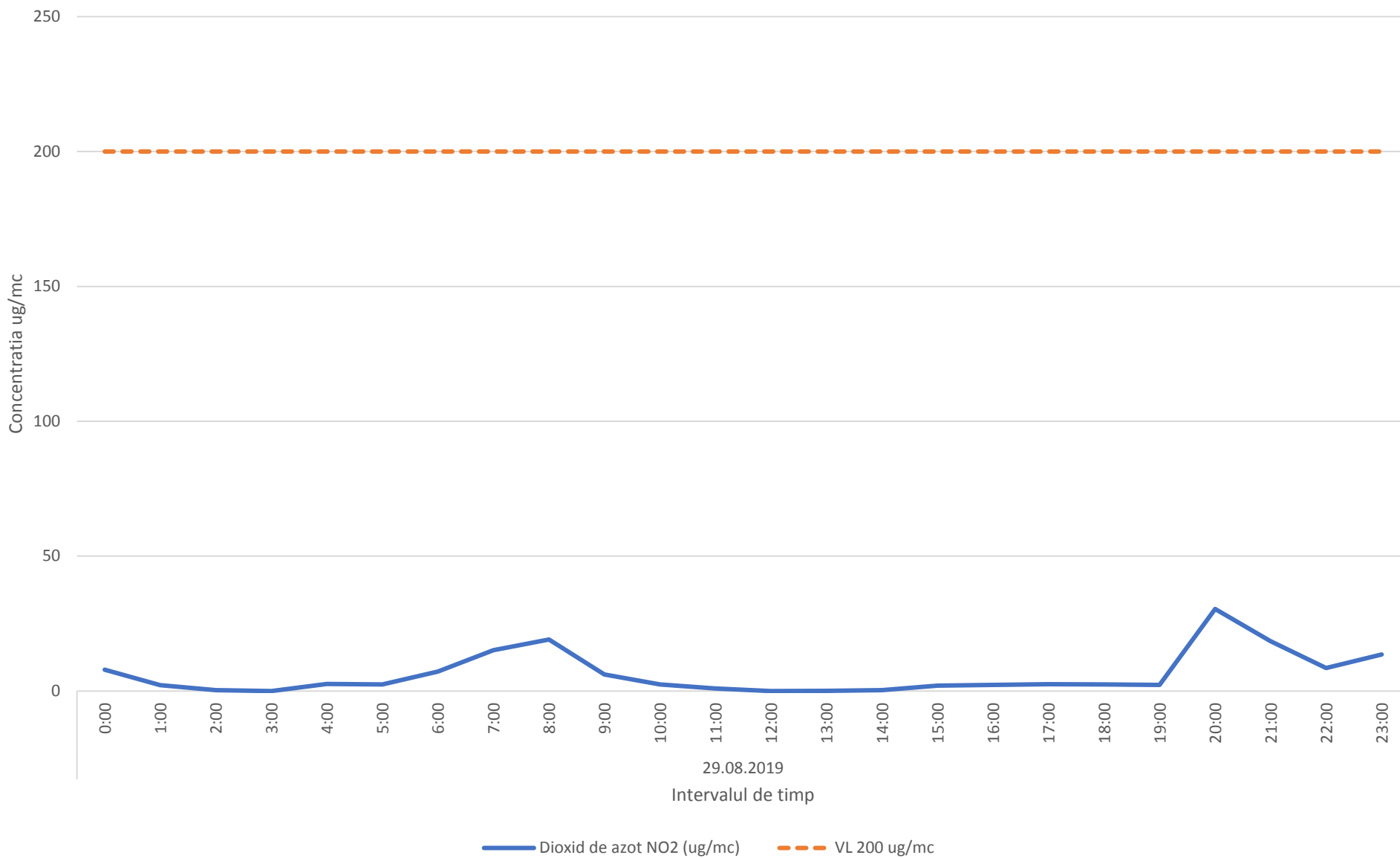
Variatia mediilor orare ale indicatorului NO2 in data de 29.08.2019 - zona Oras Plopeni
