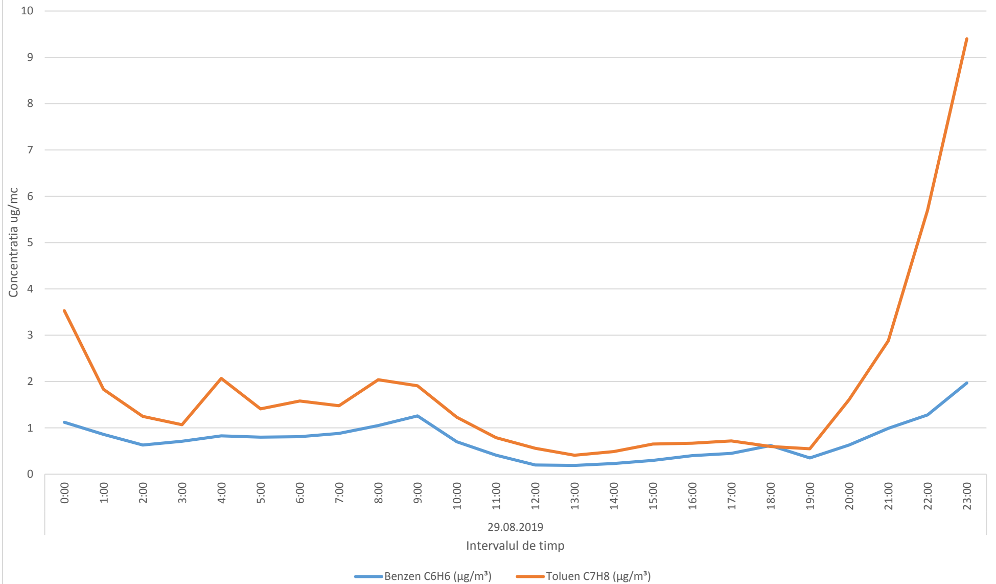
Variatia mediilor orare a indicatorilor C6H6,C7H8 in data de 29.08.2019 - zona Oras Plopeni
