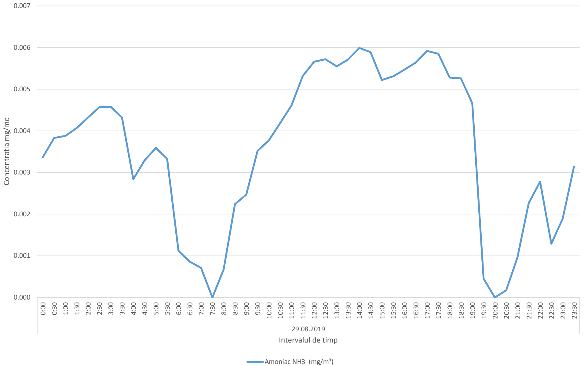
Variatia momentana (30 min.) a indicatorului NH3 in data de 29.08.2019 - zona Oras Plopeni
