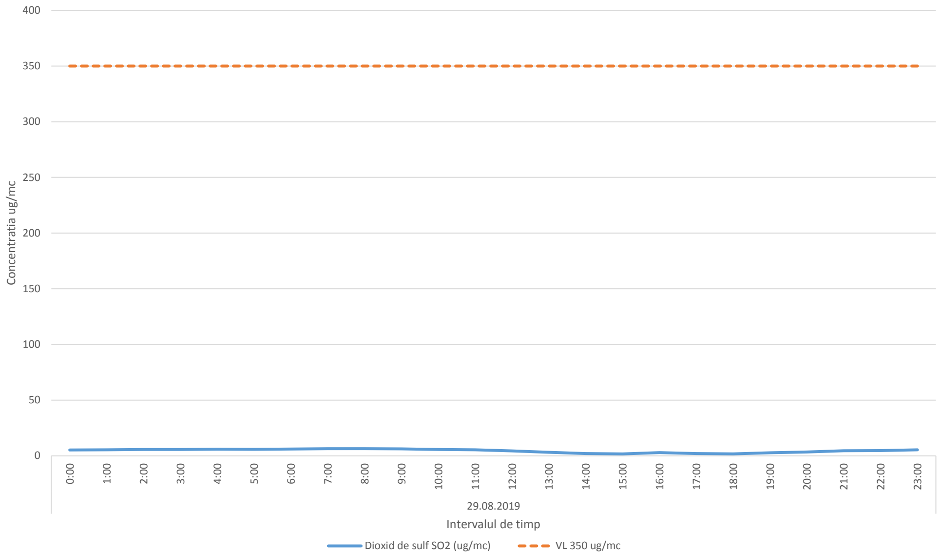
Variatia mediilor orare ale indicatorului SO2 in data de 29.08.2019 - zona Oras Plopeni
