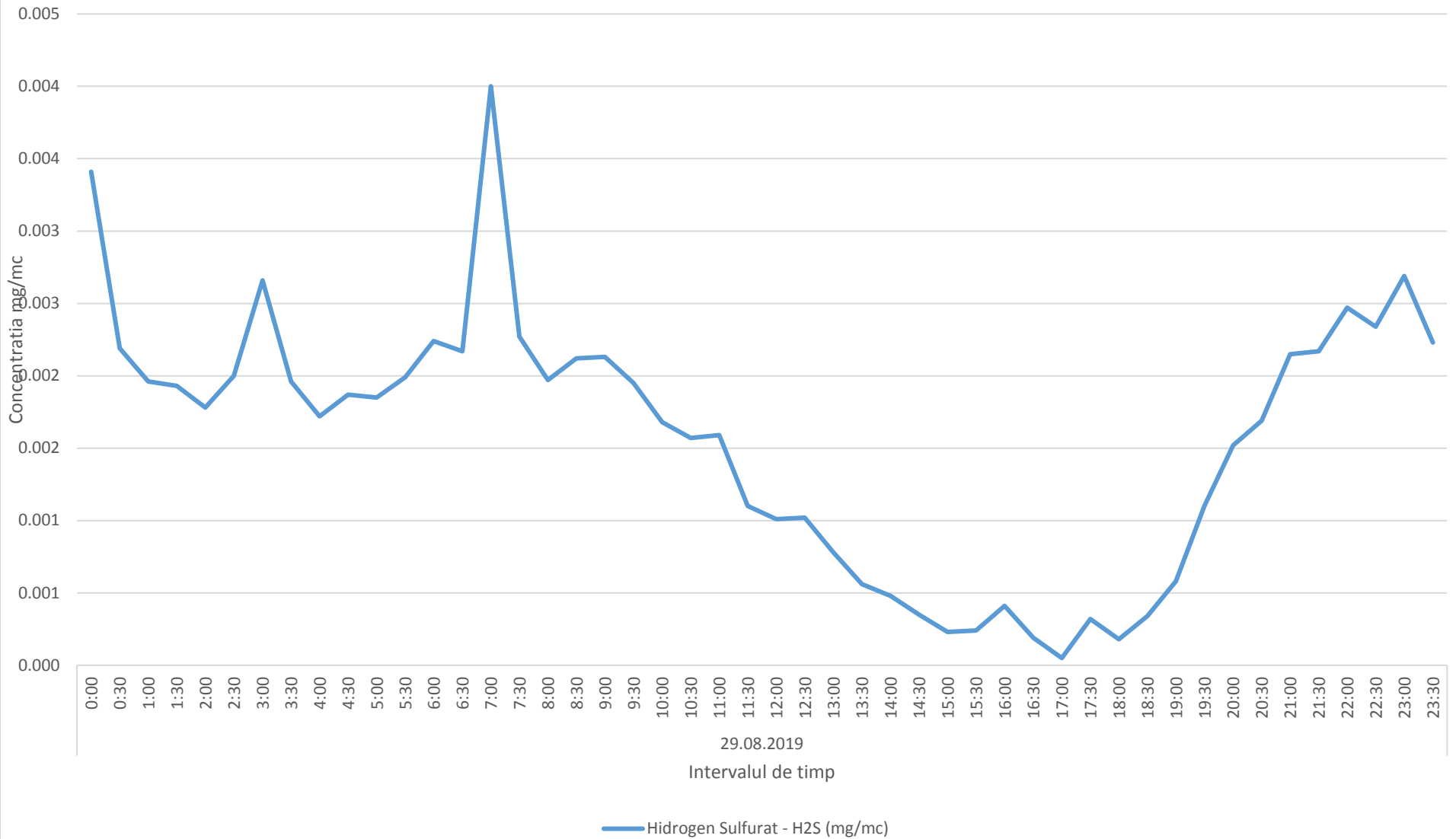
Variatia momentana (30 min.) a indicatorului H2S in data de 29.08.2019 - zona Oras Plopeni
