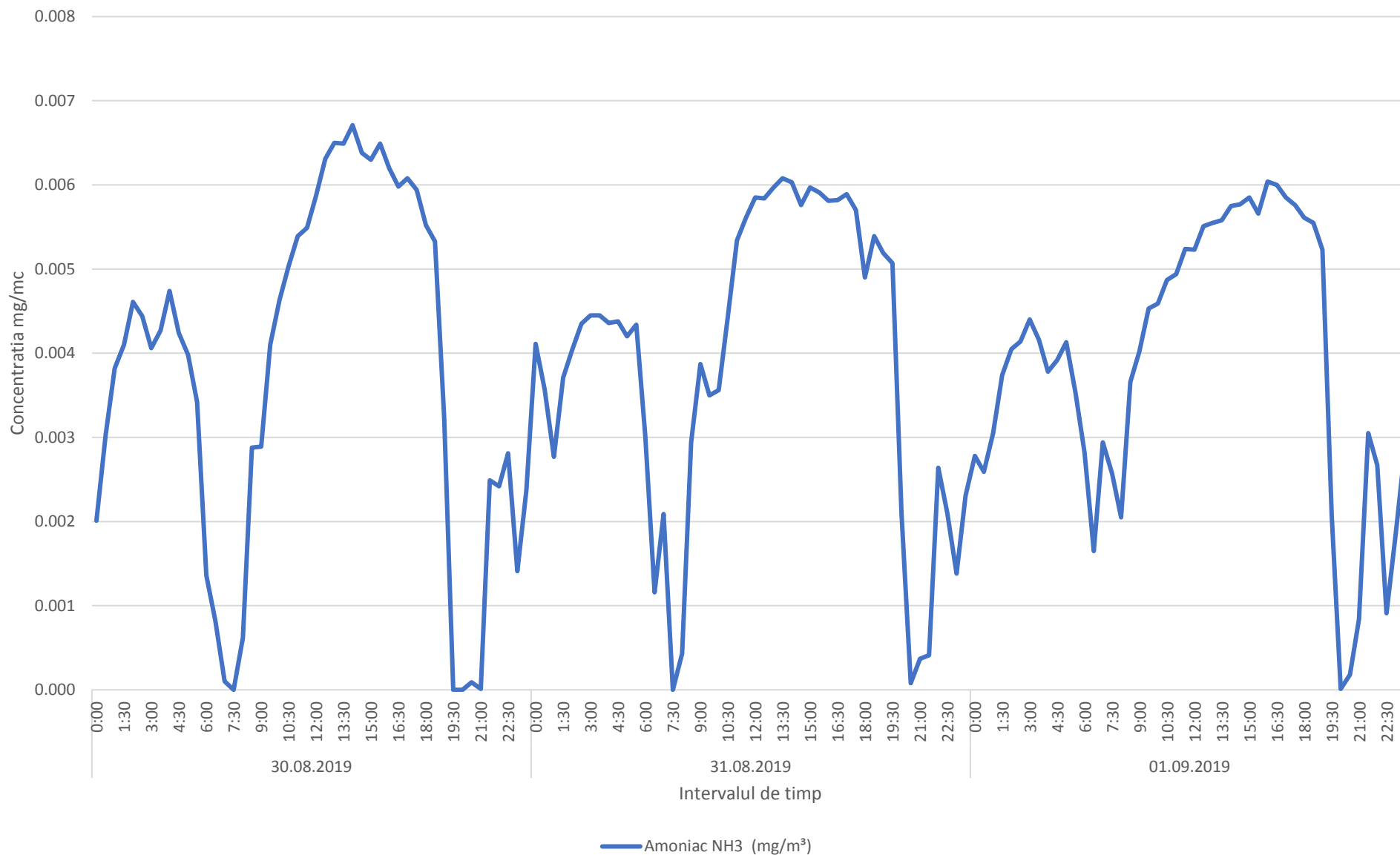
Variatia momentana (30 min.) a indicatorului NH3 in perioada 30.08.2019-01.09.2019- zona Oras Plopeni
