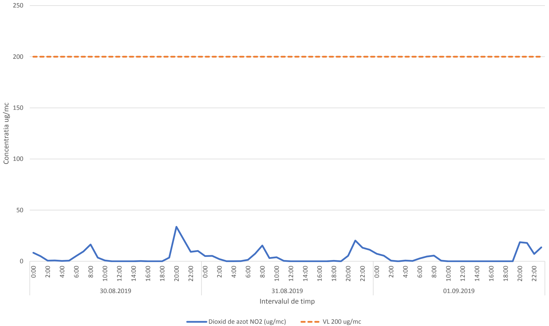
Variatia mediilor orare ale indicatorului NO2 in perioada 30.08.2019-01.09.2019- zona Oras Plopeni
