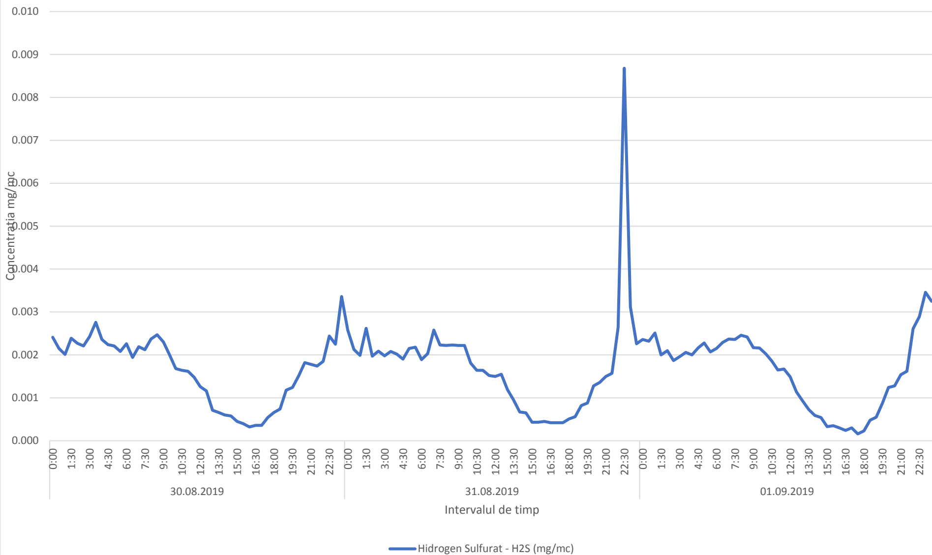
Variatia momentana (30 min.) a indicatorului H2S in perioada 30.08.2019-01.09.2019- zona Oras Plopeni
