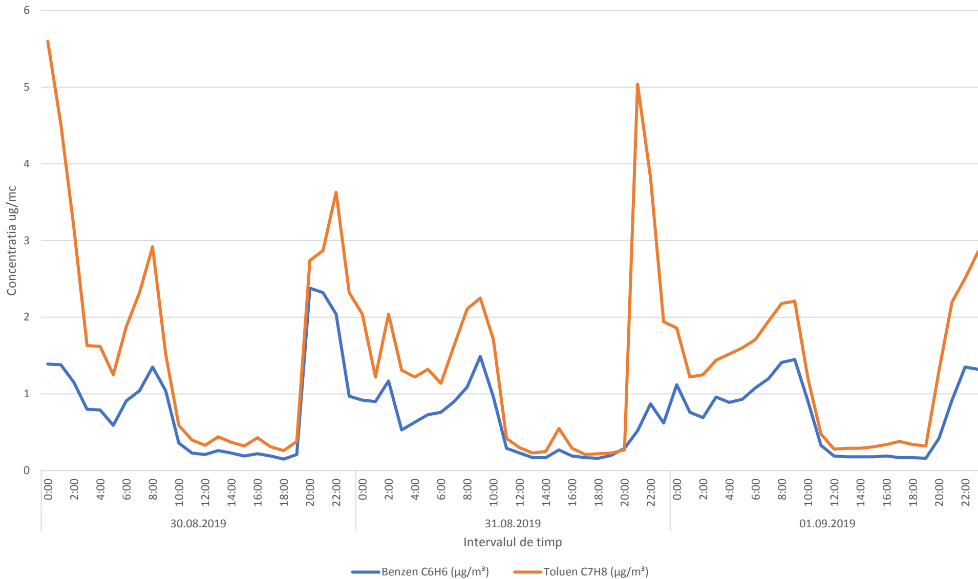
Variatia mediilor orare a indicatorilor C6H6,C7H8 in perioada 30.08.2019-01.09.2019- zona Oras Plopeni
