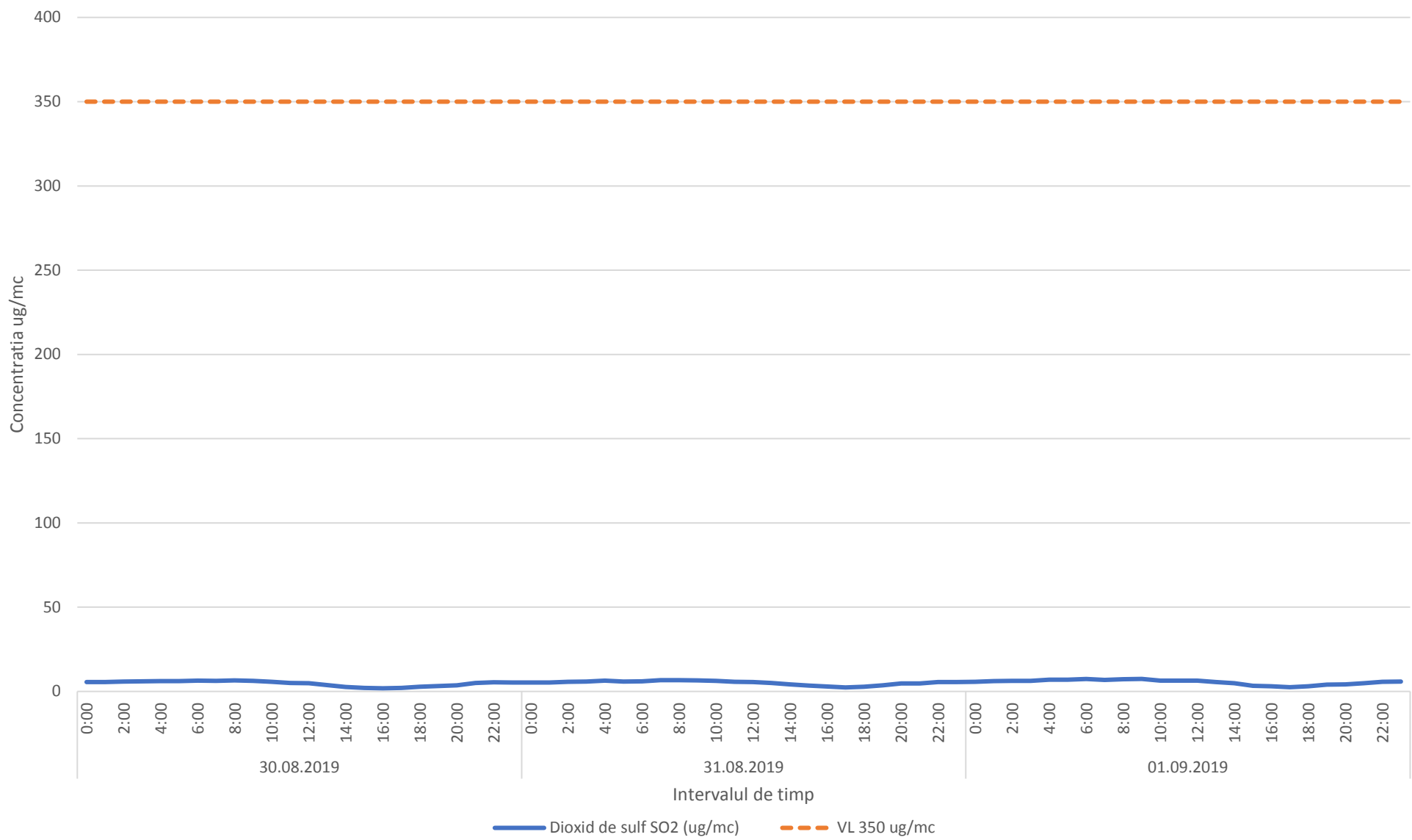
Variatia mediilor orare ale indicatorului SO2 in perioada 30.08.2019-01.09.2019- zona Oras Plopeni
