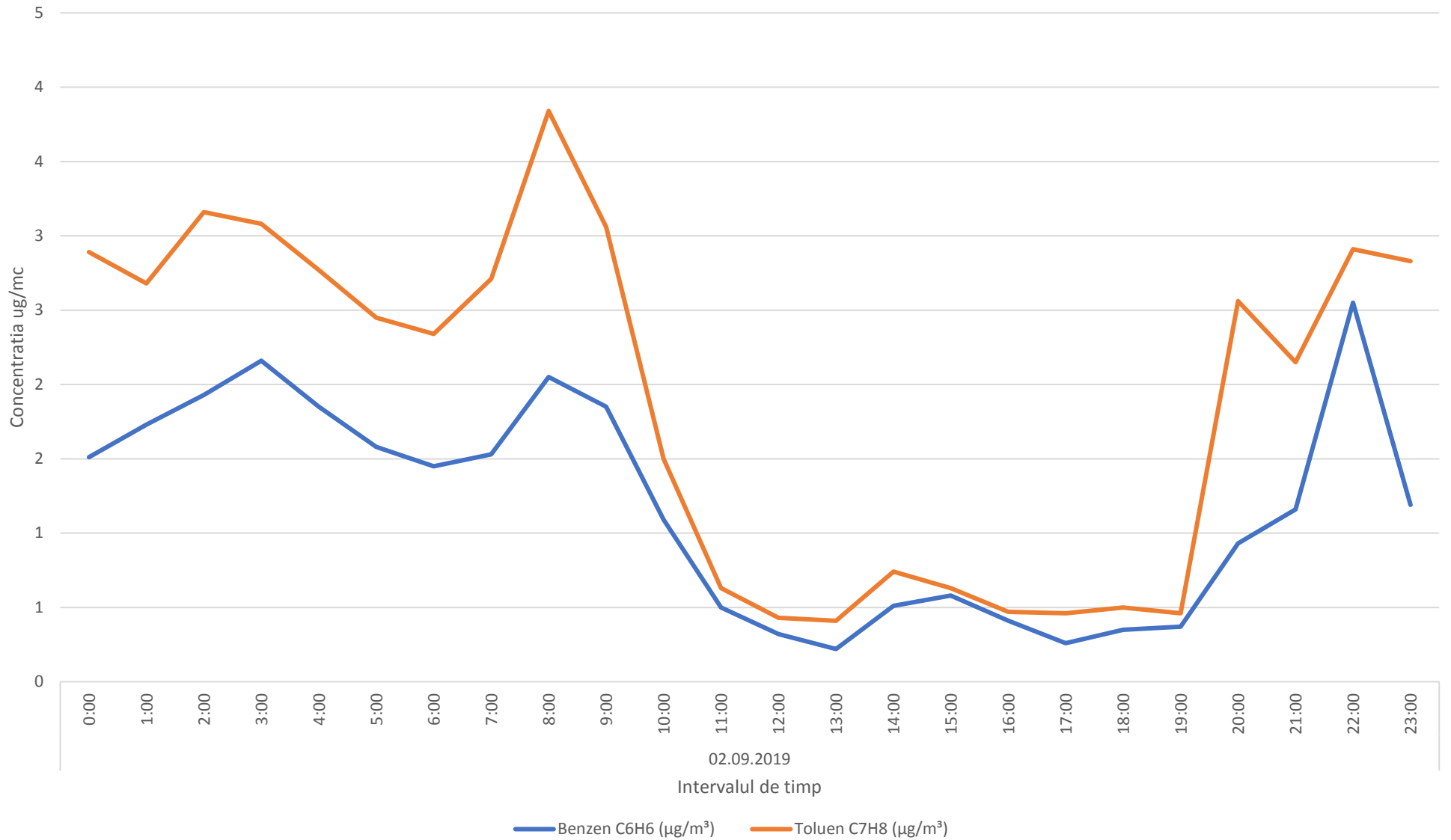
Variatia mediilor orare a indicatorilor C6H6,C7H8 in data de 02.09.2019- zona Oras Plopeni
