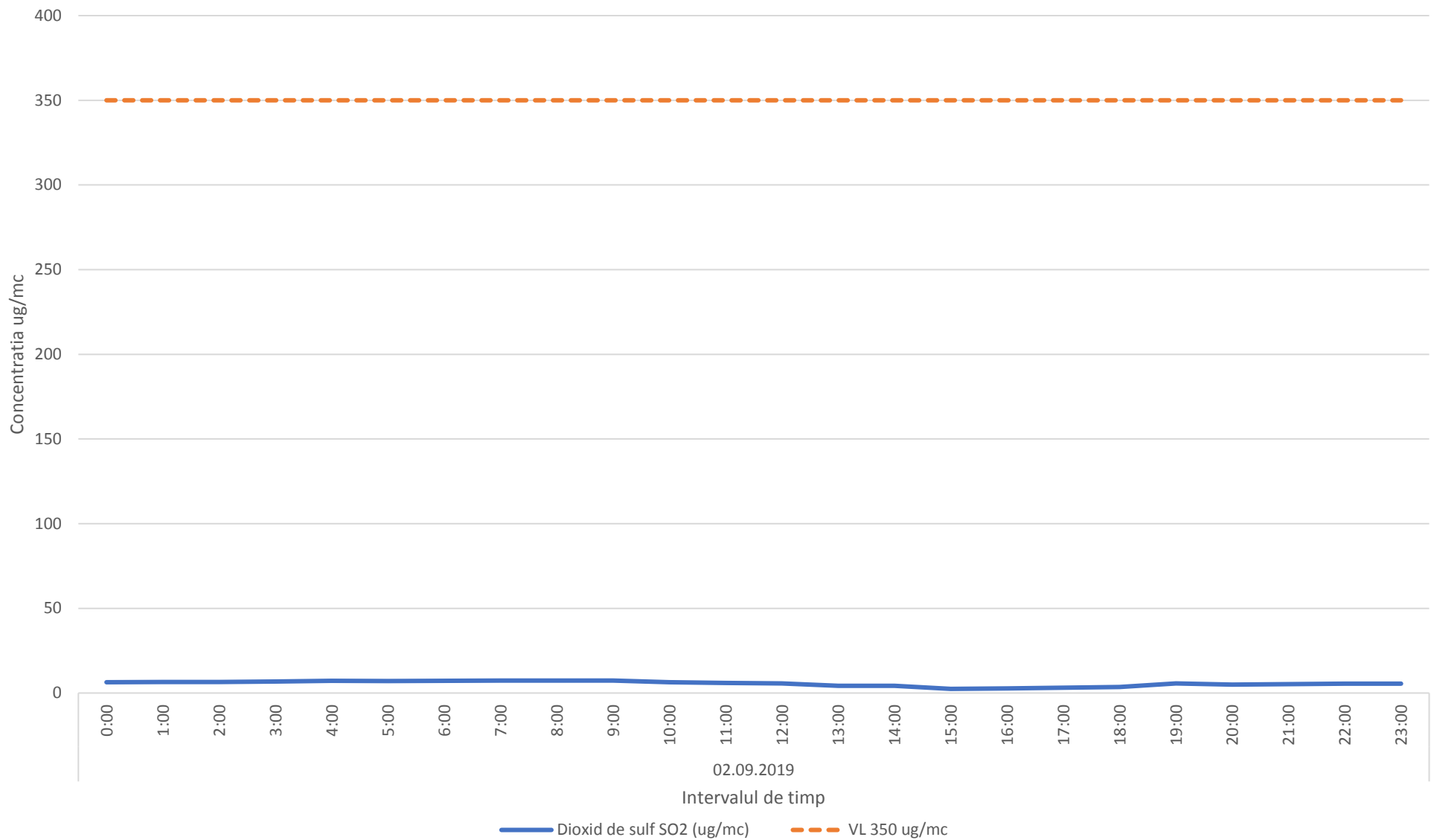
Variatia mediilor orare ale indicatorului SO2 in data de 02.09.2019- zona Oras Plopeni
