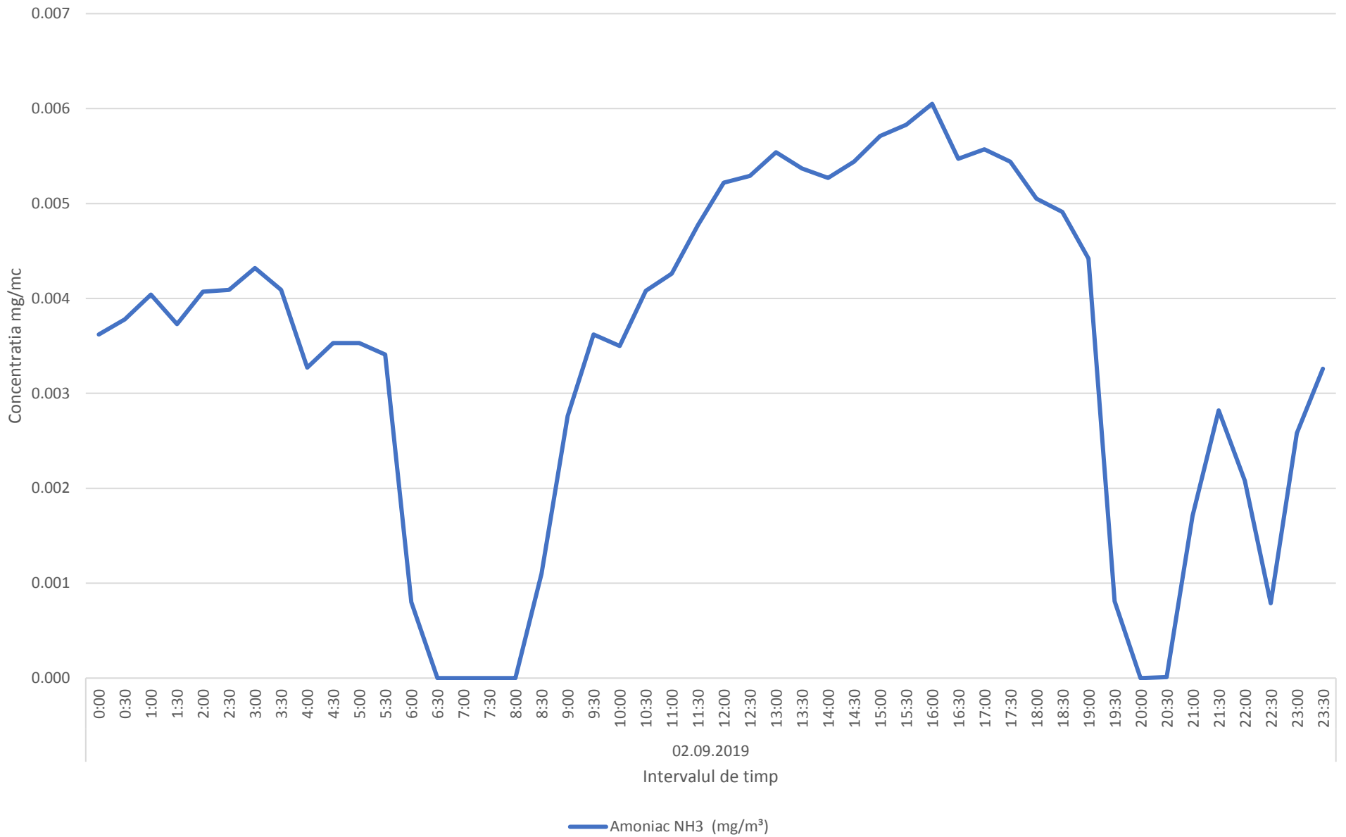
Variatia momentana (30 min.) a indicatorului NH3 in data de 02.09.2019- zona Oras Plopeni
