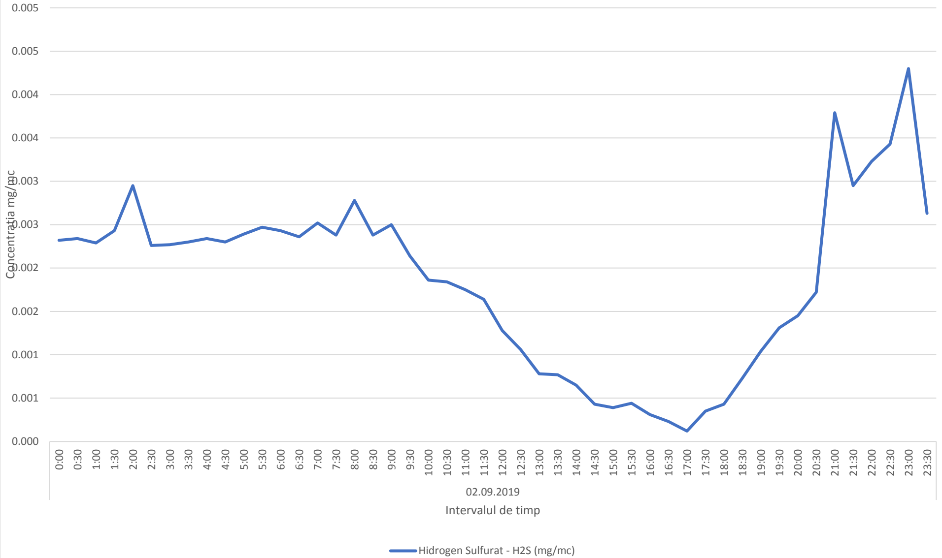
Variatia momentana (30 min.) a indicatorului H2S in data de 02.09.2019- zona Oras Plopeni
