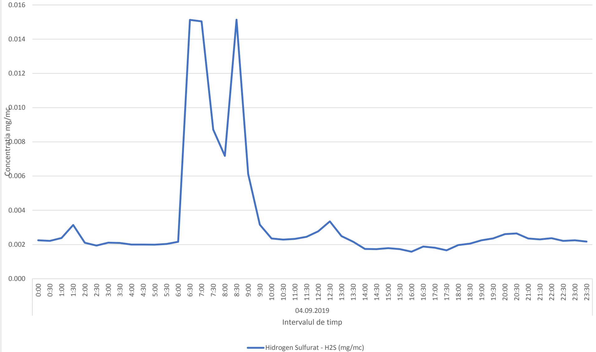
Variatia momentana (30 min.) a indicatorului H2S in data de 04.09.2019- zona Oras Plopeni
