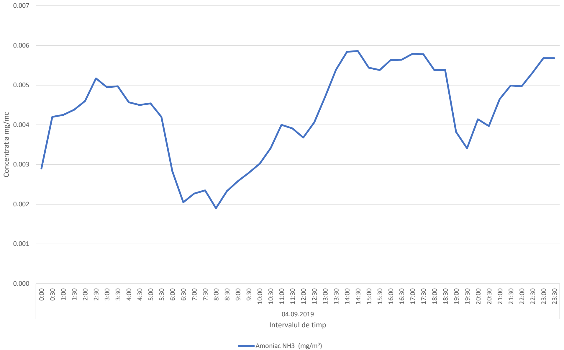
Variatia momentana (30 min.) a indicatorului NH3 in data de 04.09.2019- zona Oras Plopeni
