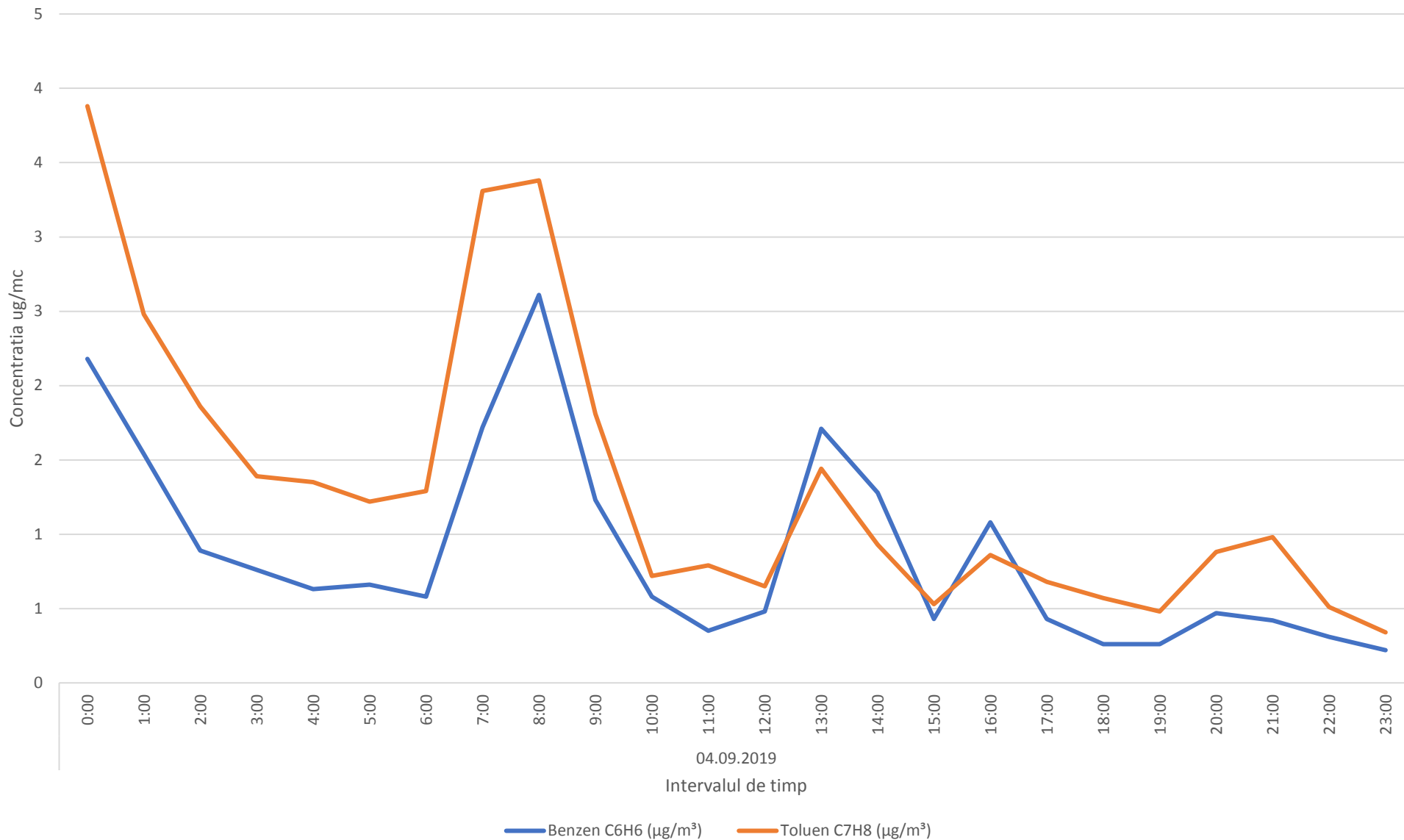
Variatia mediilor orare a indicatorilor C6H6,C7H8 in data de 04.09.2019- zona Oras Plopeni
