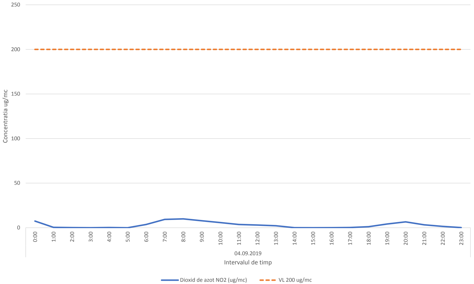
Variatia mediilor orare ale indicatorului NO2 in data de 04.09.2019- zona Oras Plopeni
