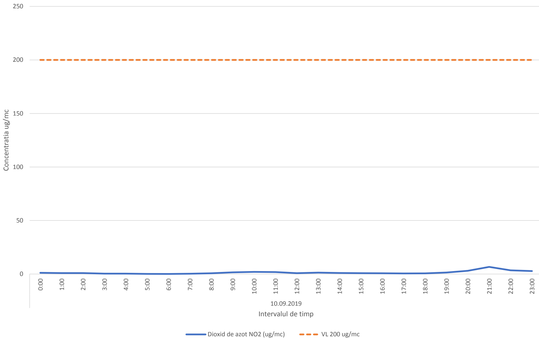
Variatia mediilor orare ale indicatorului NO2 in data de 10.09.2019- zona Comunei Paulesti
