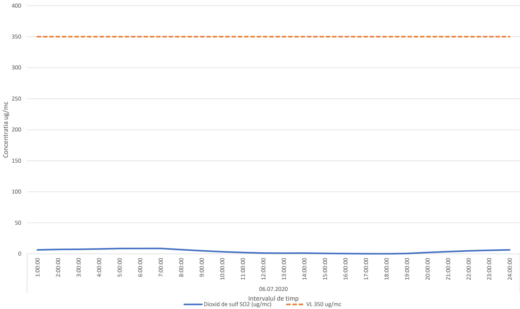
Variatia mediilor orare ale indicatorului SO2 in data de 06.07.2020 - comuna Barcanesti
