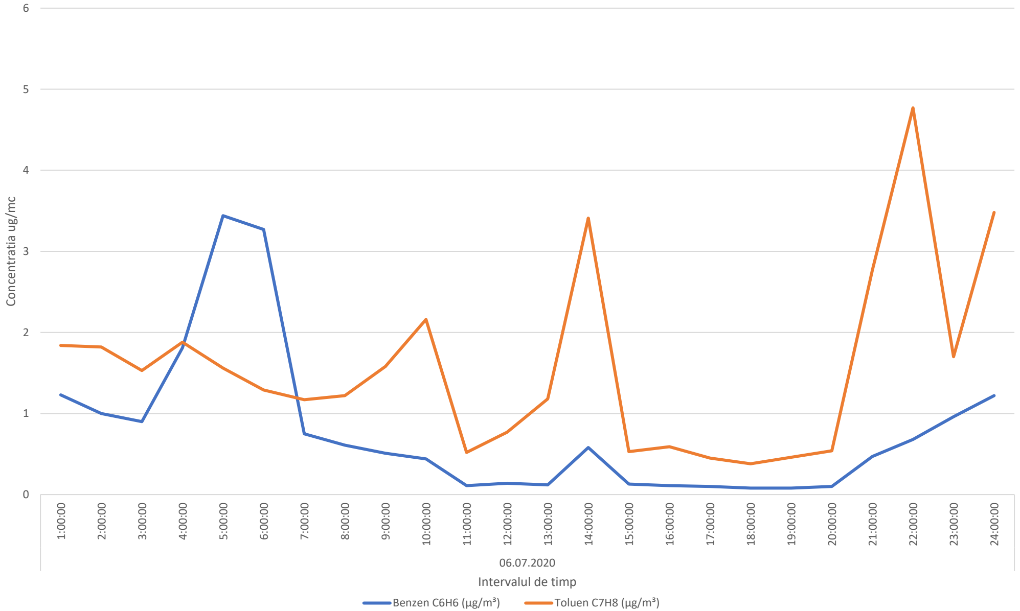
Variatia mediilor orare ale indicatorilor C6H6/C7H8 in data de 06.07.2020 - comuna Barcanesti
