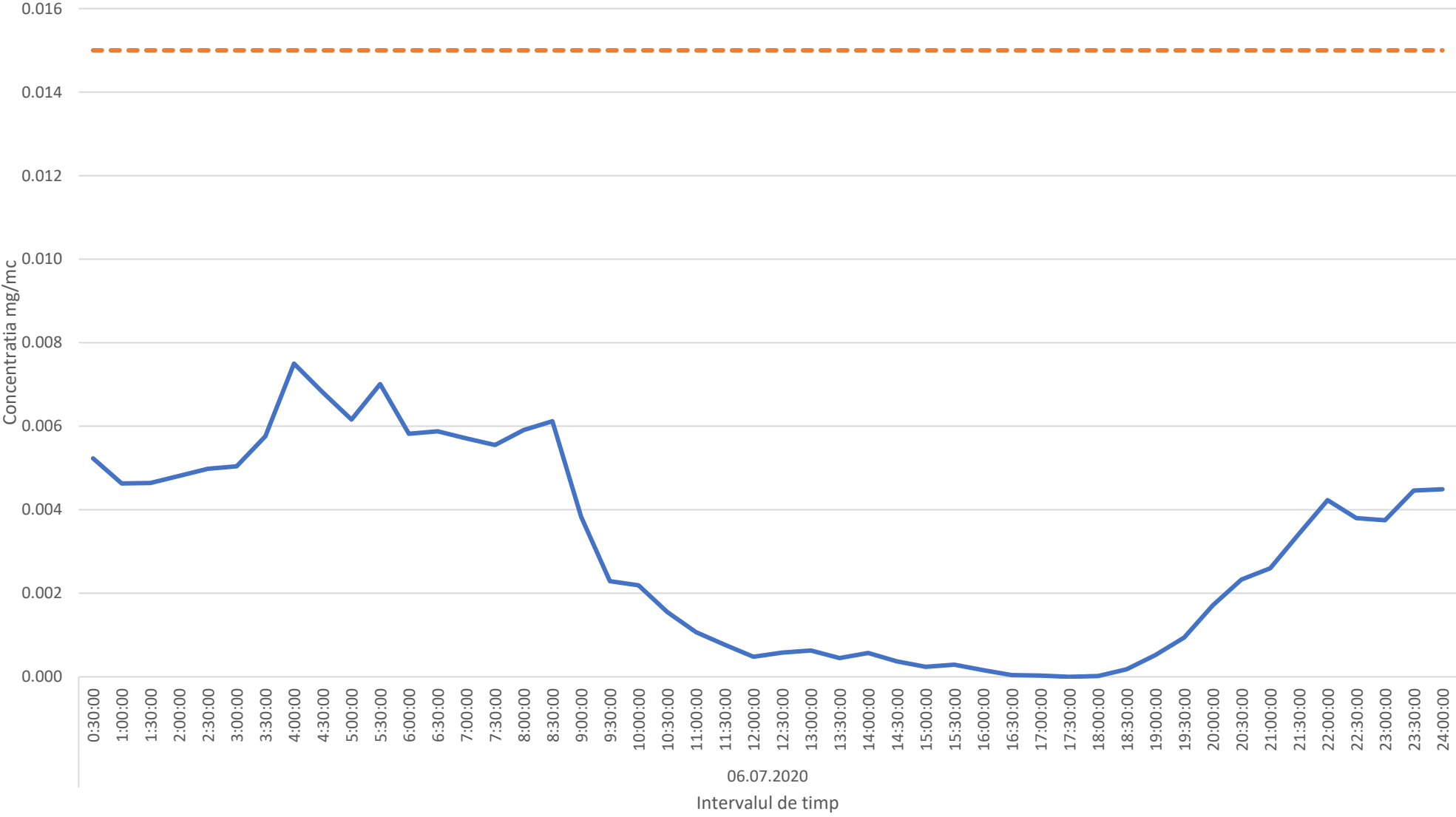
Variatia momentana (30 min.) a indicatorului H2S in data de 06.07.2020 - comuna Barcanesti
