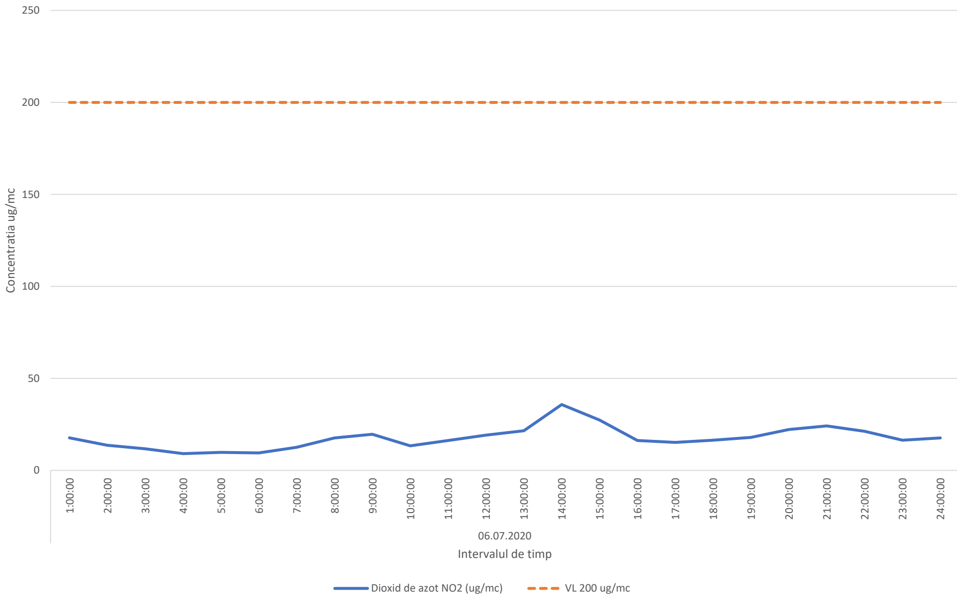
Variatia mediilor orare ale indicatorului NO2 in data de 06.07.2020 - comuna Barcanesti
