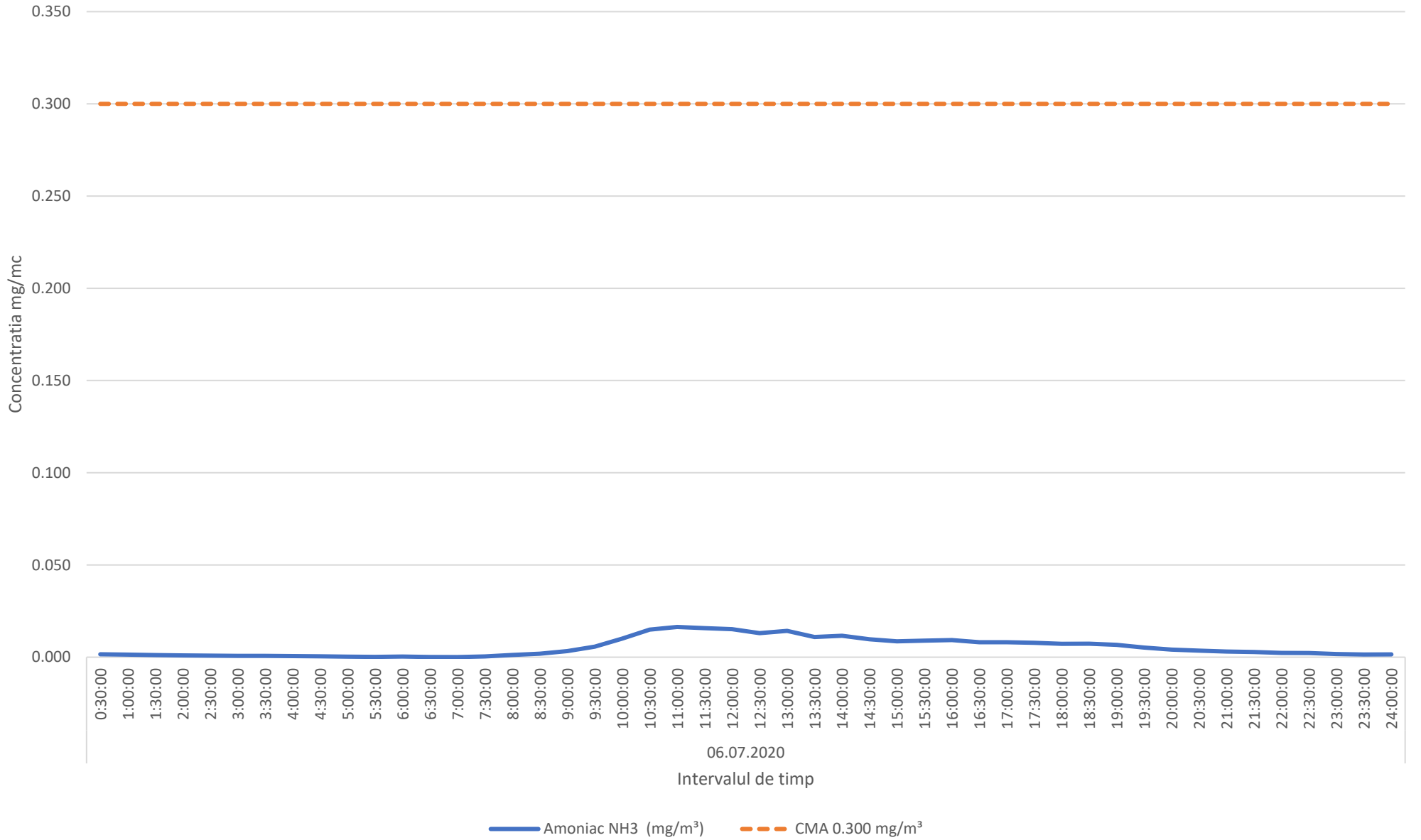
Variatia momentana (30 min.) a indicatorului NH3 in data de 06.07.2020 -comuna Barcanesti
