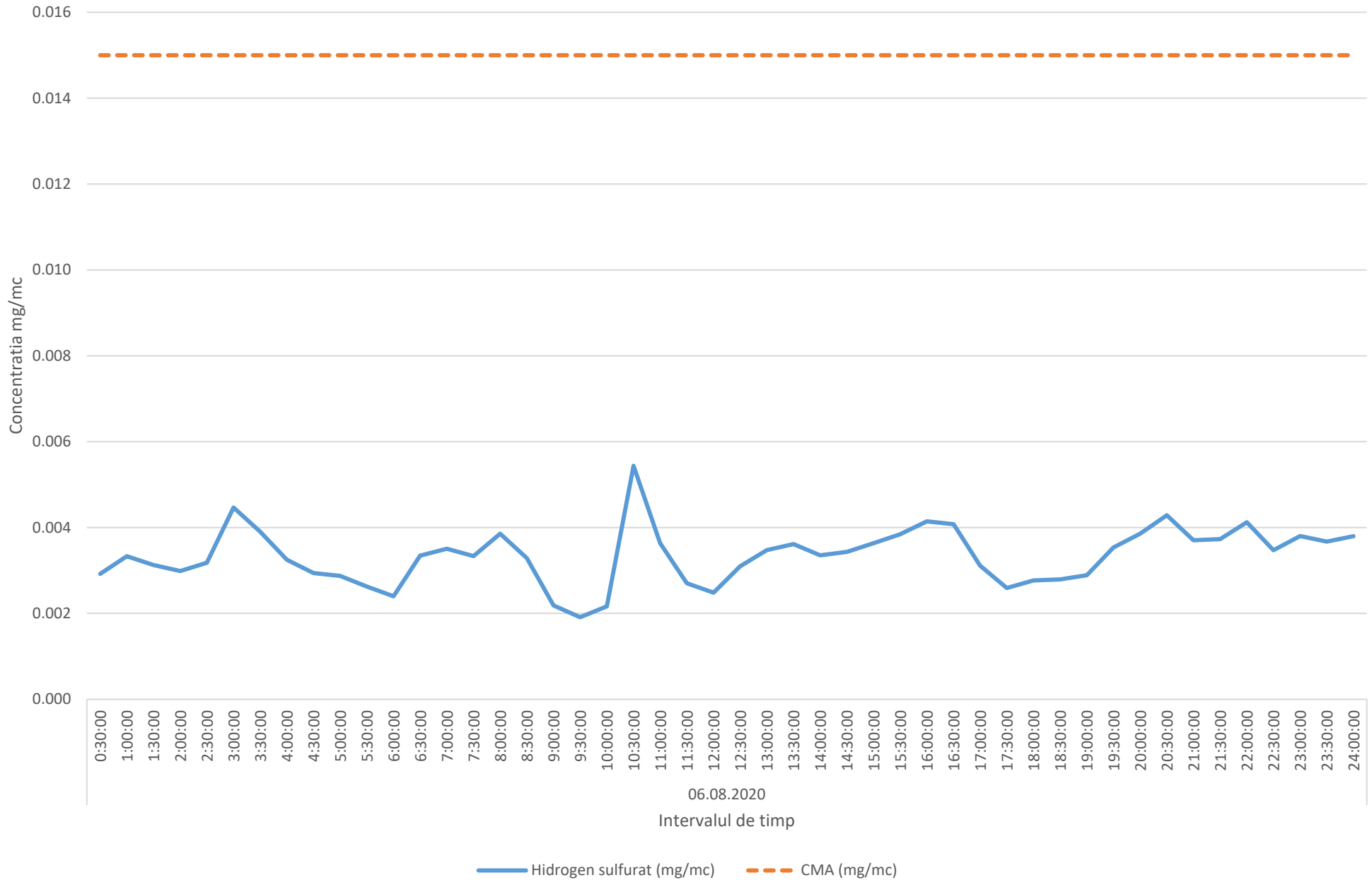
Variatia momentana (30 min.) a indicatorului H2S in data de 06.08.2020 - Sala Sporturilor Olimpia
