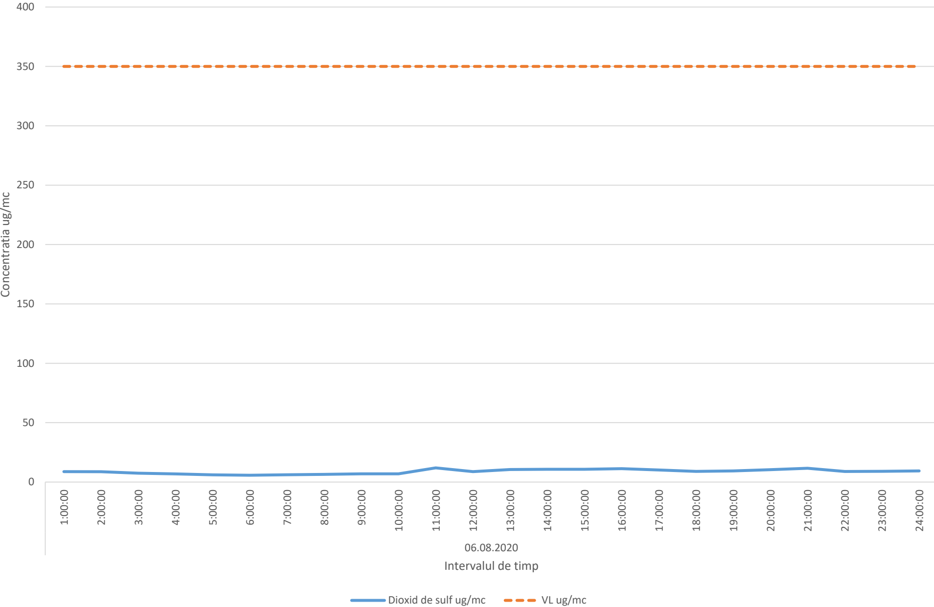
Variatia mediilor orare ale indicatorului SO2 in data de 06.08.2020- Sala Sporturilor Olimpia
