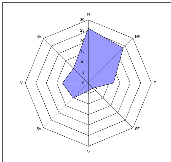
Figura 8. Roza vânturilor
