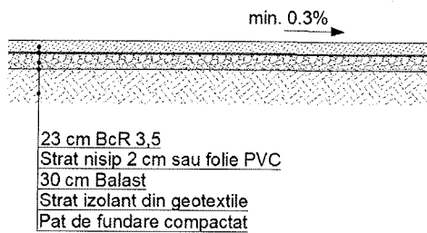
fig.1 Detaliu alcătuire
