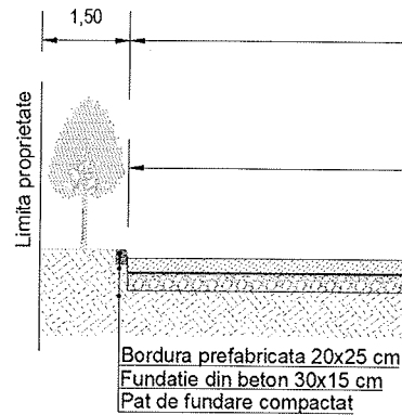
fig.2 Detaliu alcătuire
