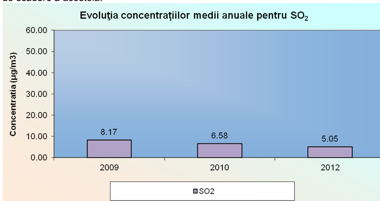
Fig. I.1.8. Evoluția concentrațiilor medii anuale pentru SO 2
