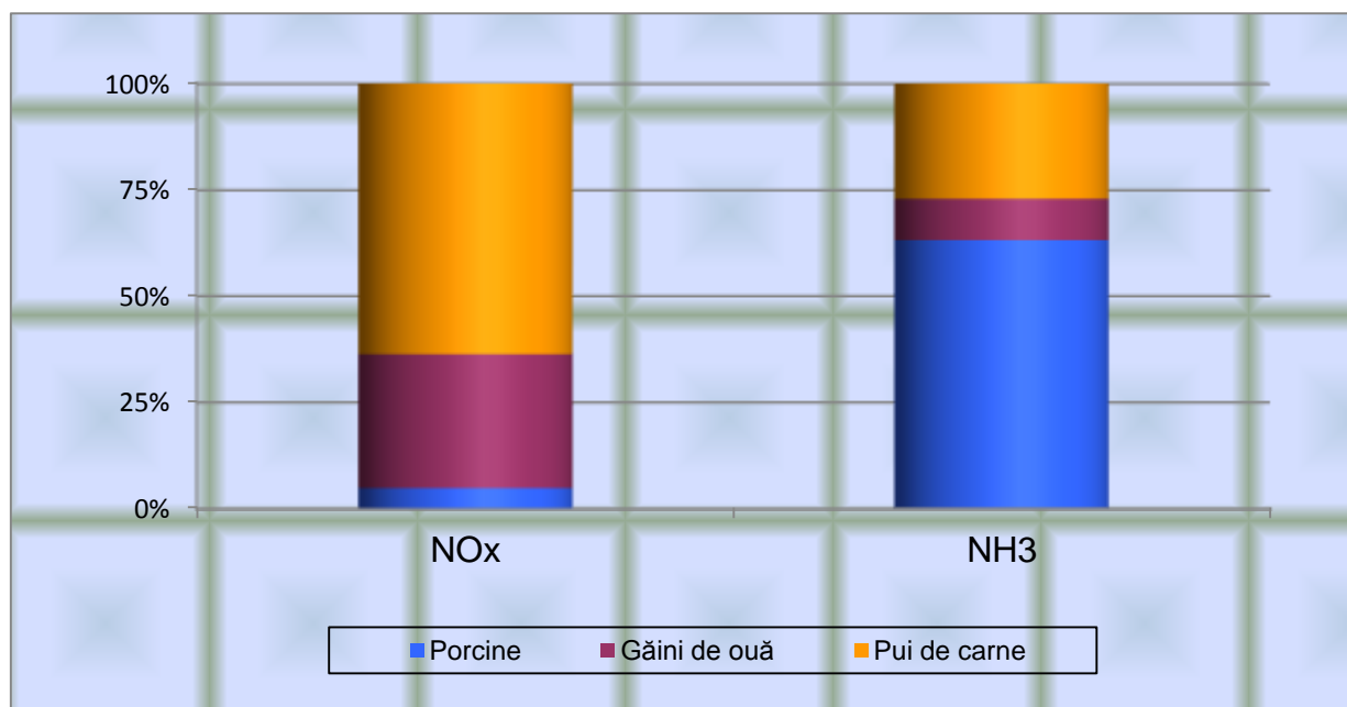
Fig. I.2.30. Pondere emisiilor de substanțe acidifiante, pe sectoare de activitate din agricultură pentru anul 2016
