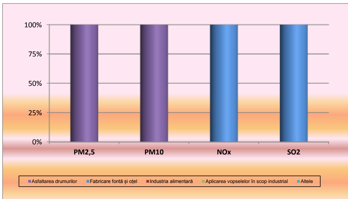
Fig. I.2.15. Ponderea emisiilor de particule prim. și precursori sec. de particule pe sectoare de activitate din industrie – 2015
