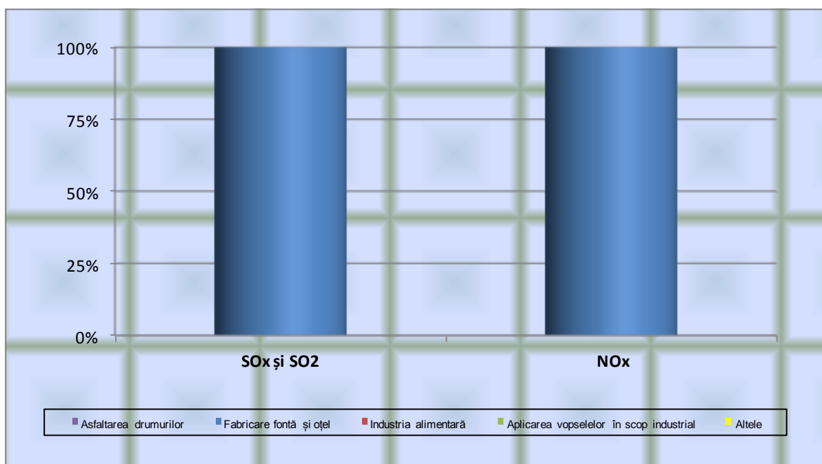
Fig. I.2.11. Ponderea emisiilor de substanțe acidifiante, pe sectoare de activitate din industrie pentru anul 2015
