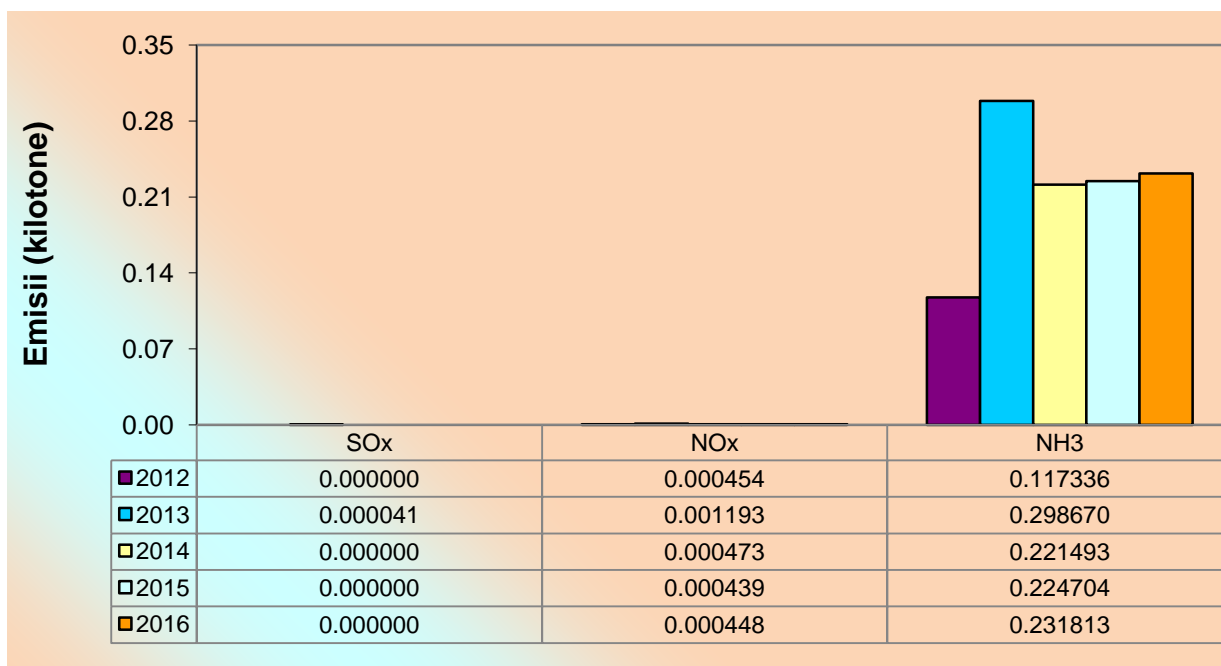
Fig. I.3.5. Evoluția emisiilor de substanțe acidifiante din agricultură, în perioada 2012 - 2016
