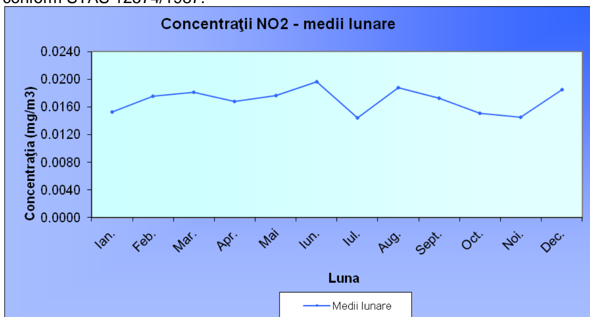
I.1.2. Concentrații de NO 2 (măsurători zilnice) – medii lunare
