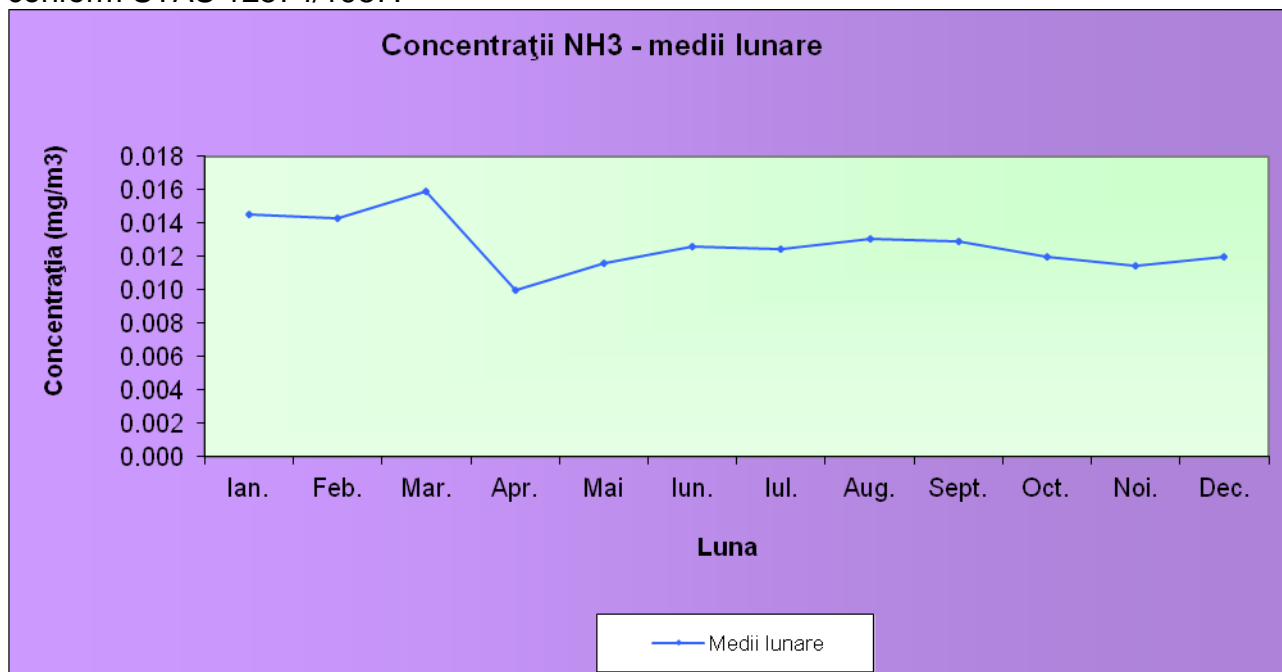
Fig. I.1.6. Concentrații de NH 3 – medii lunare
