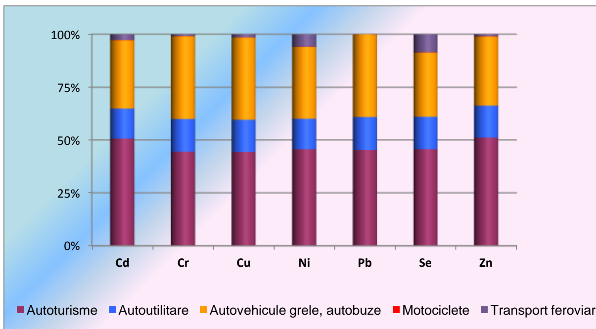
Fig. I.2.28 Pondere emisiilor de metale grele pe tipuri de vehicule de transport – 2016
