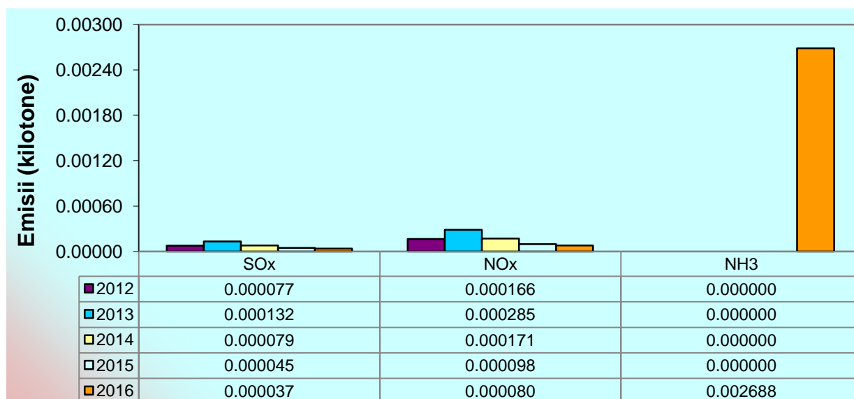
Fig. I.3.3. Evoluția emisiilor de substanțe acidifiante din industrie, în perioada 2012 - 2016
