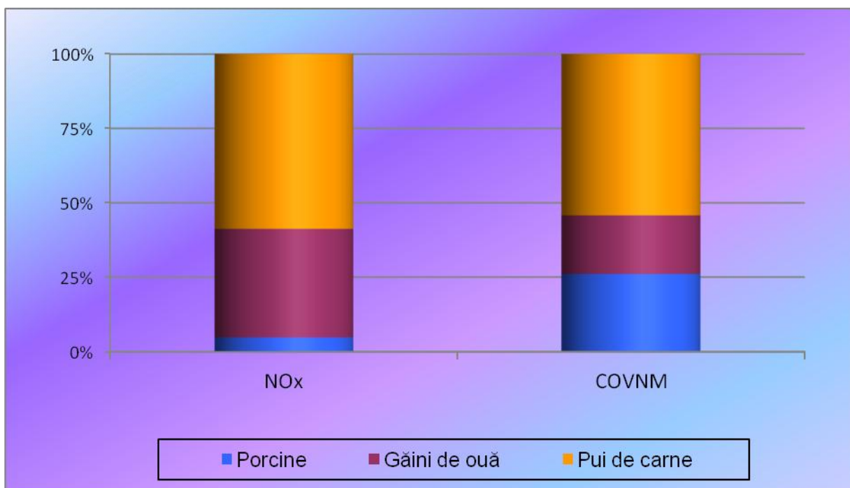
Fig. I.2.31. Ponderea emisiilor de precursori ai ozonului, pe sectoare de activitate din agricultură – 2015
