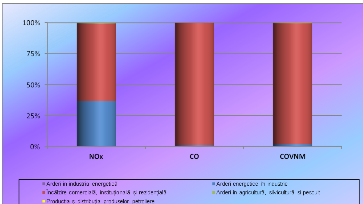
Fig. I.2.4. Pondere emisiilor de precursori ai ozonului, pe sectoare de activitate din energie pentru anul 2016
