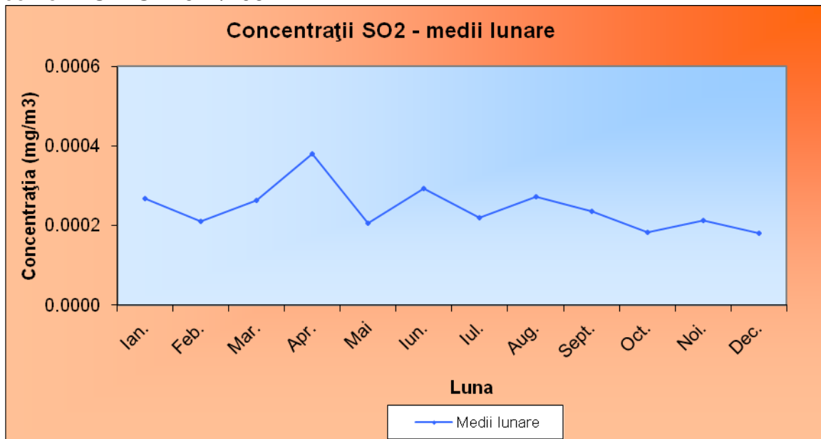
I.1.3. Concentrații de SO 2 – medii lunare
