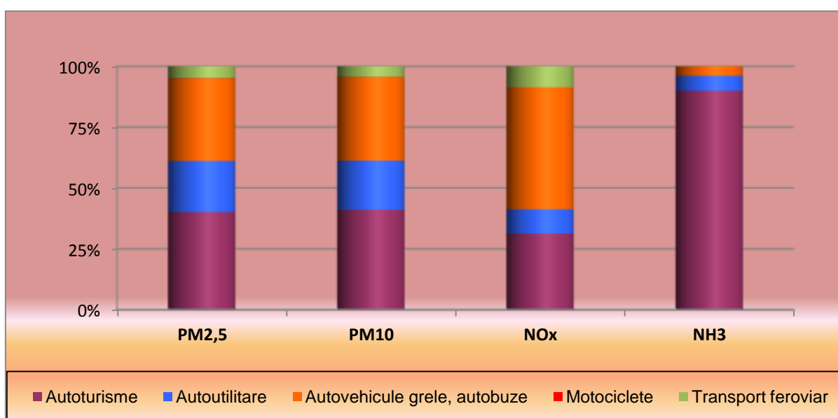
Fig. I.2.25. Ponderea emisiilor de particule prim. și precursori secund. de particule pe tipuri de vehicule de transport pentru anul 2015
