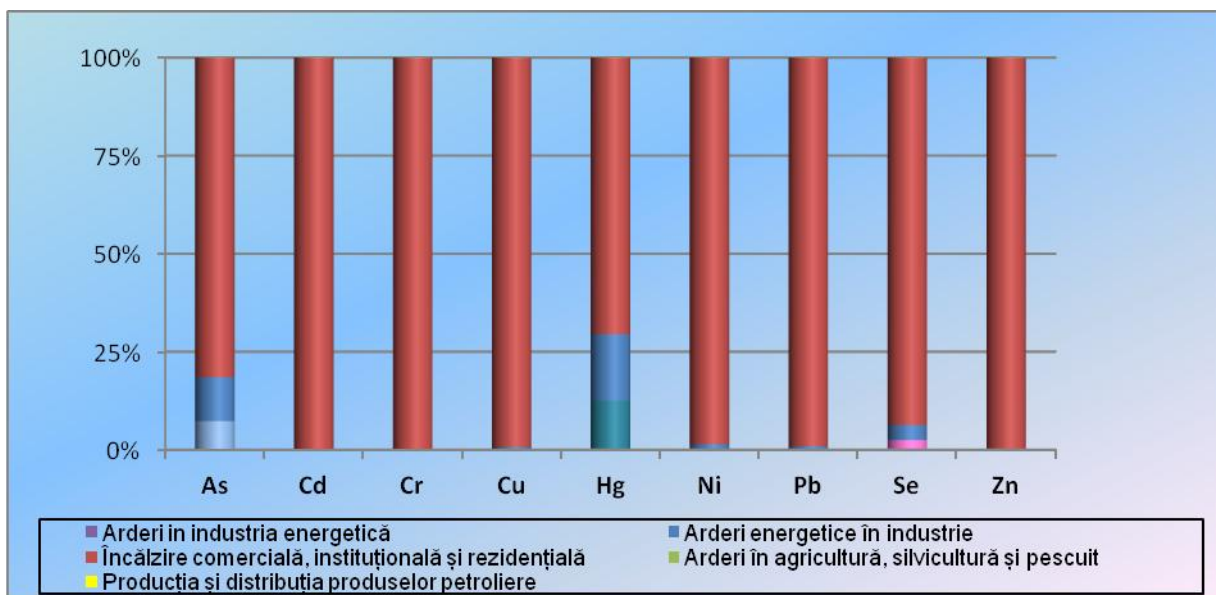
Fig. I.2.7 Pondere emisiilor de metale grele pe sectoare de activitate din energie – 2015
