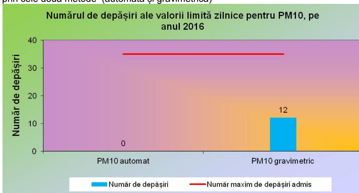
Fig. I.1.12. Numărul de depășiri a valorii limită zilnice pentru PM10
