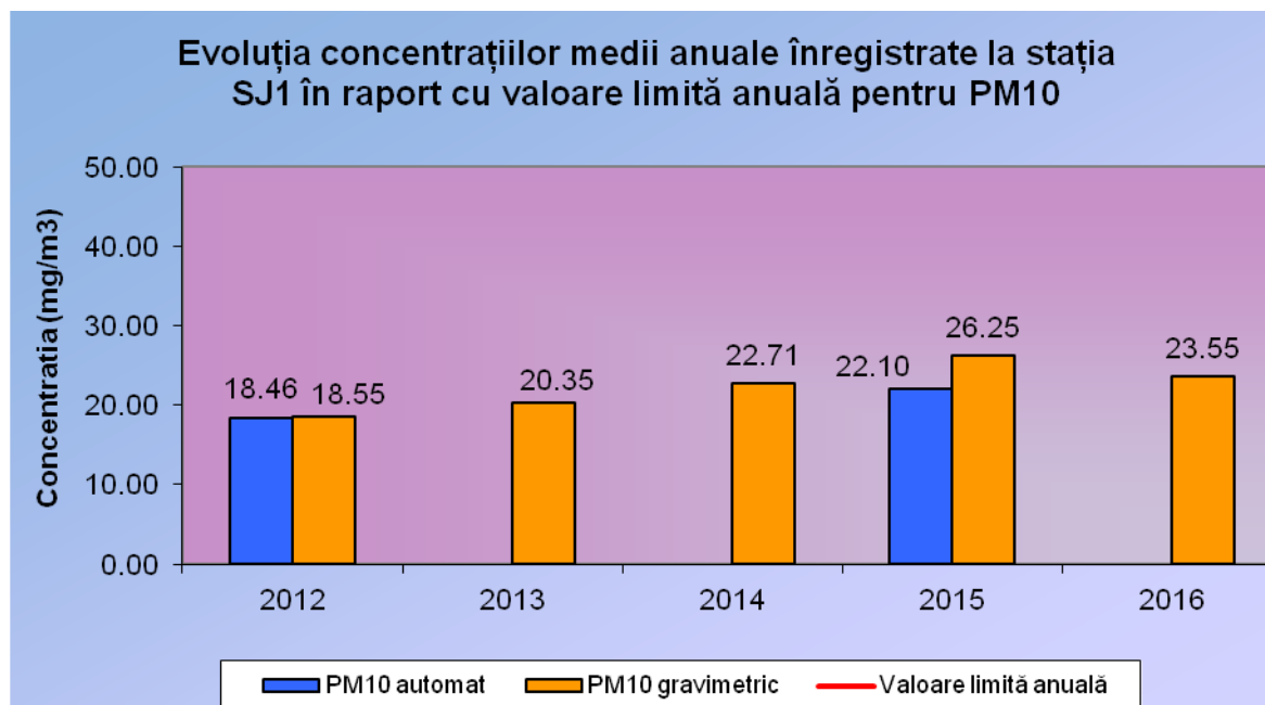
Fig. I.1.11. Evoluția mediilor anuale pentru PM10 automat și PM10 gravimetric
