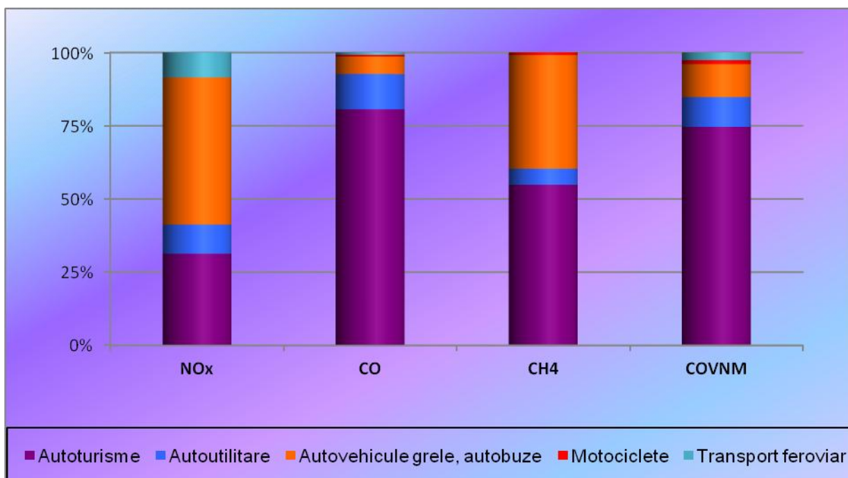
Fig. I.2.23. Ponderea emisiilor de precursori ai ozonului, pe tipuri de vehicule de transport – 2015
