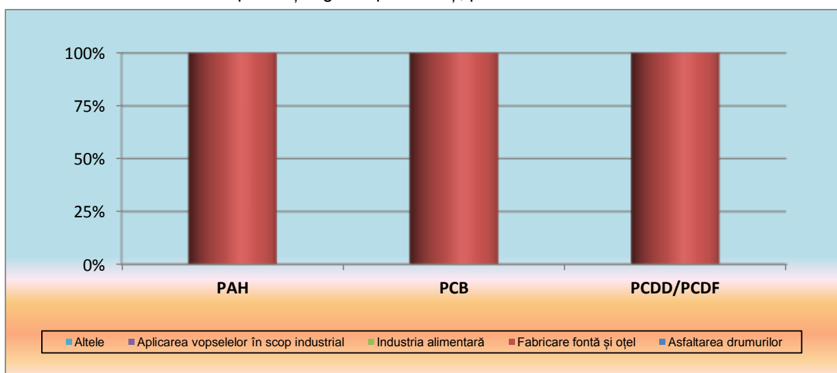
Fig. I.2.19. Pondere emisiilor de poluanți organici persistenti pe sectoare de activitate din industrie pentru anul 2015
