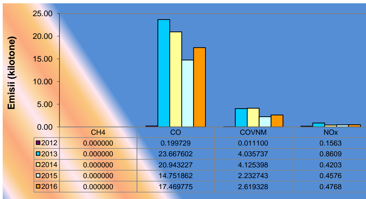
Fig. I.3.7. Evoluția emisiilor de precursori ai ozonului, din sectorul de activitate energie, în perioada 2012 - 2016
