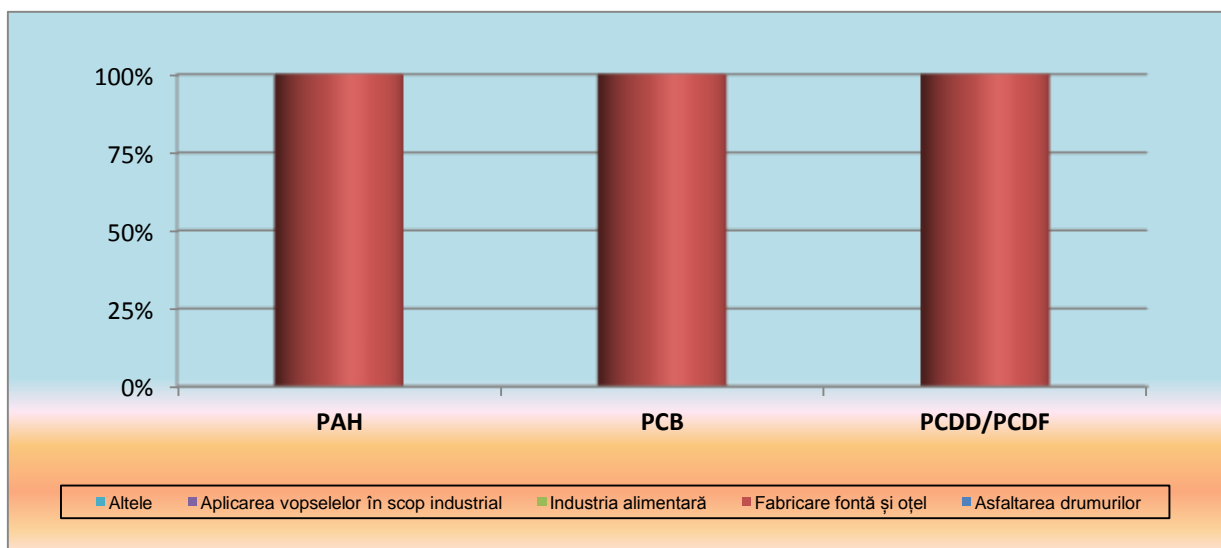
Fig. I.2.20. Pondere emisiilor de poluanți organici persistenți pe sectoare de activitate din industrie pentru anul 2016
