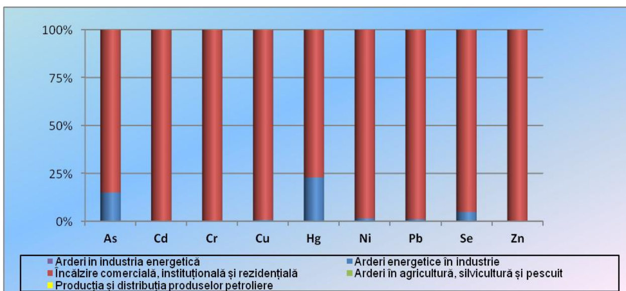
Fig. I.2.8 Pondere emisiilor de metale grele pe sectoare de activitate din energie – 2016
