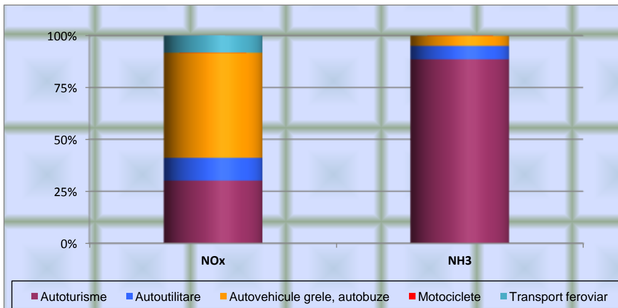
Fig. I.2.22. Ponderea emisiilor de substanțe acidifiante, pe tipuri de vehicule de transport, pentru anul 2016
