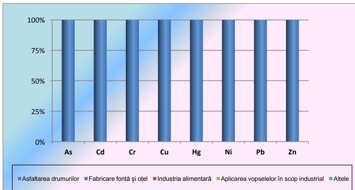
Fig. I.2.17. Ponderea emisiilor de metale grele pe sectoare de activitate din industrie pentru anul 2015
