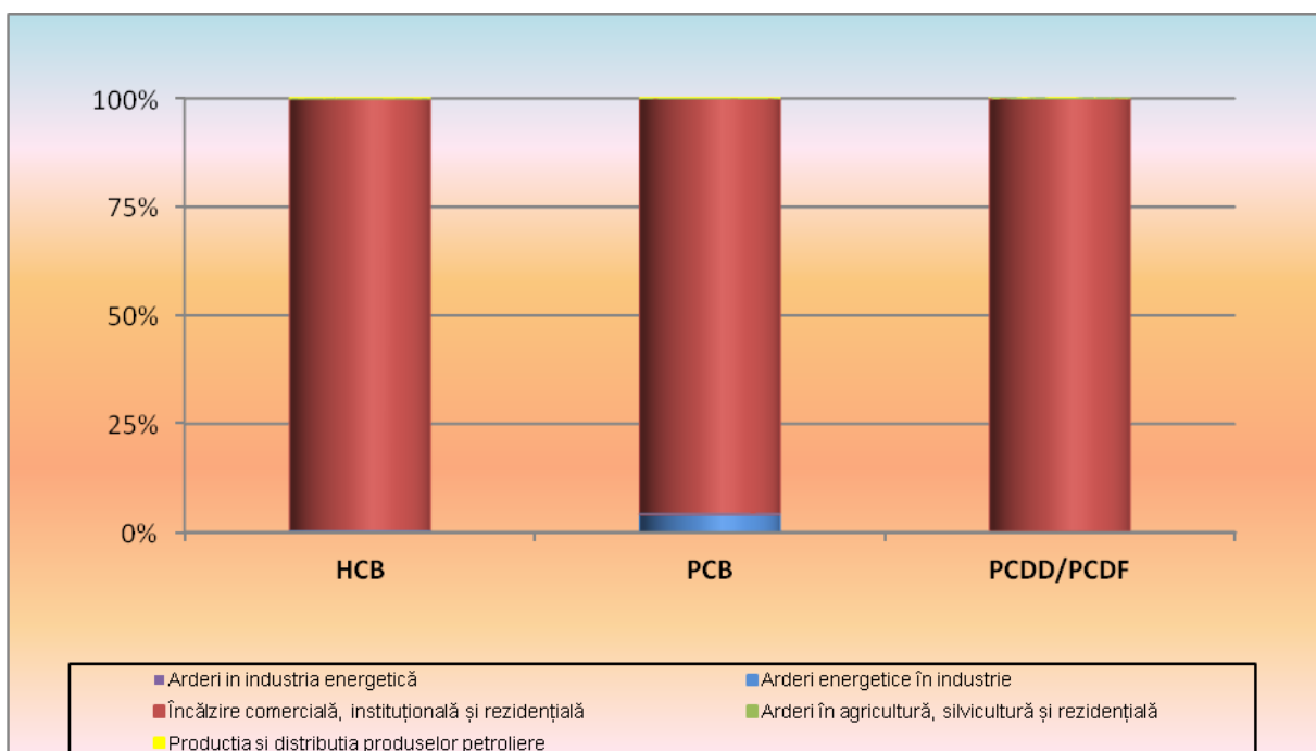
Fig. I.2.10. Pondere emisiilor de poluanți organici persistenti pe sectoare de activitate din energie pentru anul 2016
