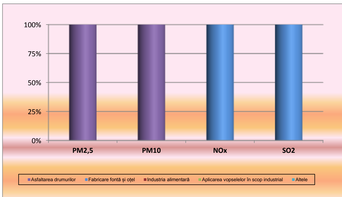
Fig. I.2.16. Ponderea emisiilor de particule prim. și precursori sec. de particule pe sectoare de activitate din industrie – 2016
