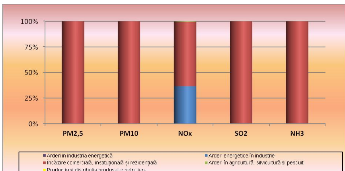
Fig. I.2.6. Ponderea emisiilor de particule prim. și precursori secund. de particule pe sectoare de activitate din energie pentru 2016
