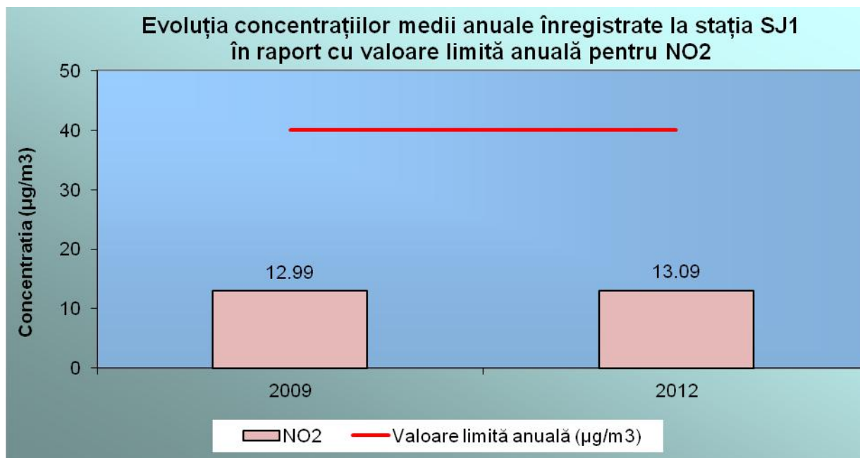
Fig. I.1.7. Evoluția concentrațiilor medii anuale pentru NO 2
