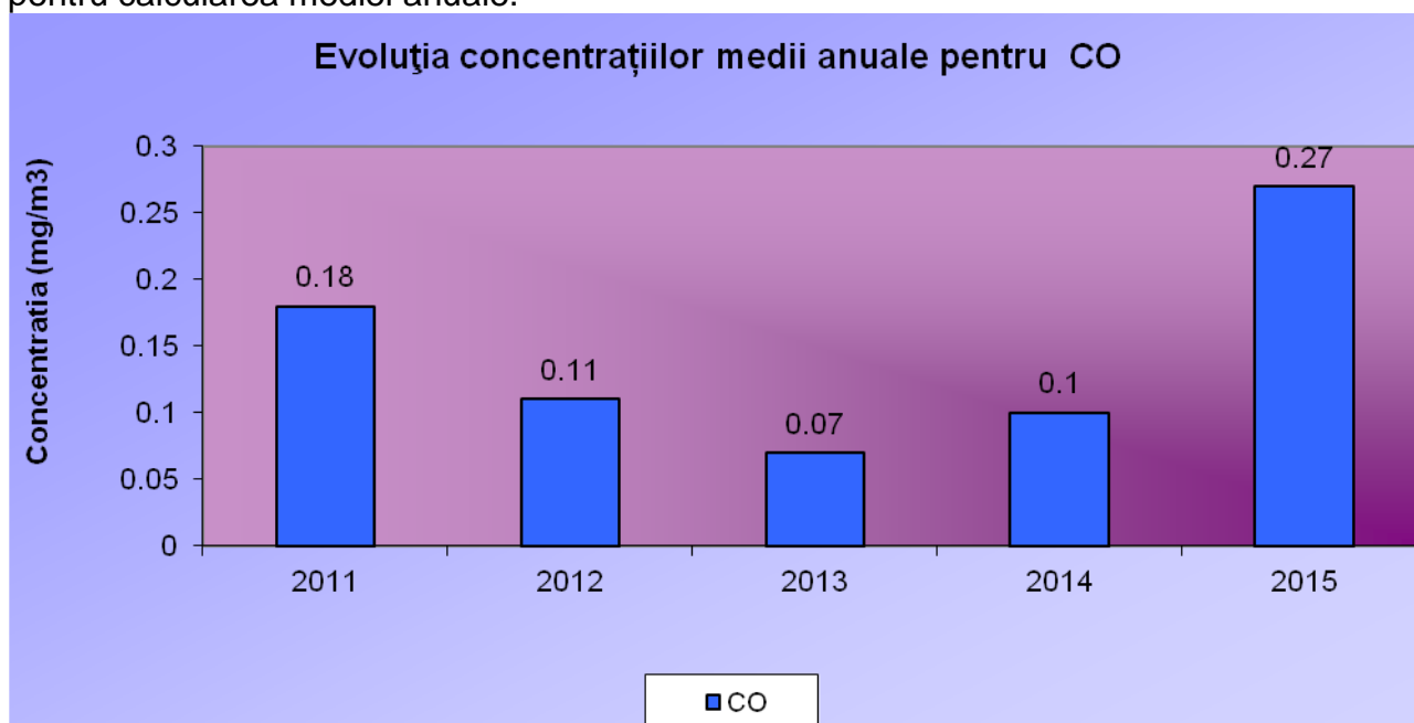
Fig. I.1.10. Evoluția concentrațiilor medii anuale pentru CO
