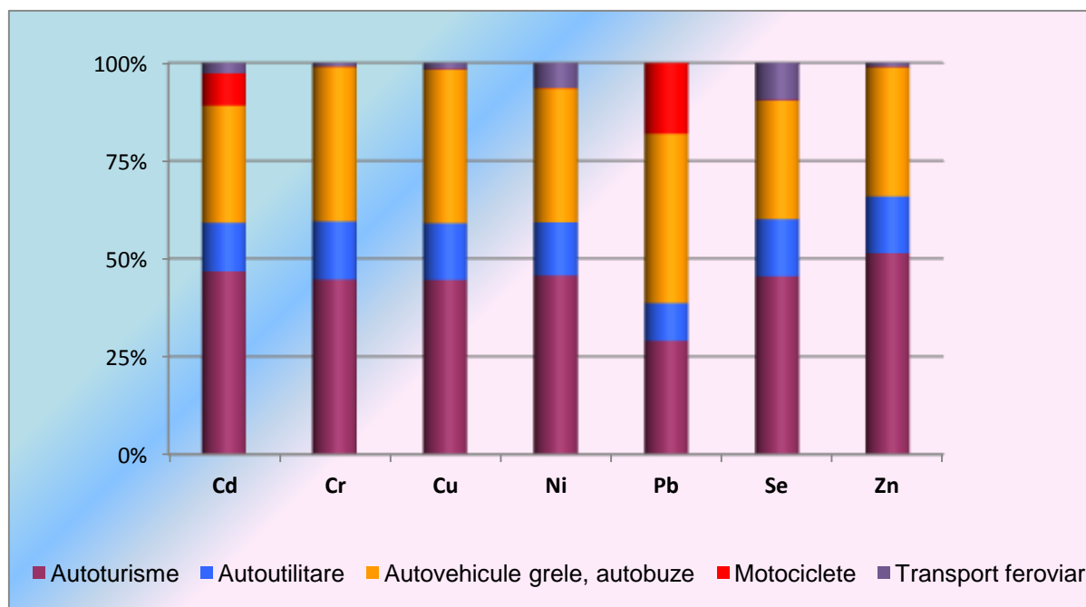
Fig. I.2.27 Pondere emisiilor de metale grele pe tipuri de vehicule de transport – 2015
