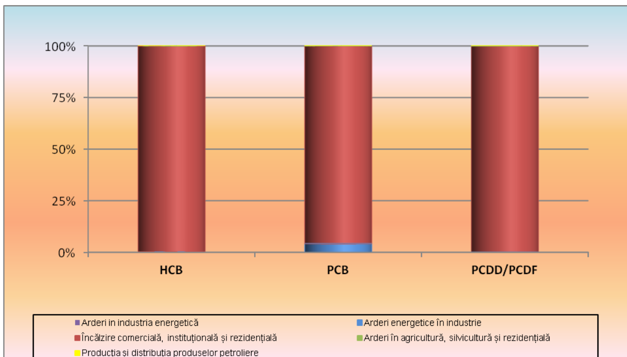
Fig. I.2.9. Pondere emisiilor de poluanți organici persistenti pe sectoare de activitate din energie pentru anul 2015
