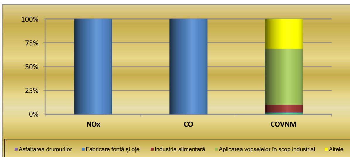
Fig. I.2.13. Ponderea emisiilor de precursori ai ozonului, pe sectoare de activitate din industrie pentru anul 2015
