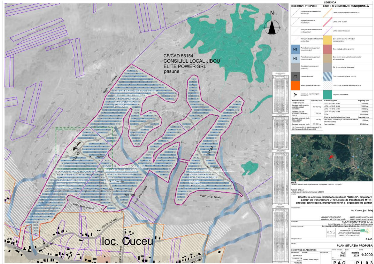
Fig. 3. Plan de situatie parc fotovoltaic
