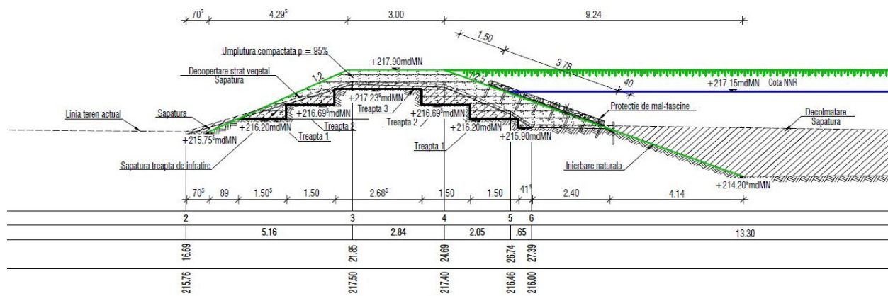
Profilul transversal prin baraj
