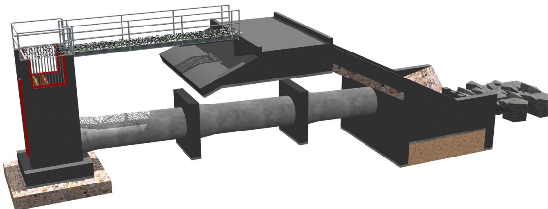
Golirea de fund și descărcătorul de ape mari
