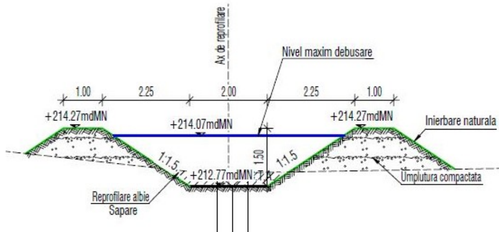
Secțiune tip decolmatare canal de evacuare
