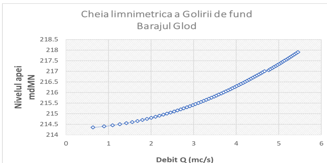
Cheia limnometrică a golirii de fund
