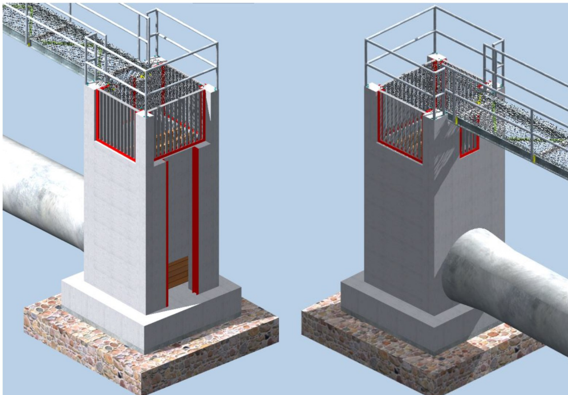
Reprezentarea călugărului/turnului de manevră și a pasarelei de acces
