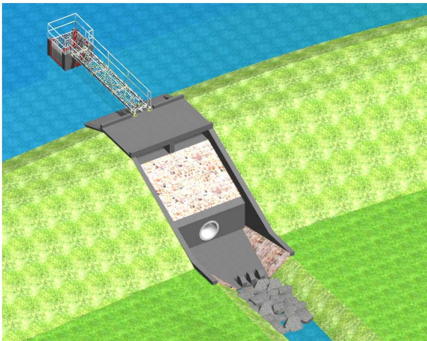
Goliria de fund și disipatorul de energie
