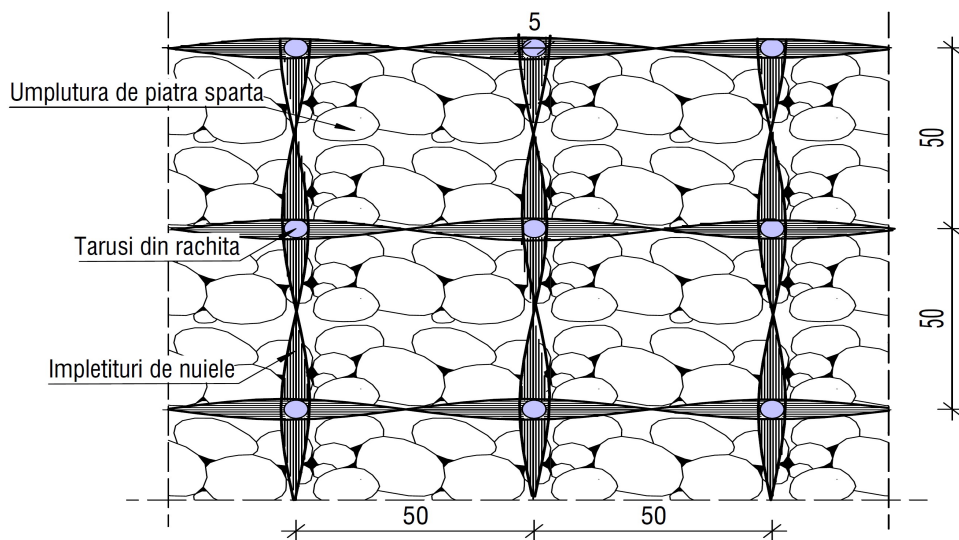
Detaliu protecției de mal amonte cleionaje din fascine lestate cu piatră
