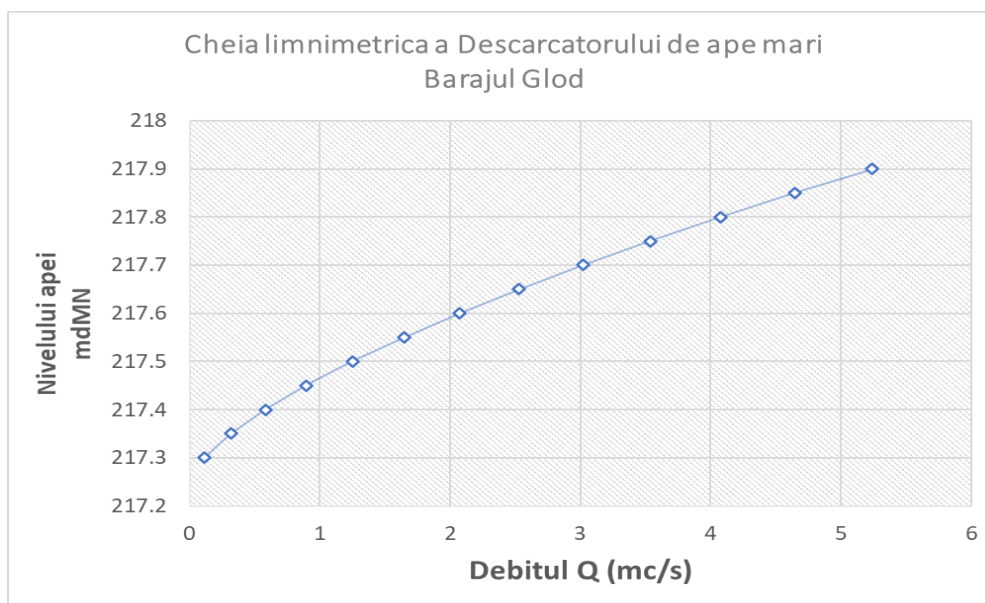
Cheia limnometrică a descărcătorului de ape mari
