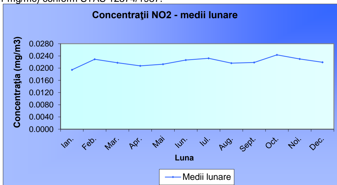
Fig. I.1.4. Concentrații de NO 2 (măsurători zilnice) – medii lunare
