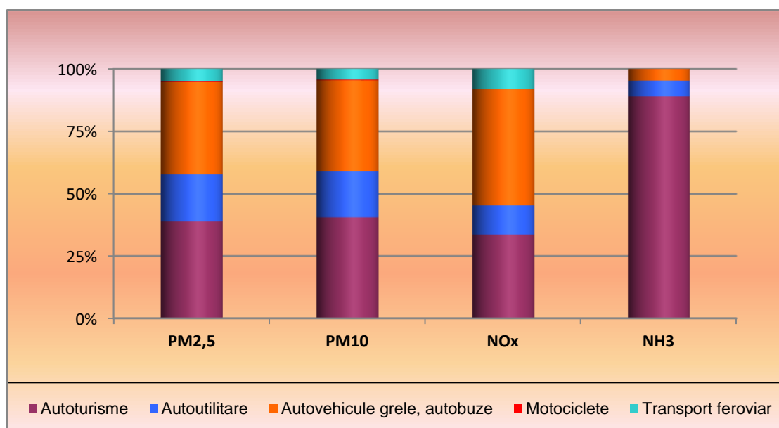
Fig. I.2.13. Pondere emisiilor de particule prim. și precursori secund. de particule pe tipuri de vehicule de transport
