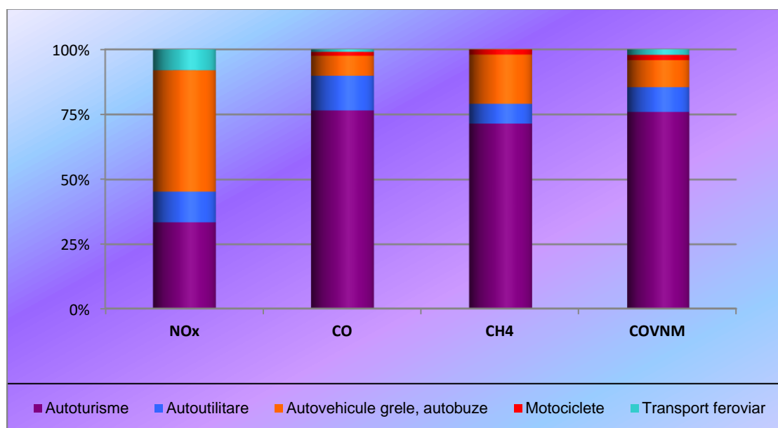
Fig. I.2.12. Pondere emisiilor de precursori ai ozonului, pe tipuri de vehicule de transport
