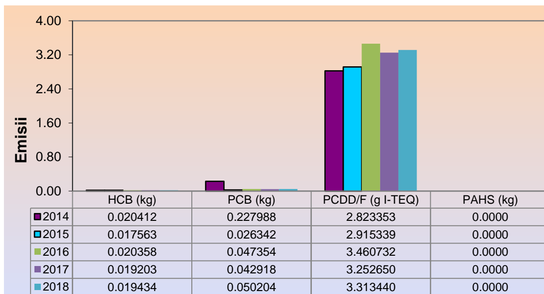
Fig. I.3.21. Evoluția emisiilor de poluanți organici persistenti din sectorul de activitate energie, în perioada 2014 – 2018
