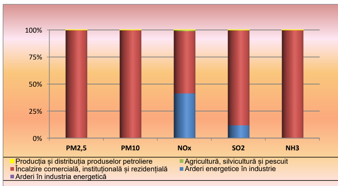
Fig. I.2.3. Pondere emisiilor de particule prim. și precursori secund. de particule pe sectoare de activitate din energie
