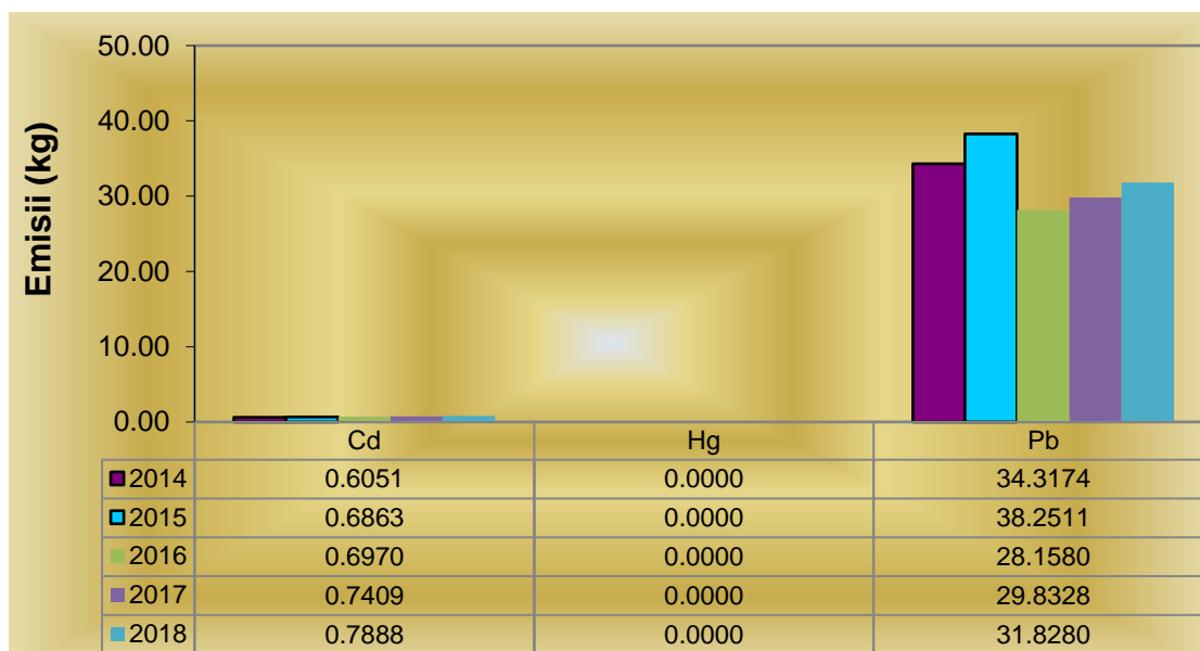
Fig. I.3.19. Evoluția emisiilor de metale grele din transport, în perioada 2014 – 2018
