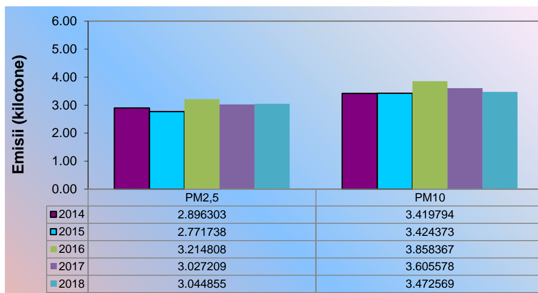
Fig. I.3.11. Evoluția emisiilor de particule primare, în perioada 2014 – 2018
