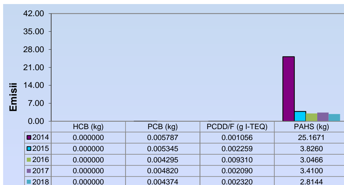
Fig. I.3.22. Evoluția emisiilor de poluanți organici persistenti din industrie, în perioada 2014 – 2018
