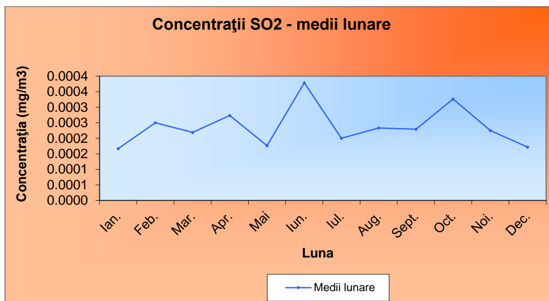
Fig. I.1.7. Concentrații de SO 2 – medii lunare
