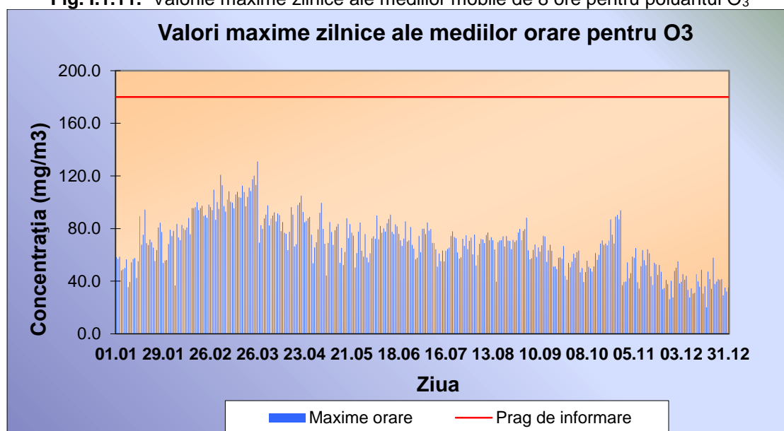
Fig. I.1.12. Valorile maxime zilnice ale mediilor orare pentru poluantul \text{O}_3
