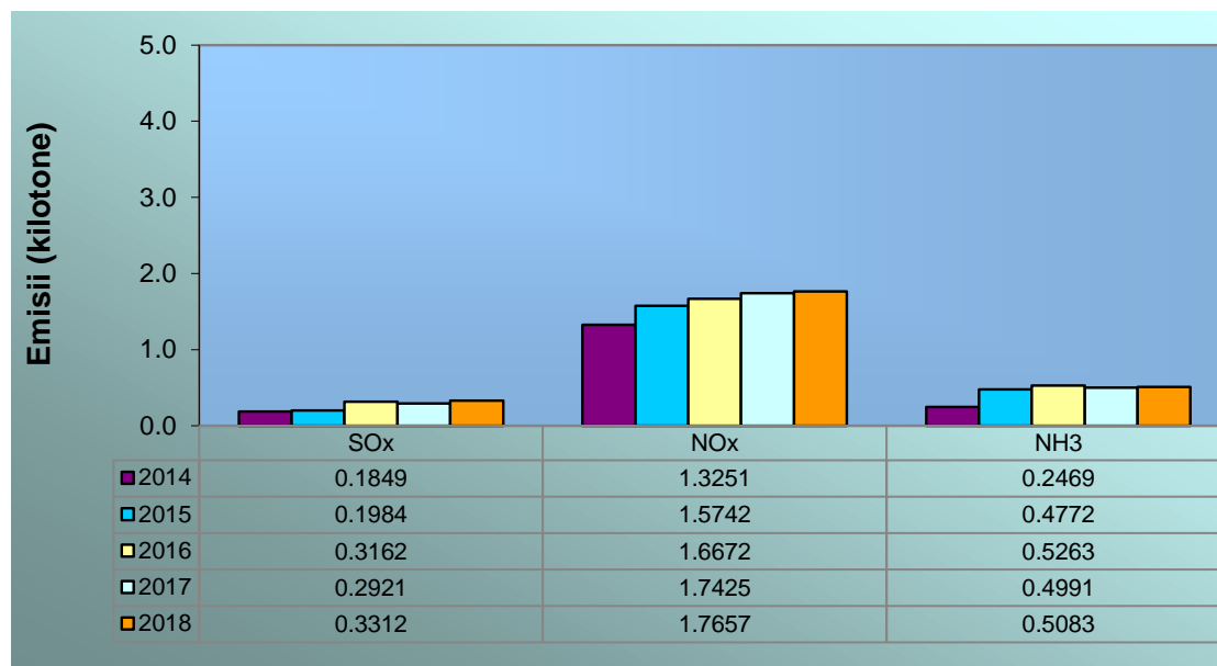
Fig. I.3.1. Evoluția emisiilor de substanțe acidifiante în perioada 2014 – 2018
