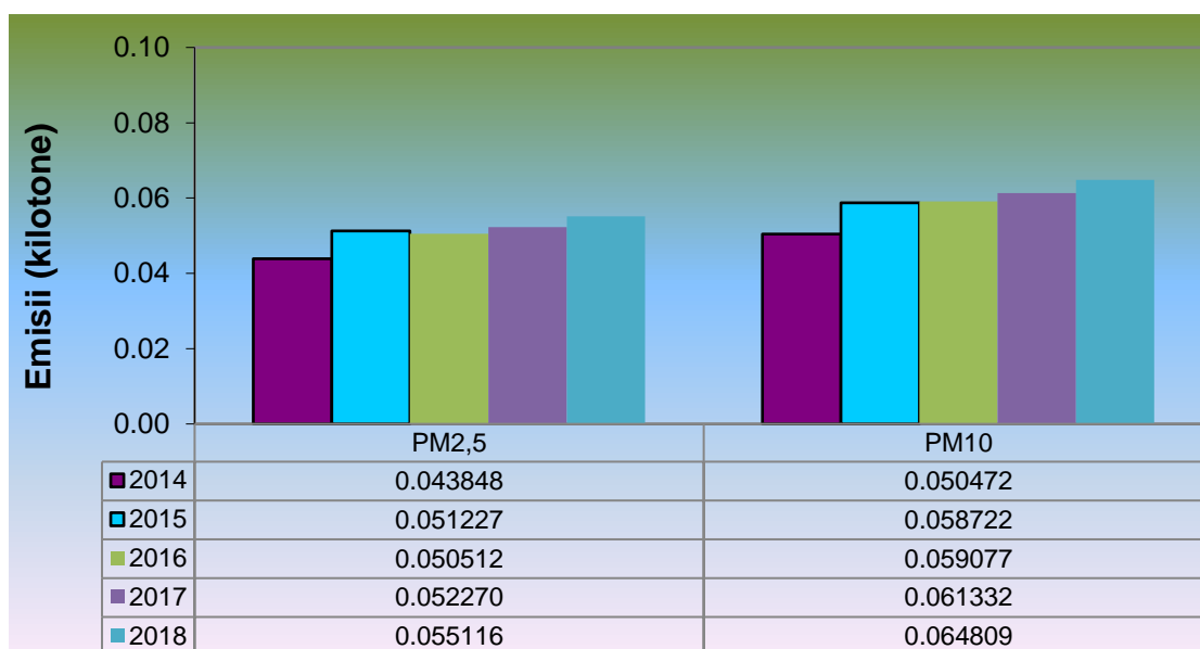
Fig. I.3.14. Evoluția emisiilor de particule primare din transporturi, în perioada 2014 – 2018
