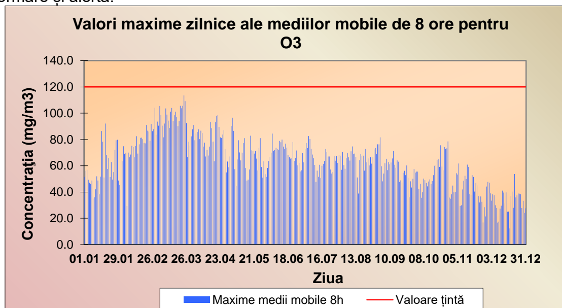
Fig. I.1.11. Valorile maxime zilnice ale mediilor mobile de 8 ore pentru poluantul \text{O}_3
