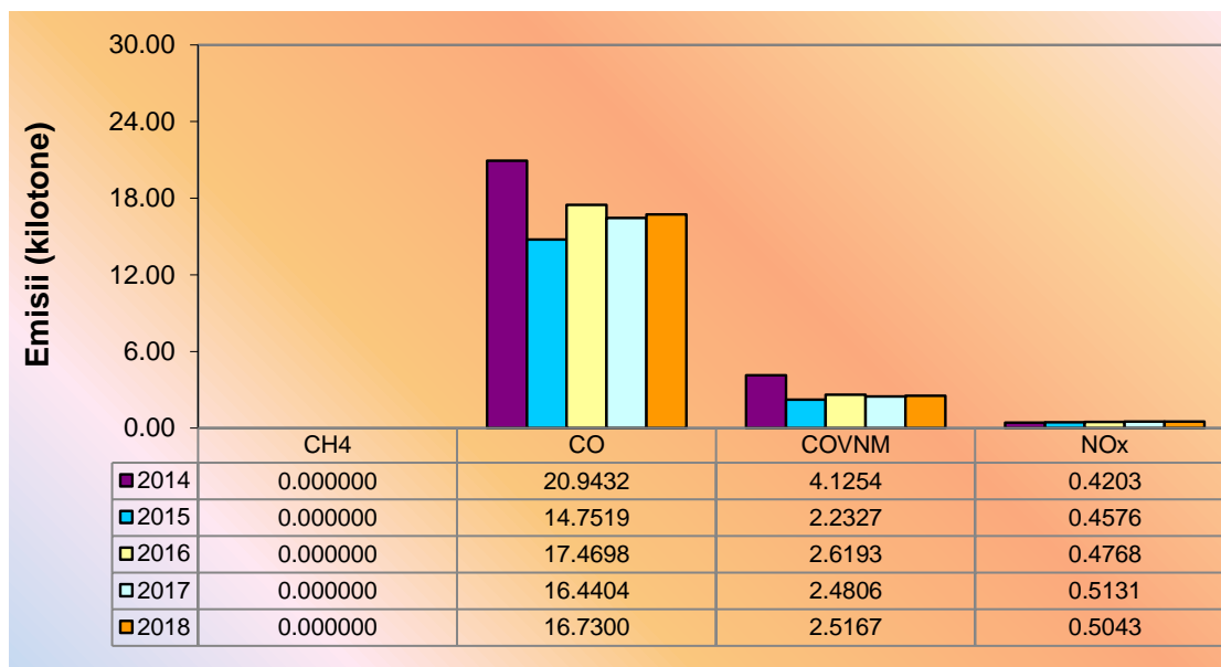
Fig. I.3.7. Evoluția emisiilor de precursori ai ozonului, din sectorul de activitate energie, în perioada 2014 – 2018
