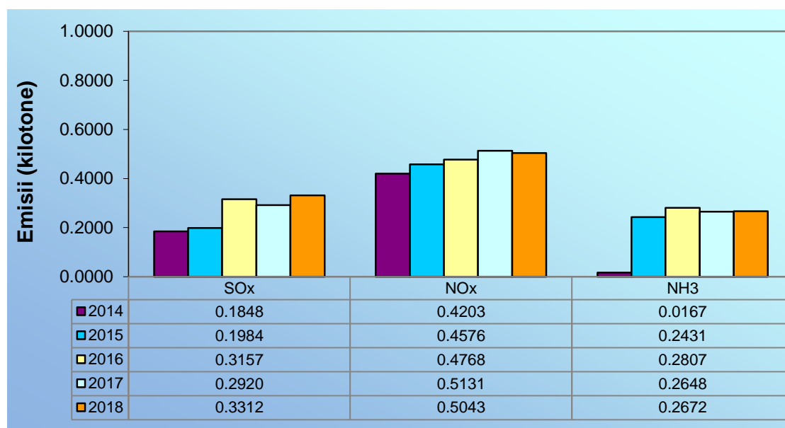
Fig. I.3.2. Evoluția emisiilor de substanțe acidifiante din sectorul de activitate energie, în perioada 2014 – 2018
