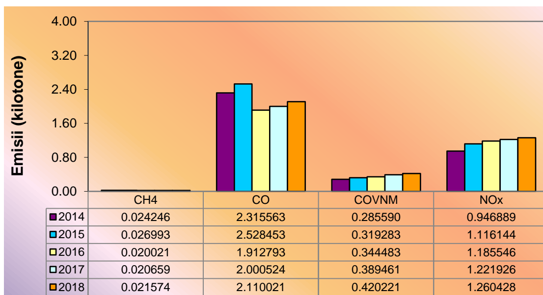
Fig. I.3.9. Evoluția emisiilor de precursori ai ozonului din transporturi, în perioada 2014 – 2018
