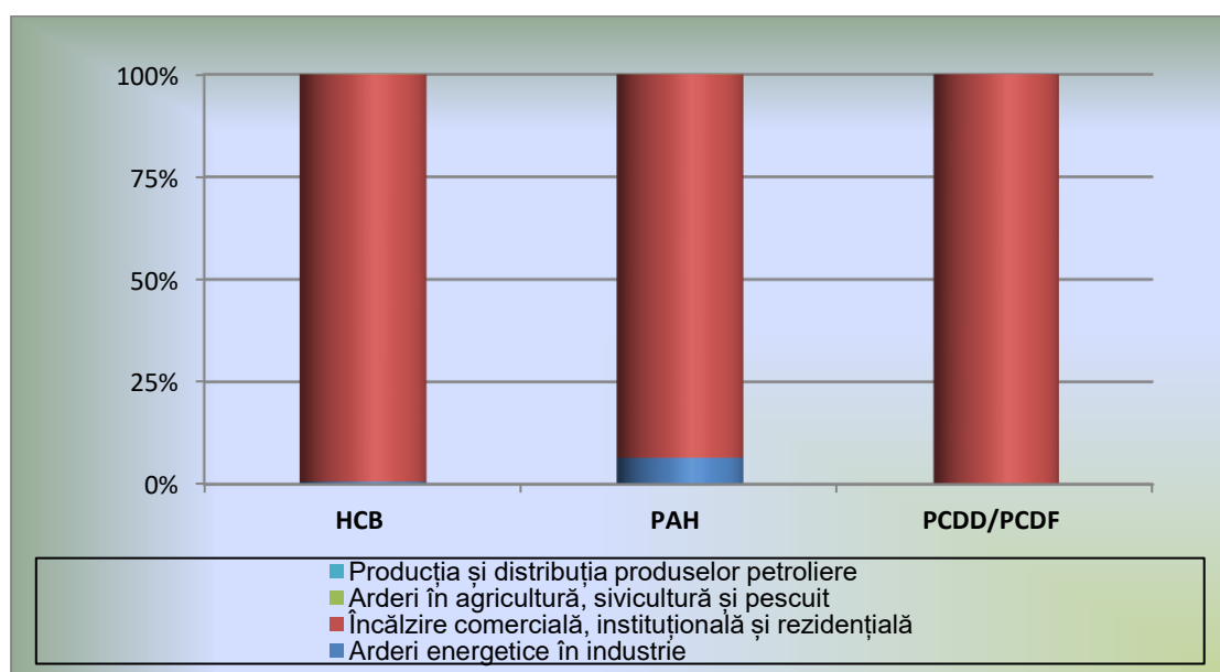
Fig. I.2.5. Ponderea emisiilor de poluanți organici persistenti pe sectoare de activitate din energie
