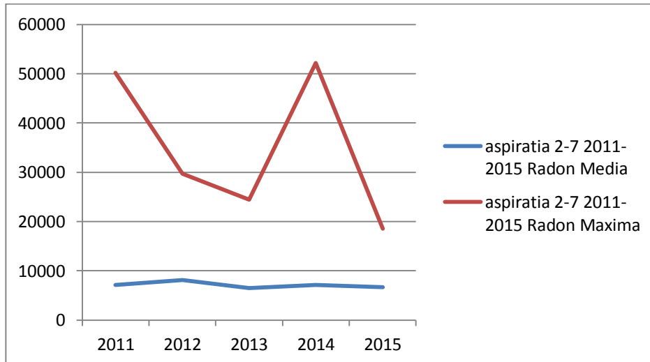
Figura IX.1.1.2.3- Variația radonului în atmosferă 2011-2015(02-07) Bq/mc
