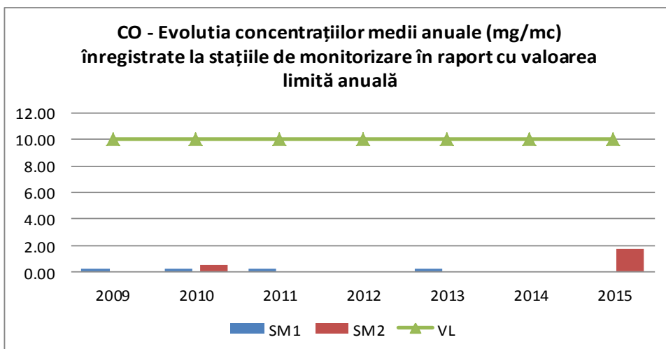
Fig. I.1.1.2.4. Evolutia concentrațiilor medii anuale înregistrate la stațiile de monitorizare în raport cu valoarea limită anuală pentru CO
