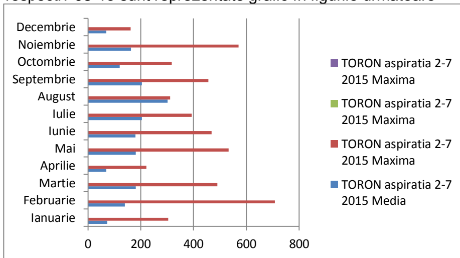
Figura IX.1.1.2.5- Variația toronului în atmosferă 2015 (02-07) Bq/mc
