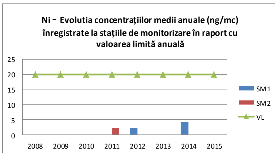
Fig. I.1.1.2.9. Evoluția concentrațiilor medii anuale înregistrate la stațiile de monitorizare în raport cu valoarea limită anuală Nichel
