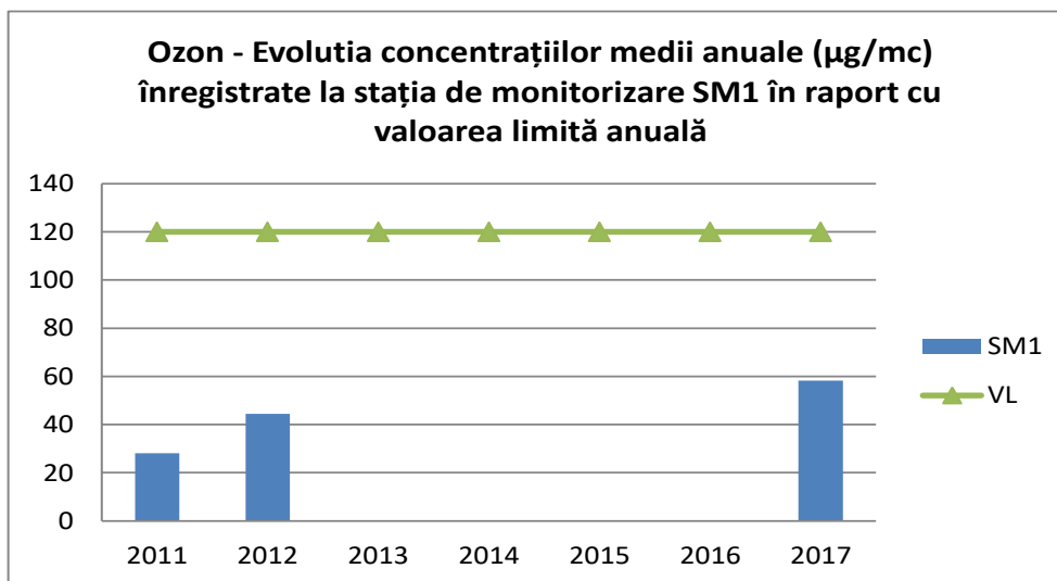
Fig. I.1.1.2.4. Evolutia concentrațiilor medii anuale înregistrate la stațiile de monitorizare în raport cu valoarea limită anuală pentru ozon
