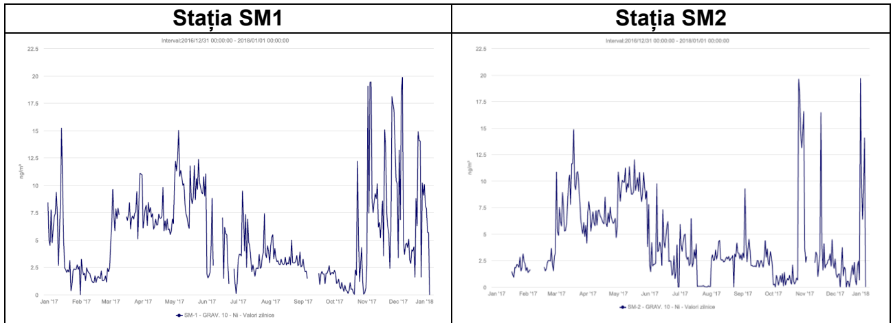
Figura I.1.1.1.15 Variația concentrației de nichel din pulberi în suspensie PM10 la stațiile SM1 și SM2
