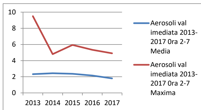
Figura IX.1.1.1.3- aerosoli atmosferici măsurarea imediată 2-7 (2013-2017) Bq/mc
