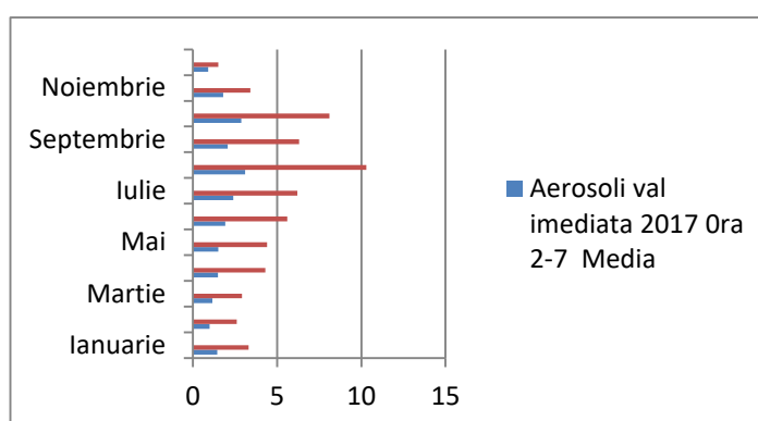
Figura IX.1.1.1.1- aerosoli măsuratori imediate 2017 ora 2-7 -Bq/mc
