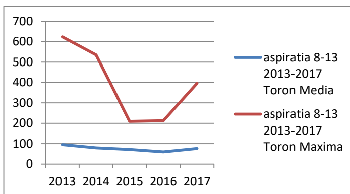
Figura IX.1.1.2.8- Variația toronului în atmosferă 2013-2017 (08-13) Bq/mc
