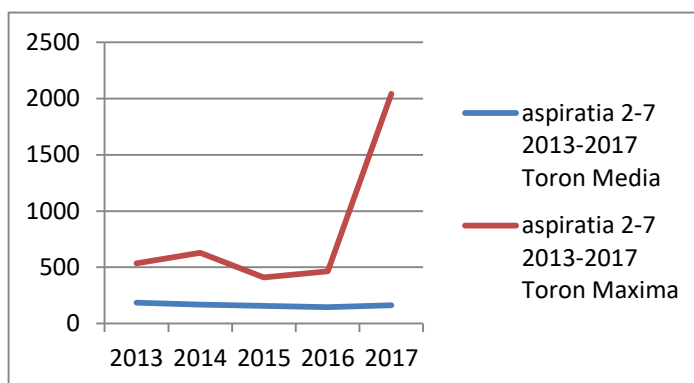
Figura IX.1.1.2.7- Variația toronului în atmosferă 2013-2017(02-07) Bq/mc
