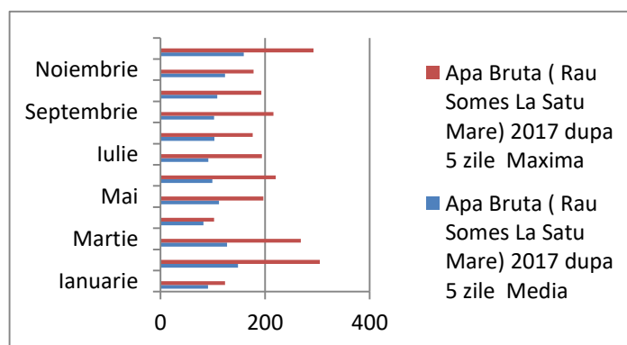
Figura IX.1.2.1.2 2017 Someș-la 5 zile Bq/l
