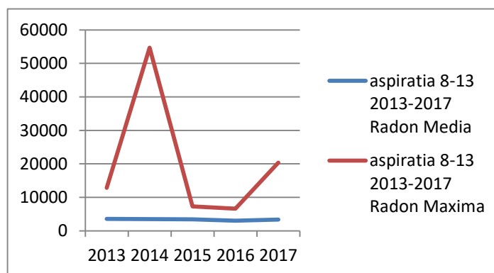
Figura IX.1.1.2.4- Variația radonului în atmosferă 2013-2017 (08-13) Bq/mc
