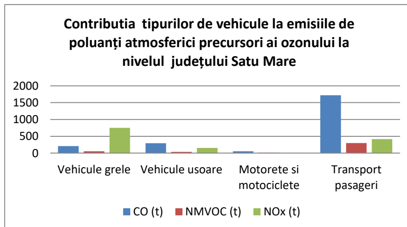
Fig. I.2.1.3.2. Contribuția tipurilor de vehicule la emisiile de poluanți atmosferici precursori ai ozonului la nivelul județului Satu Mare
