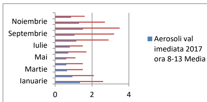
Figura IX.1.1.1.2- aerosoli măsuratori imediate 2017 ora 8-13-Bq/mc
