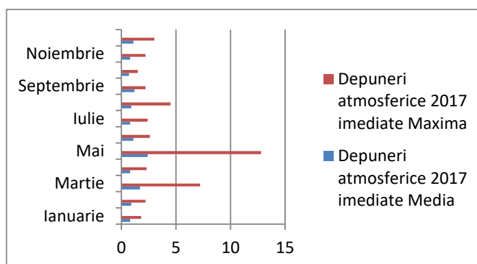
Figura IX.1.1.5.1 depuneri atmosferice imediate 2017 Bq/mp zi
