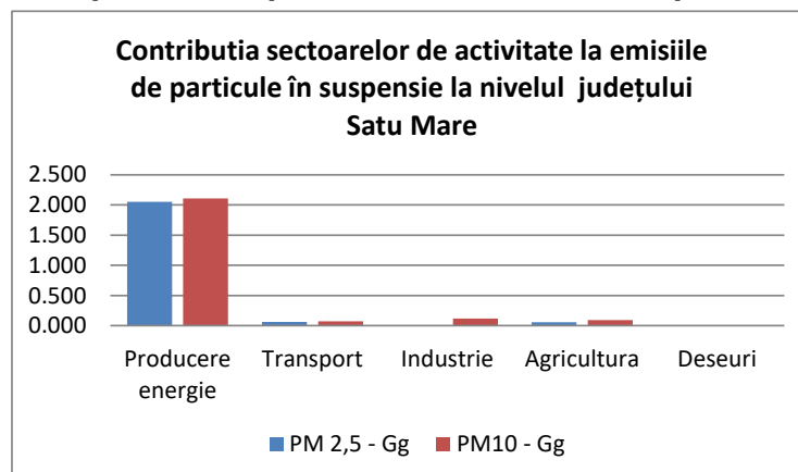
Fig. I.2.1.2.4. Contribuția sectoarelor de activitate la emisiile de particule în suspensie la nivelul județului Satu Mare
