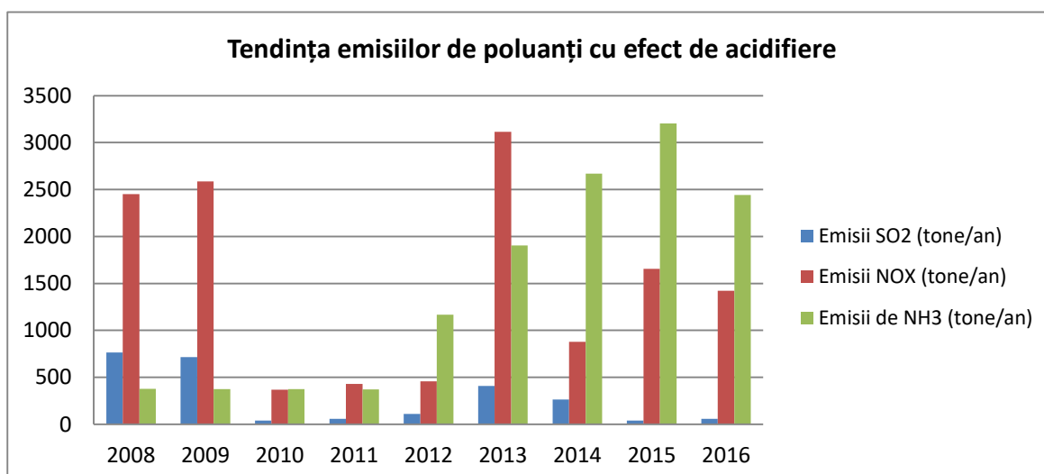
Fig.I.3.1.1. Tendința emisiilor de poluanți cu efect de acidifiere
