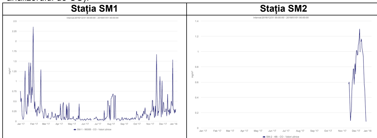
Figura I.1.1.1.8 Variația valorilor medii orare a concentrațiilor de CO prelevate prin stația automată SM1 și SM2
