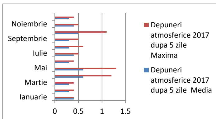
Figura IX.1.1.5.2 depuneri -5 zile 2017 Bq/mp zi
