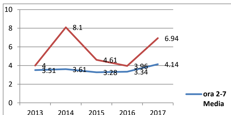
Figura IX.1.1.3.3 -Aerosoli, măsurare 5 zile interval orar 02-07 perioada 2013-2017 Bq/mc
