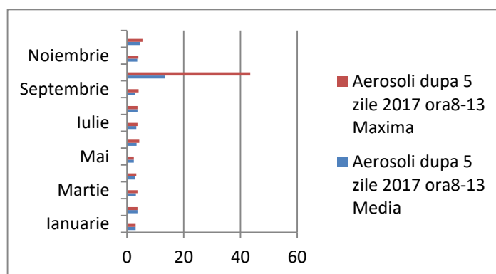
Figura IX.1.1.3.4 -Aerosoli, măsurare 5 zile interval orar 08-13 perioada 2013-2017 Bq/mc
