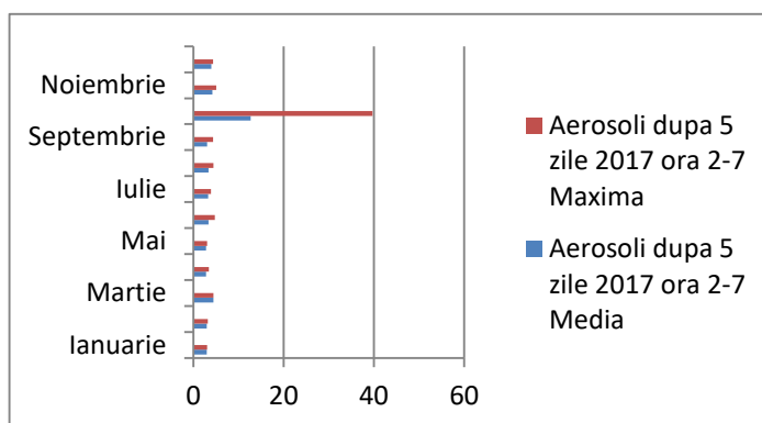
Figura IX.1.1.3.1- Aerosoli masurați la 5 zile interval orar 02-07 2017 Bq/mc
