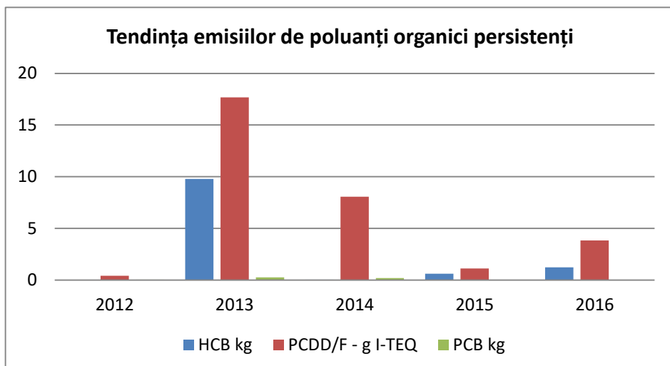
Fig.I.3.1.4. Tendința emisiilor de poluanți organici persistenti
