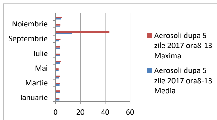
Figura IX.1.1.3.2- Aerosoli masuratori la 5 zile interval orar 08-13 2017 Bq/mc
