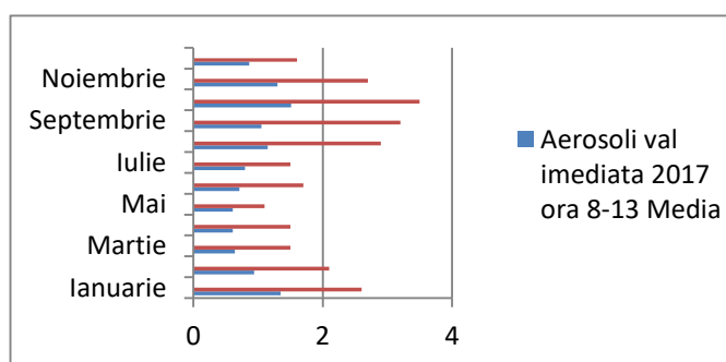
Figura IX.1.1.1.4 - aerosoli atmosferici măsurarea imediată 8-13 (2013-2017) Bq/mc
