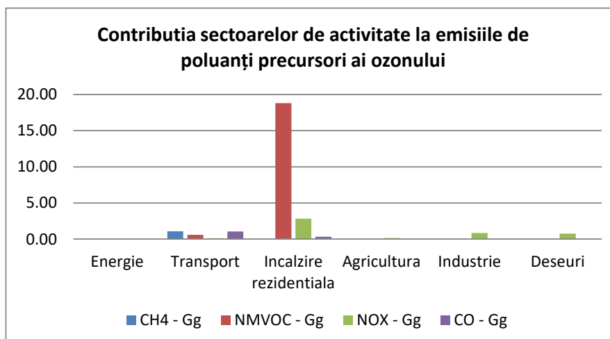
Fig. I.2.1.2.3. Contribuția sectoarelor de activitate la emisiile de poluanți precursori ai ozonului la nivelul județului Satu Mare
