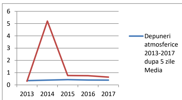
Figura IX.1.1.5.4 depuneri -5 zile 2013-2017 Bq/mp zi
