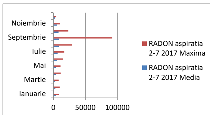
Figura IX.1.1.2.1- Variația radonului în atmosferă 2017 (02-07) Bq/mc
