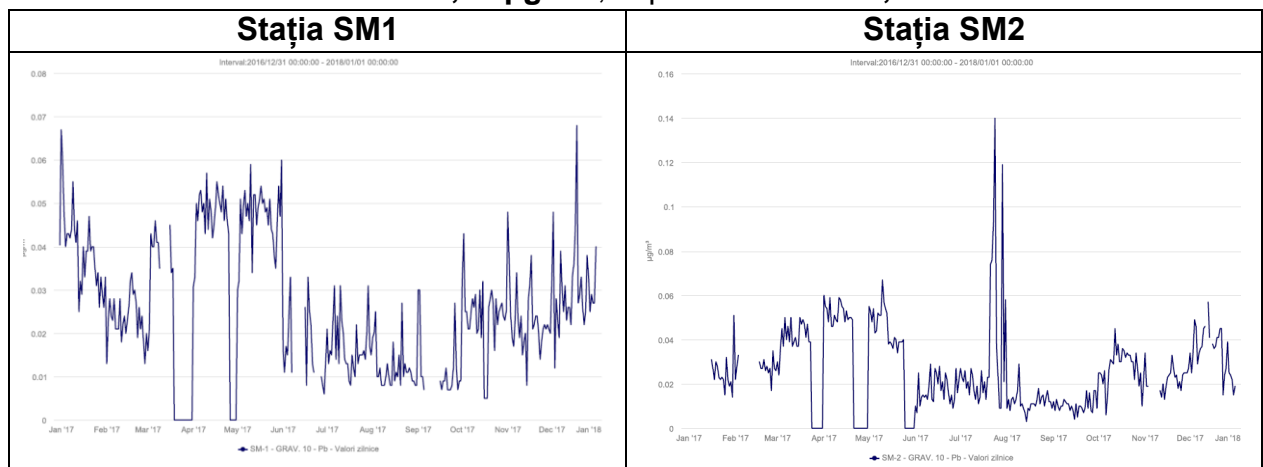
Figura I.1.1.1.13 Variația concentrației de plumb din pulberi în suspensie PM10 la stațiile SM1 și SM2
