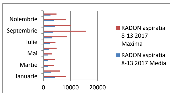
Figura IX.1.1.2.2- Variația radonului în atmosferă 2017 (08-13) Bq/mc
