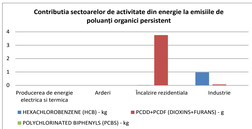
Fig. I.2.1.1.5. Contributia sectoarelor de activitate din energie la emisiile de poluanți organici persistent
