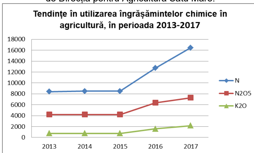
Fig. III.3.1.1. Tendințe în utilizarea îngrășămintelor chimice în agricultură în perioada 2013 - 2017
