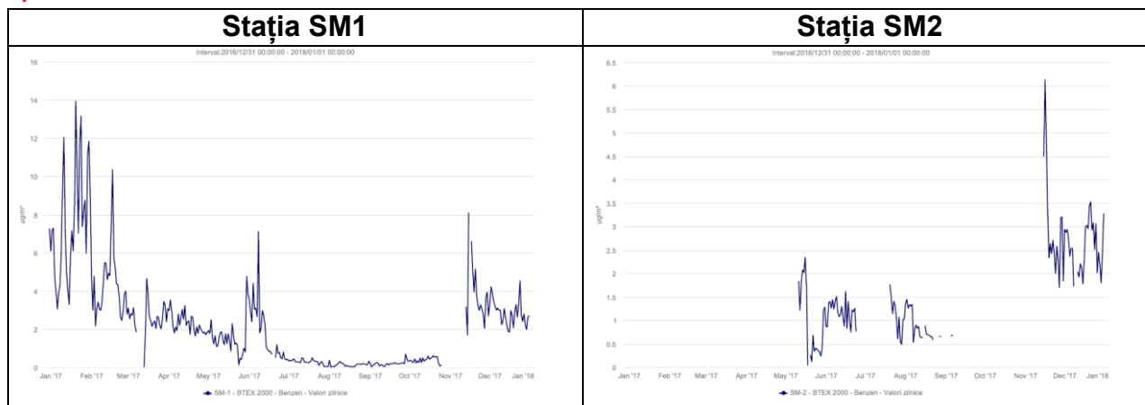
Figura I.1.1.1.9 Variația valorilor medii orare a concentrațiilor de benzen prelevate în stațiile SM1 și SM2
