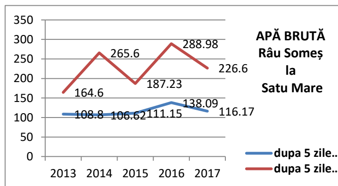
Figura IX.1.2.1.5 Apa brută măsurată la 5 zile 2013-2017 Bq/l
