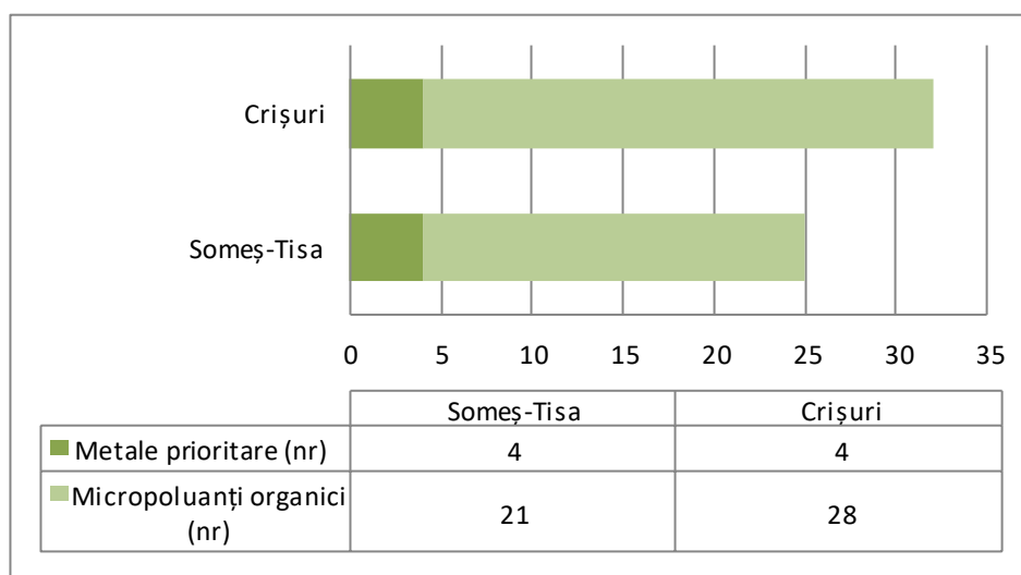
Figura II.2.1.1.2.1 Substanțe prioritare monitorizate în cursurile de apă pe spații /bazine hidrografice în anul 2017 (nr.) – mediul de investigație APĂ
