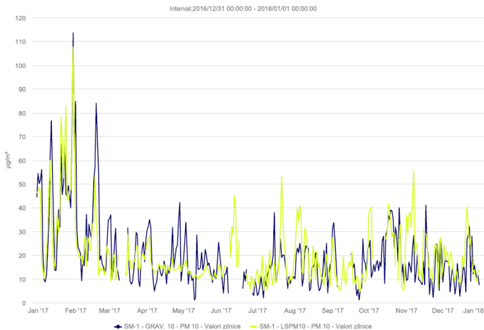
Figura I.1.1.1.11 Variația valorilor medii zilnice a concentrațiilor de pulberi în suspensie PM10 la stația SM1 determinate nefelometric și gravimetric
