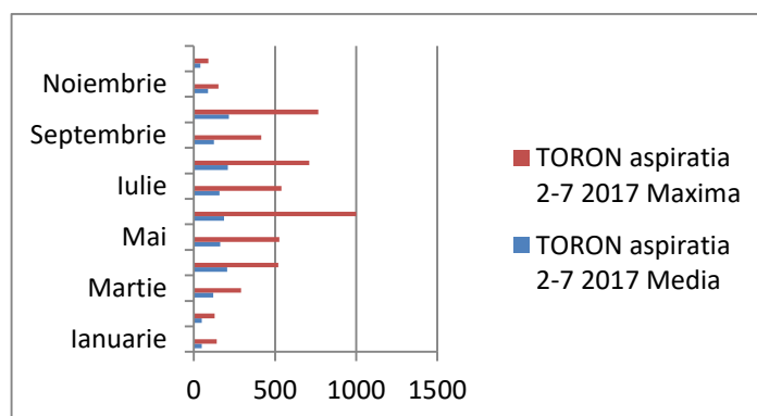
Figura IX.1.1.2.5- Variația toronului în atmosferă 2017 (02-07) Bq/mc
