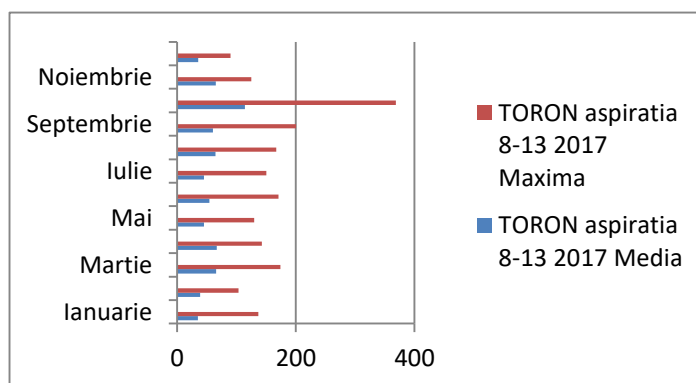
Figura IX.1.1.2.6- Variația toronului în atmosferă 2017 (08-13) Bq/mc
