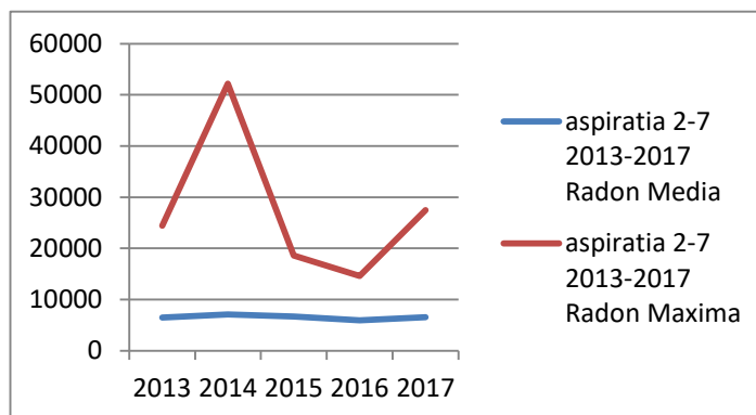
Figura IX.1.1.2.3- Variația radonului în atmosferă 2013-2017(02-07) Bq/mc
