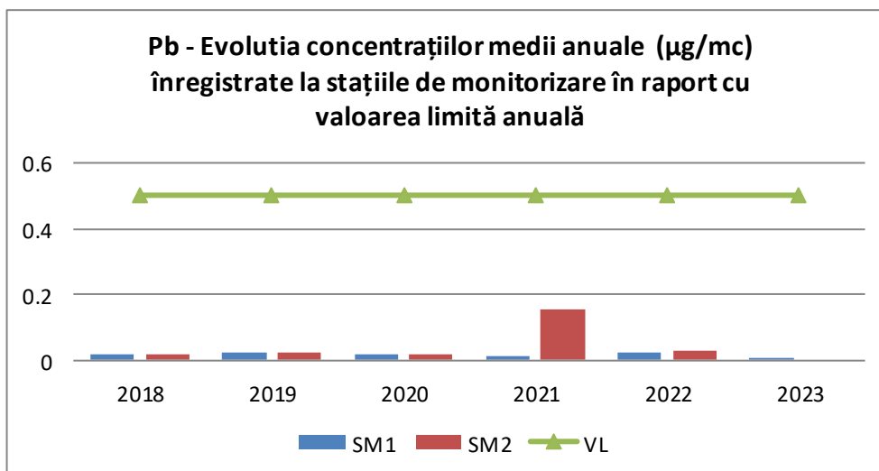
Fig. I.1.1.2.8. Evolutia concentrațiilor medii anuale înregistrate la stațiile de monitorizare în raport cu valoarea limită anuală pentru Pb
