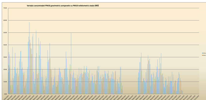
Fig.10. Variația valorilor medii zilnice a concentrațiilor de pulberi în suspensie PM10 la stația SM2 determinate nefelometric și gravimetric
