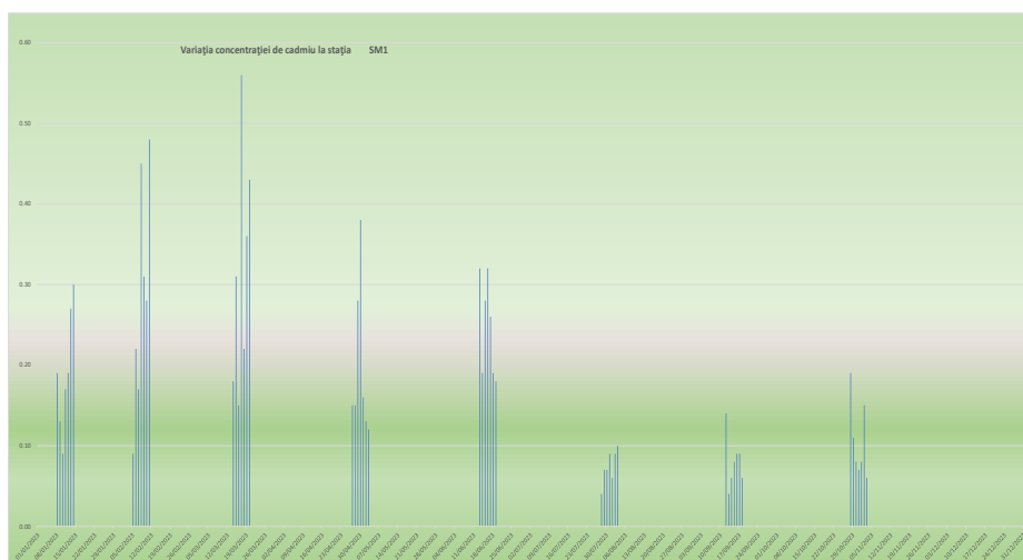
Fig. 12 Variația concentrației de cadmiu din pulberi în suspensie PM10 la stațiile SM1 și SM2 Tabel sinteză a poluanților determinați prin stațiile automate amplasate în județul Satu Mare
