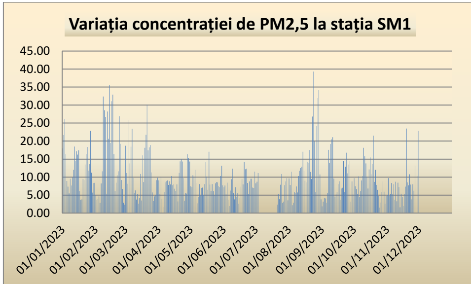
Fig. 8. Variația valorilor medii zilnice a concentrațiilor de pulberi în suspensie PM2,5 la stația SM1 determinate gravimetric
