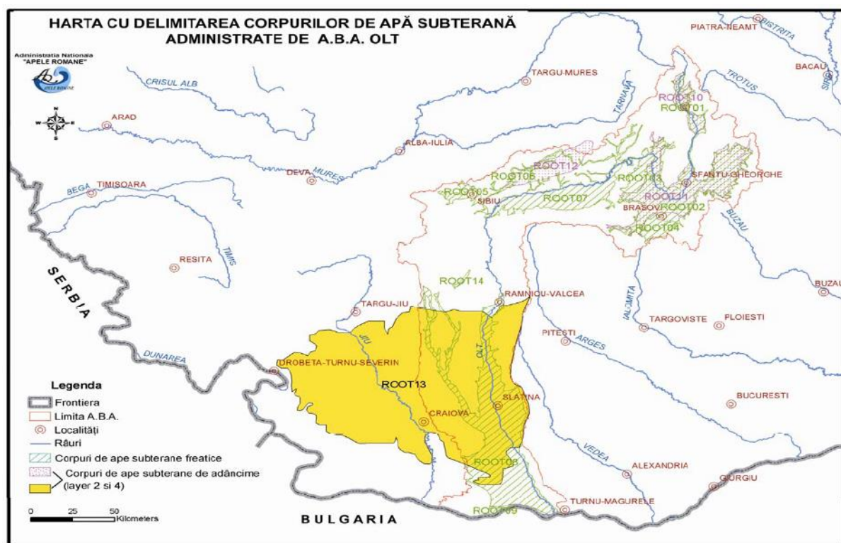
Figura 4: Delimitarea corpurilor de apă subterană administrate de ABA Olt
