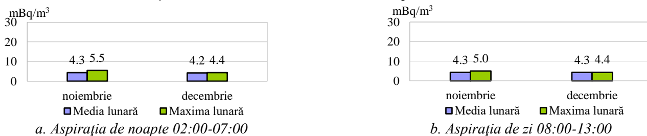
Fig. 2.2.3.1. Aerosoli atmosferici, activități specifice beta globale întârziate (la 5 zile) - valori medii și maxime în luna decembrie 2022, comparativ cu luna noiembrie 2022
