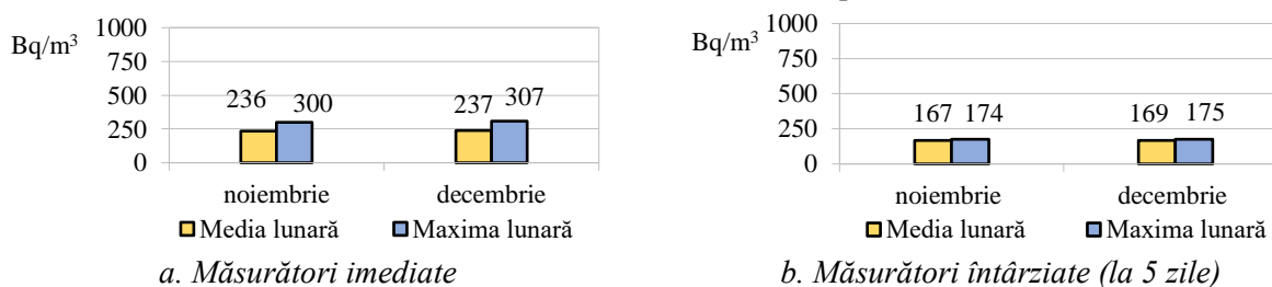
Fig. 2.4.1.1. Apă brută (râu Suceava - Burdujeni), activități specifice beta globale imediate și întârziate - medii lunare și maxime zilnice în luna decembrie 2022, comparativ cu luna noiembrie 2022
