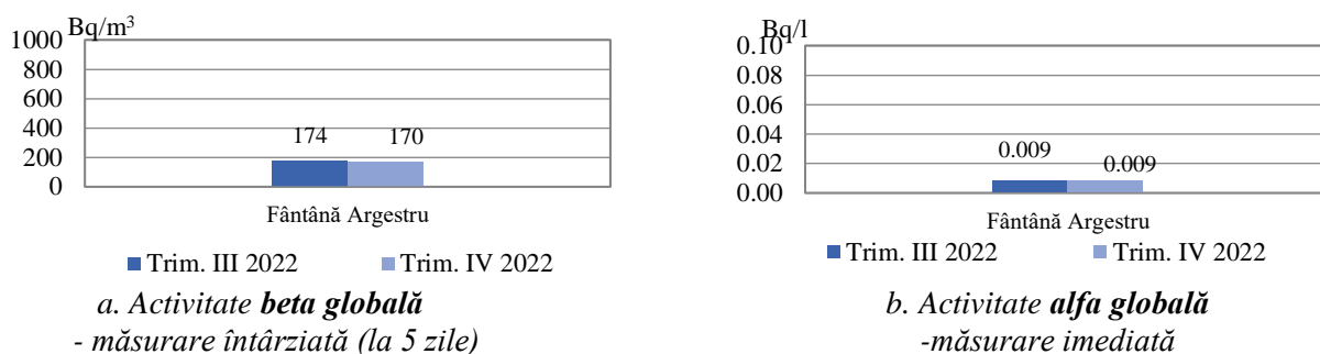
Fig. 2.4.2.2. Apă freatică – activități beta și alfa globale la proba prelevată în luna decembrie 2022
