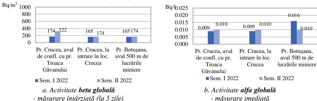
Fig. 2.4.2.1. Apă de suprafață – activități beta și alfa globale la probele prelevate în luna decembrie 2022
