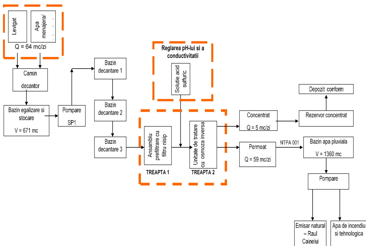
Diagramă 1 Flux ape uzate- levigat
