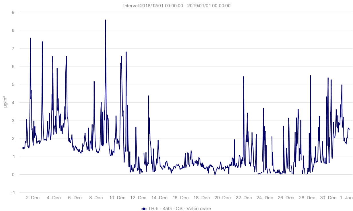
Fig. 1.5 – H 2 S(µg/m 3 ) – decembrie 2018
