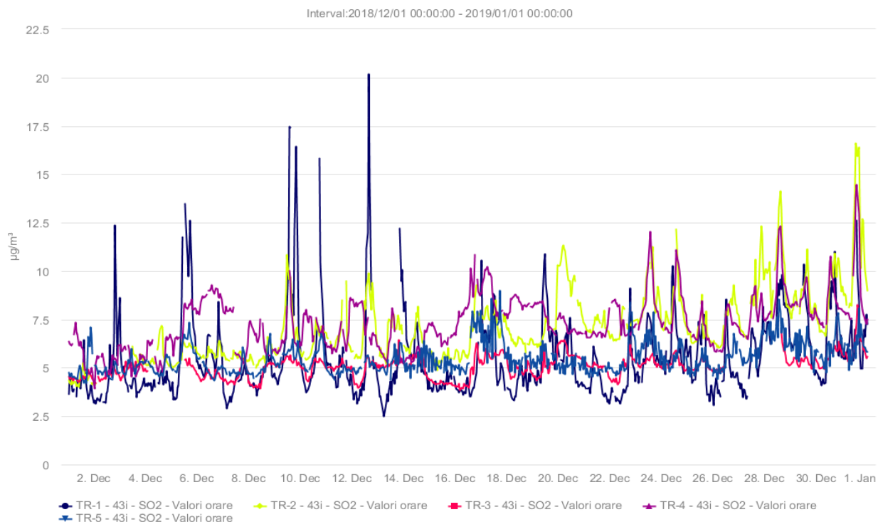
Fig. 1.1 - SO 2 (µg/m 3 ) - decembrie 2018
