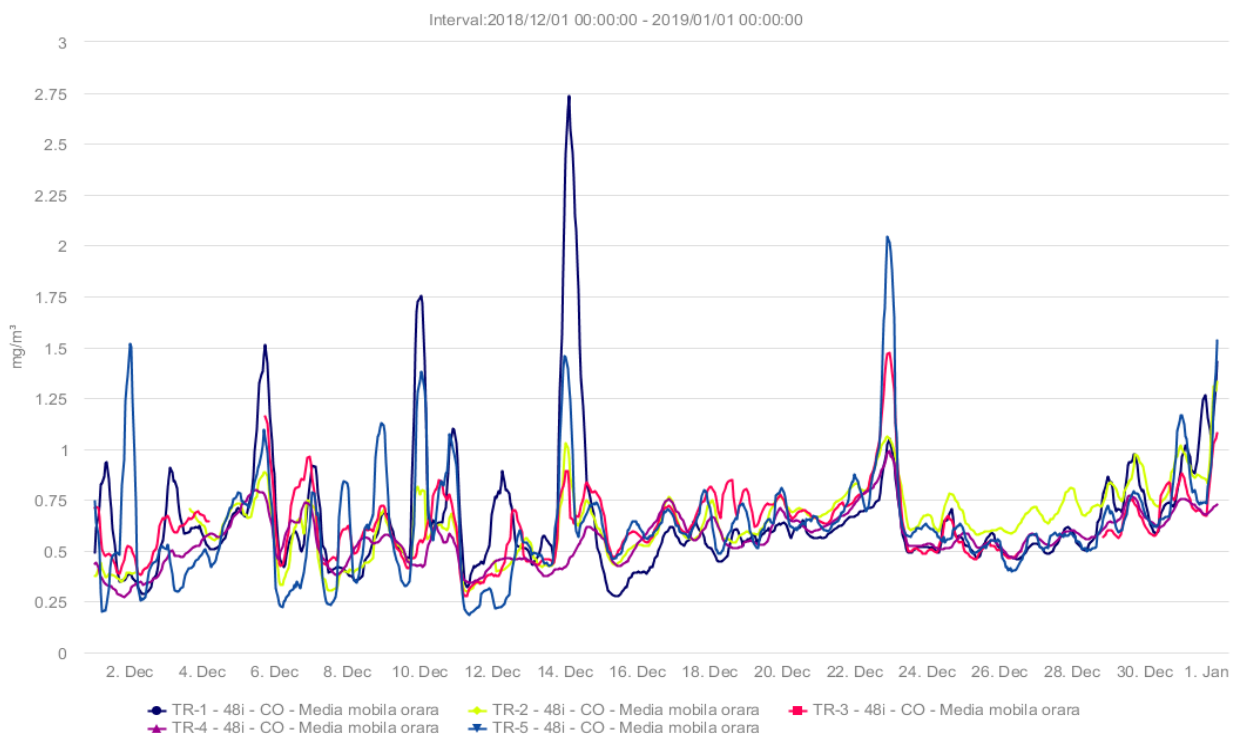
Fig. 1.4 - CO ( \text{mg}/\text{m}^3 ) - decembrie 2018
