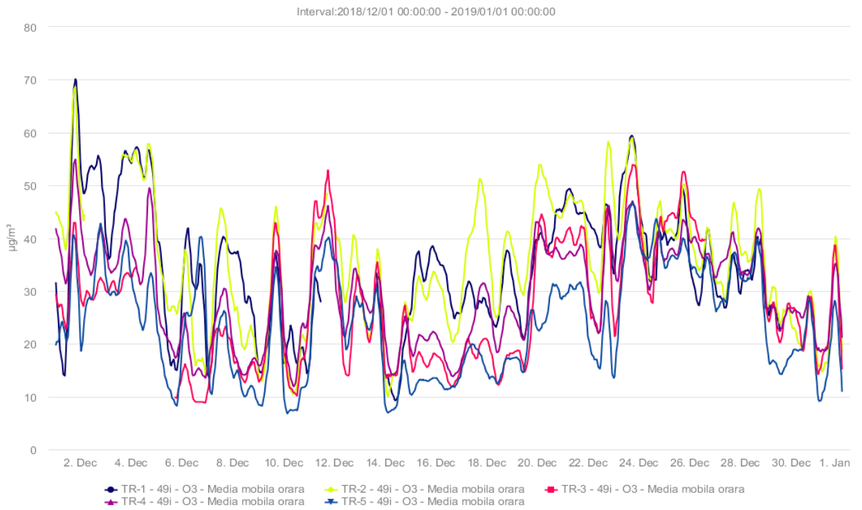
Fig. 1.3 - \text{O}_3 ( \mu\text{g}/\text{m}^3 ) – decembrie 2018
