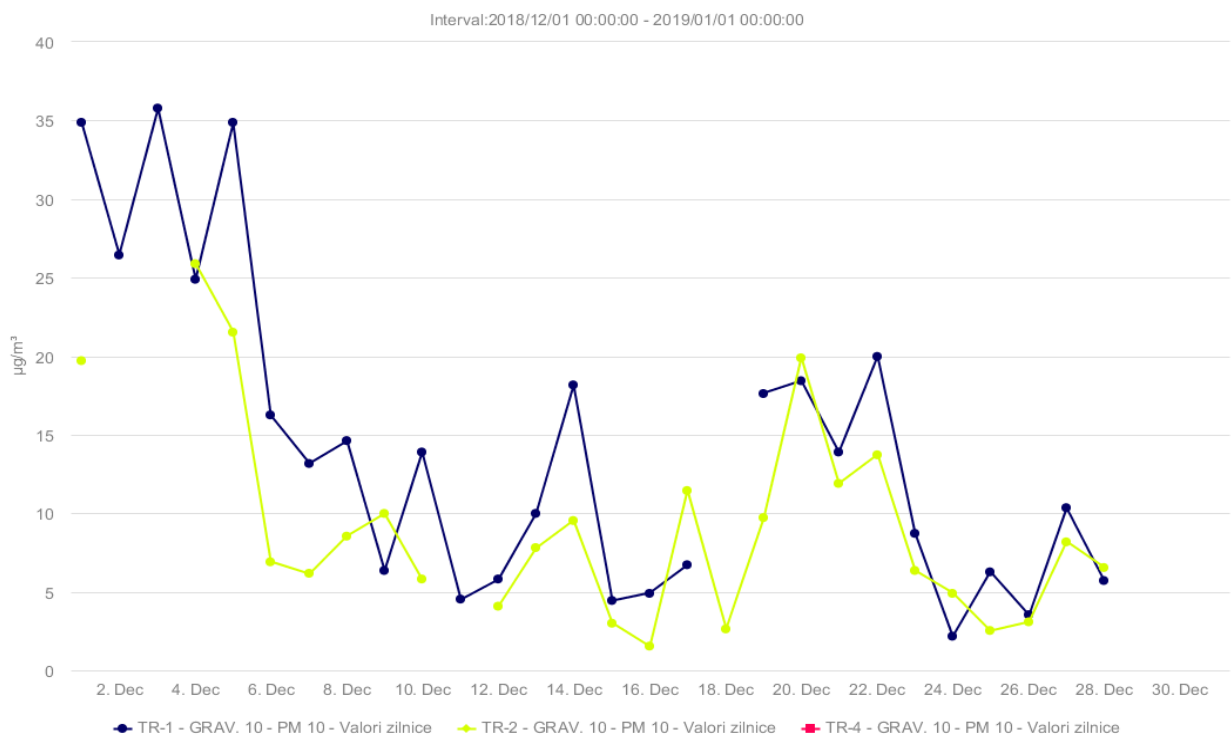
Fig. 1.6 – PM10 gravm. (µg/m 3 ) – decembrie 2018
