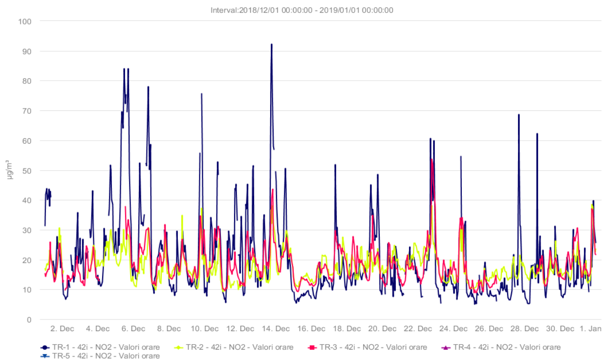
Fig. 1.2 - NO 2 (µg/m 3 ) - decembrie 2018
