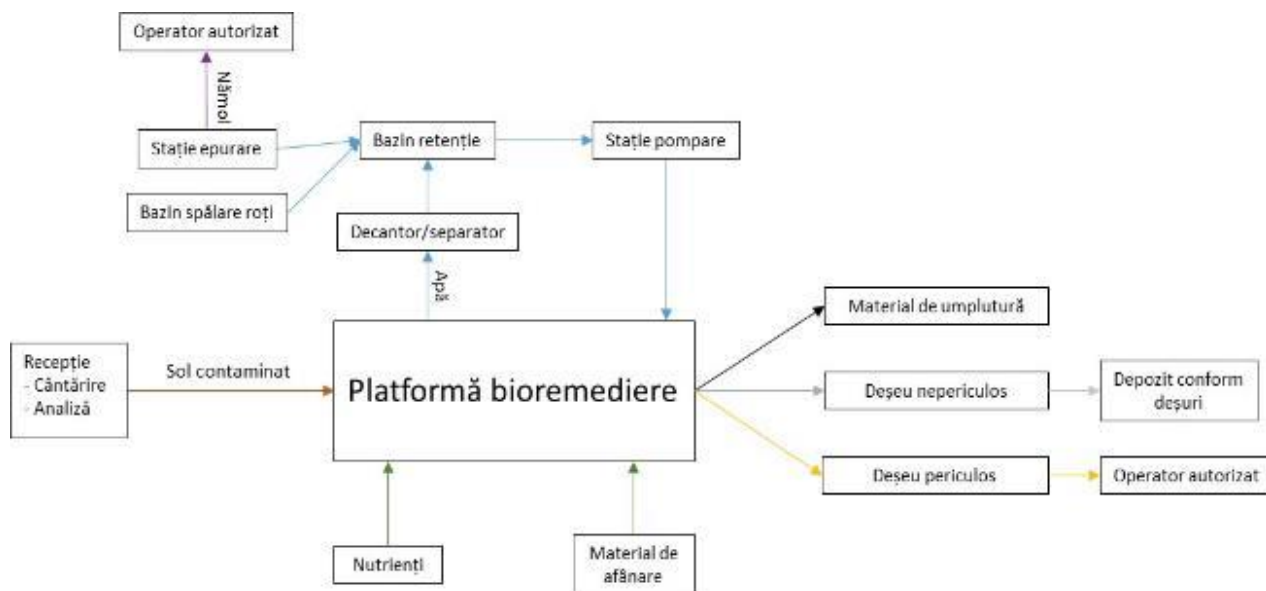
Figura 1.1. Schema noului sistem OMV Petrom de gestionare a deșeurilor
