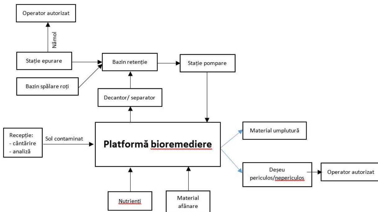
Figura 3.4.3. Diagrama Flux Tehnologic
