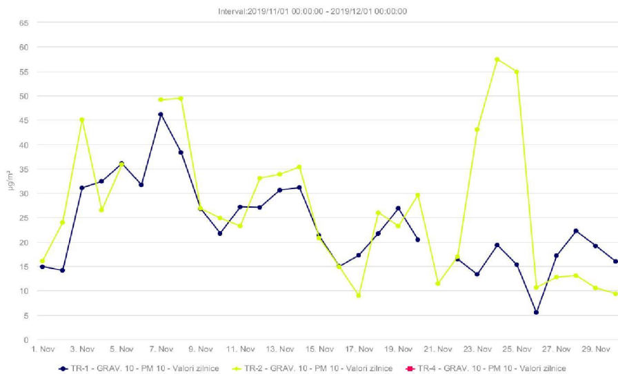
Fig. 1.8 – PM10 gravm. ( \mu\text{g}/\text{m}^3 ) – noiembrie 2019
