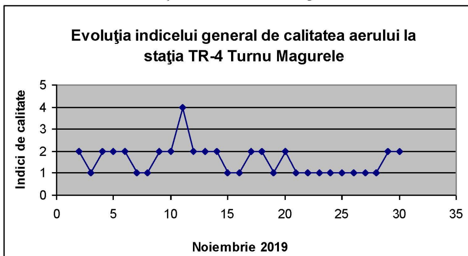
Fig 1.12 Evoluția indicelui general de calitate a aerului la stația TR-4 Turnu Măgurele
