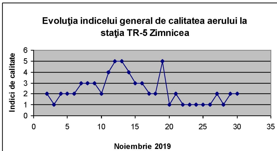
Fig 1.13 Evoluția indicelui general de calitate a aerului la stația TR-5 Zimnicea
