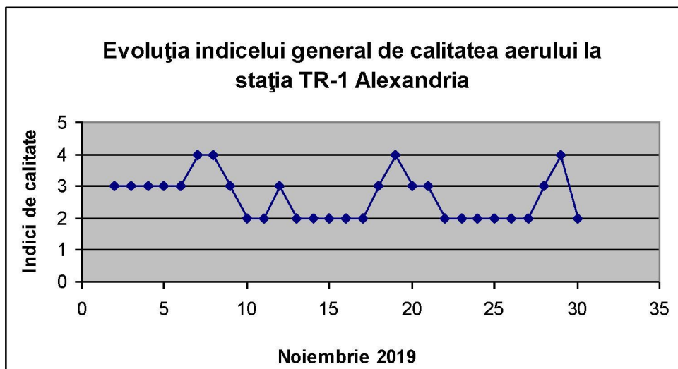
Fig 1.9 Evoluția indicelui general de calitate a aerului la stația TR-1 Alexandria
