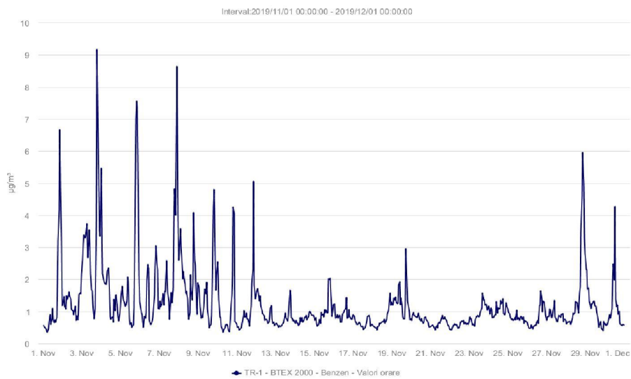
Fig. 1.5 – Benzen (µg/m 3 ) – noiembrie 2019
