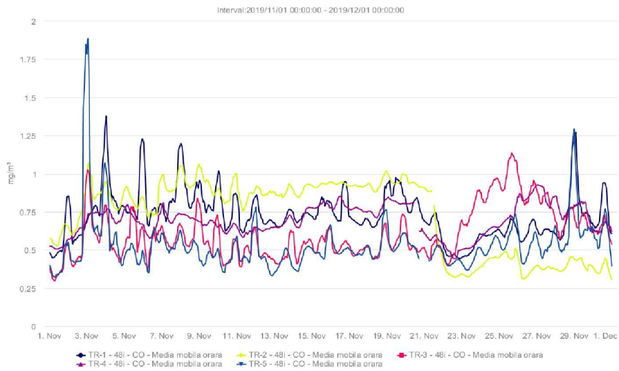
Fig. 1.4 - CO (mg/m 3 ) - noiembrie 2019
