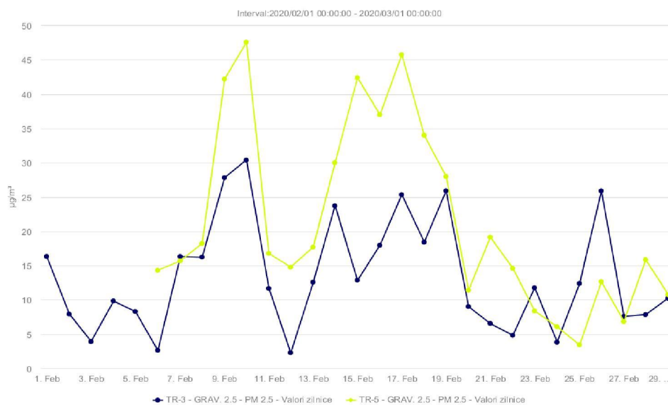
Fig. 1.9 – PM2.5 gravm. (µg/m 3 ) – februarie 2020
