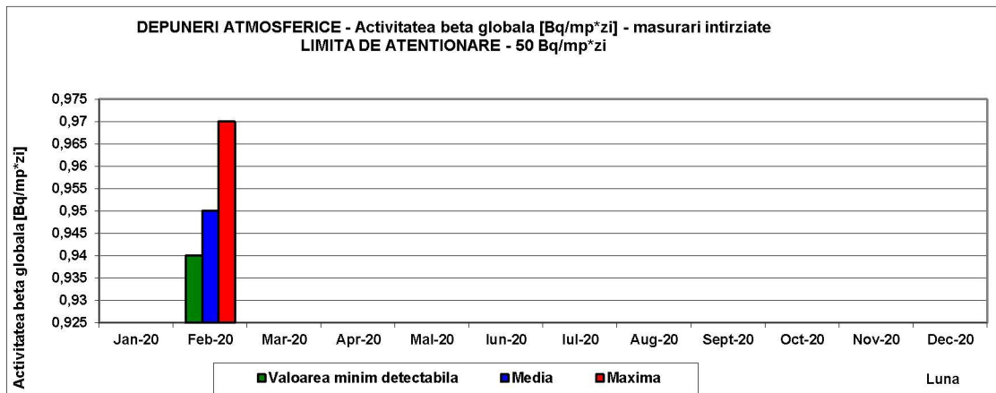
Fig.3.8 – Depuneri atmosferice – măș. intârziatē (5 zile) – Luna Februarie 2020
