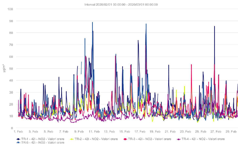
Fig. 1.2 - NO 2 ( \mu\text{g}/\text{m}^3 ) - februarie 2020
