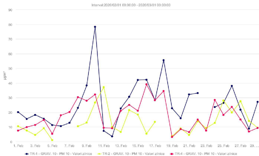
Fig. 1.8 – PM10 gravm. (µg/m 3 ) – februarie 2020
