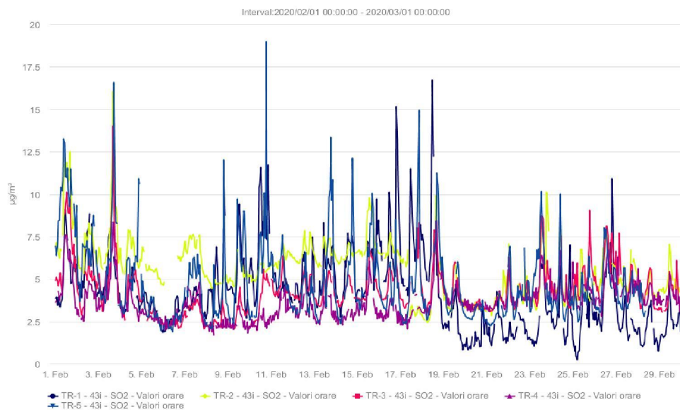
Fig. 1.1 - SO 2 ( \mu\text{g}/\text{m}^3 ) - februarie 2020
