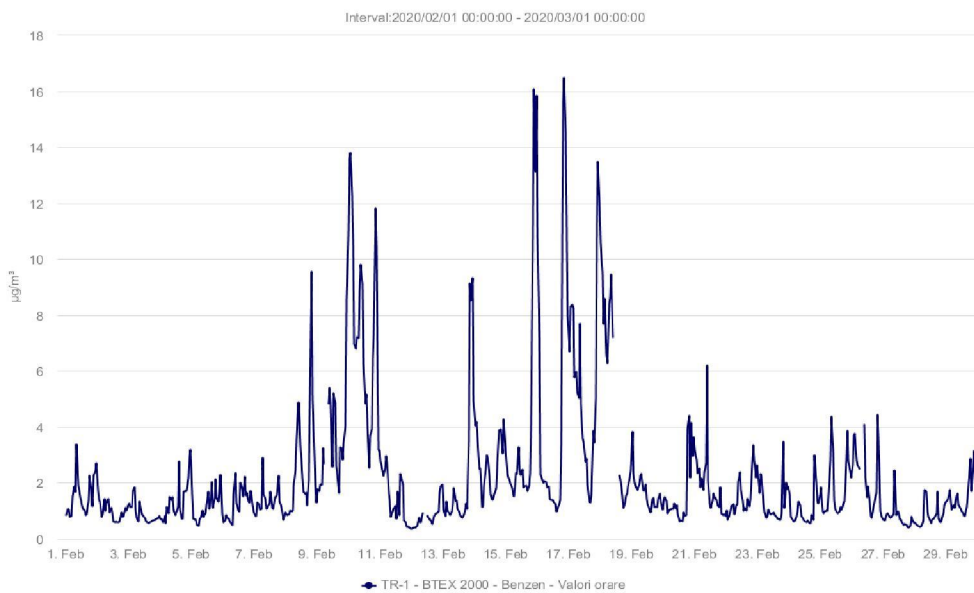
Fig. 1.5 – Benzen (µg/m 3 ) – februarie 2020
