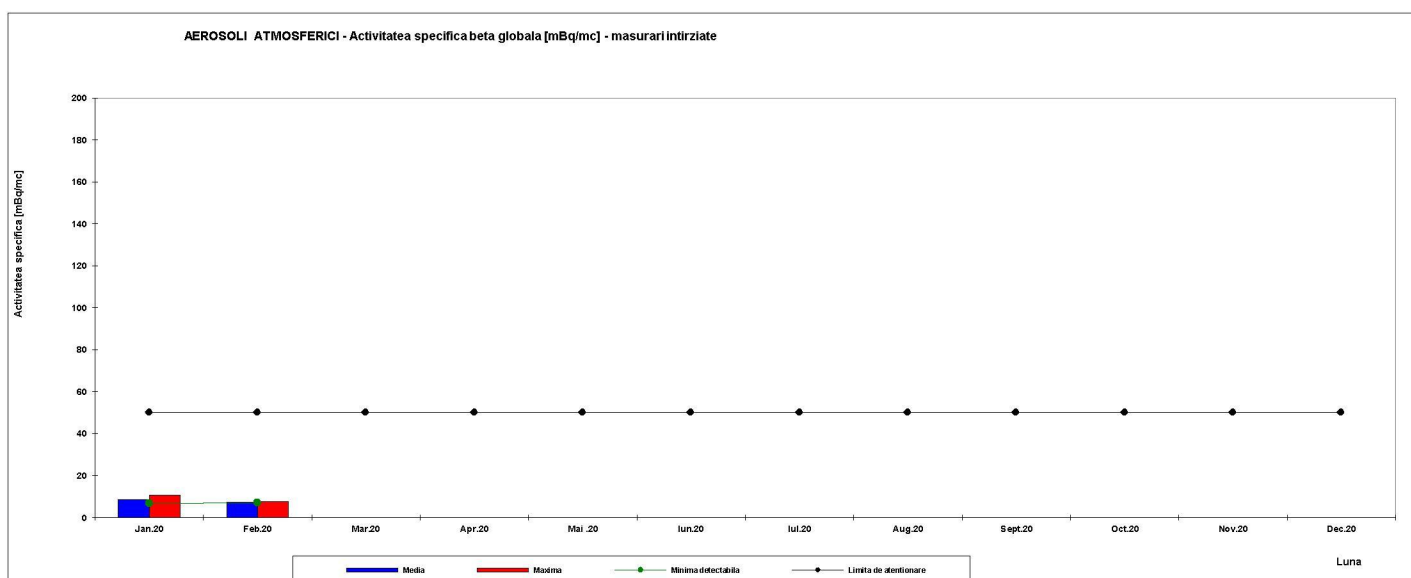
Fig.3.7 – Aerosoli atmosferici – măsurări întârziate (5 zile) – Luna Februarie 2020
