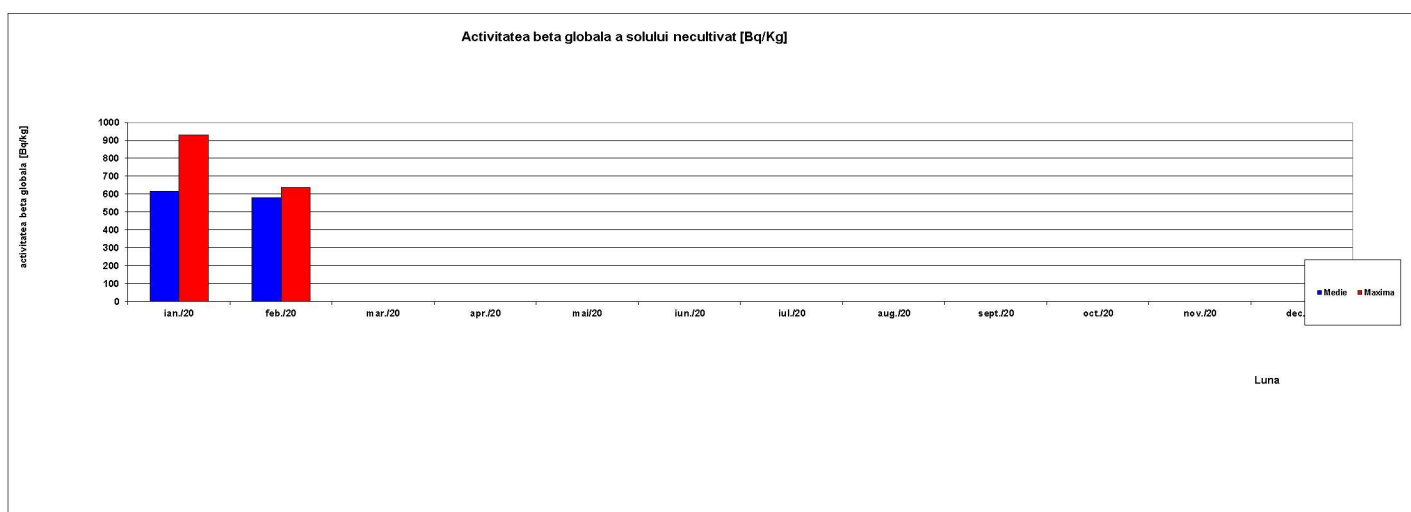
Fig.3.6 – Sol necultivat – măsurări întârziate (5 zile) – Luna Februarie 2020
