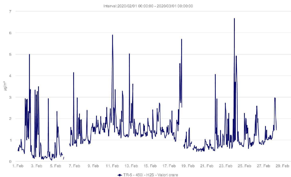
Fig. 1.6 – H 2 S (µg/m 3 ) – februarie 2020
