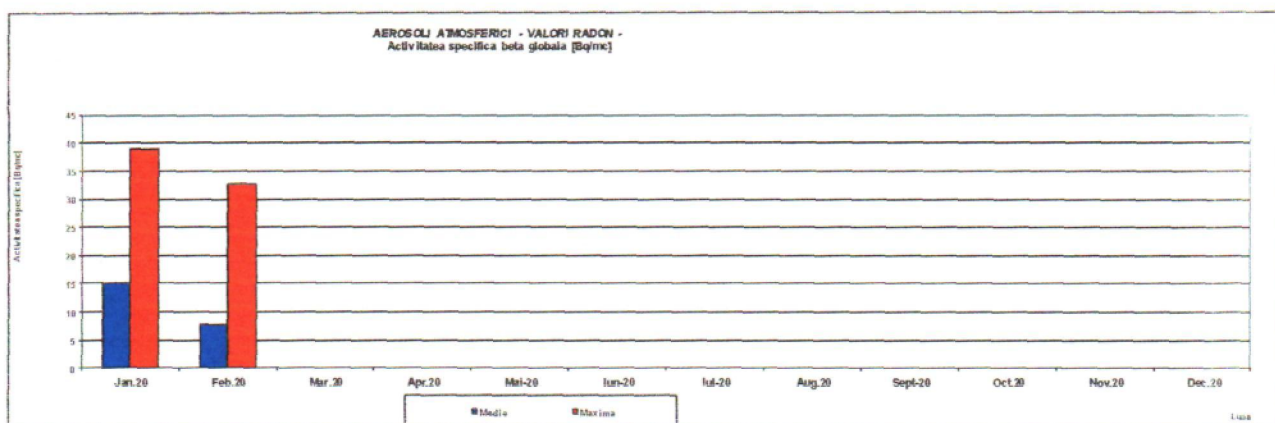
Fig.3.11 – Aerosoli atmosferici – Activitatea beta globală Radon – Luna Februarie 2020
