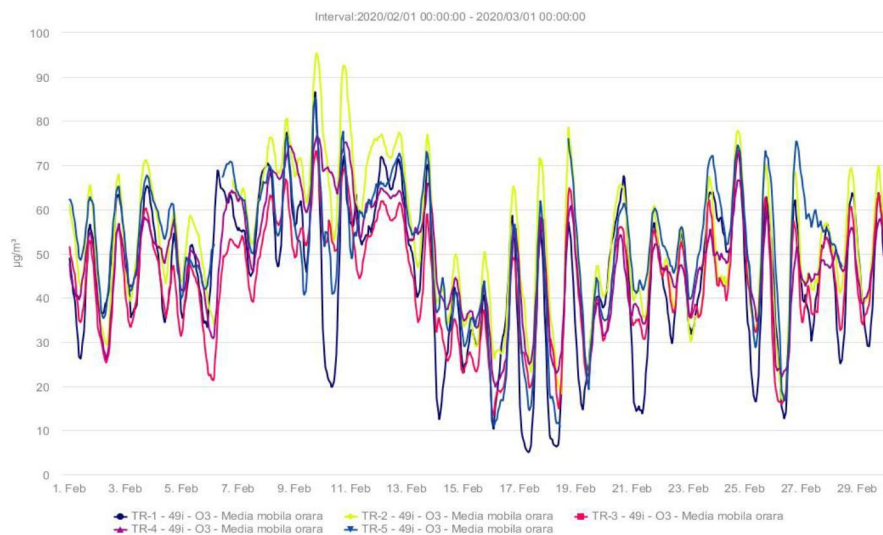
Fig. 1.3 - O 3 ( \mu\text{g}/\text{m}^3 ) - februarie 2020
