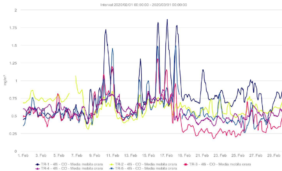
Fig. 1.4 - CO (mg/m 3 ) - februarie 2020
