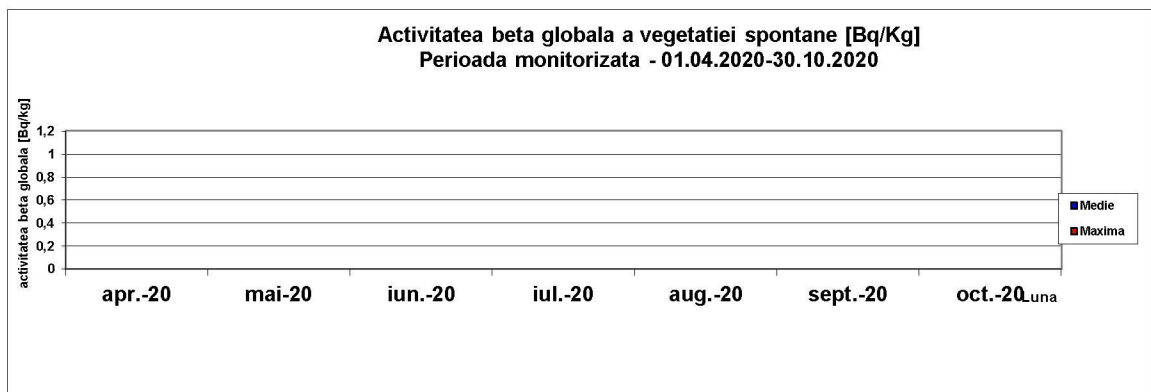
Fig.3.9 – Vegetatie spontana – activitatea beta globala – perioada: Aprilie - Octombrie
