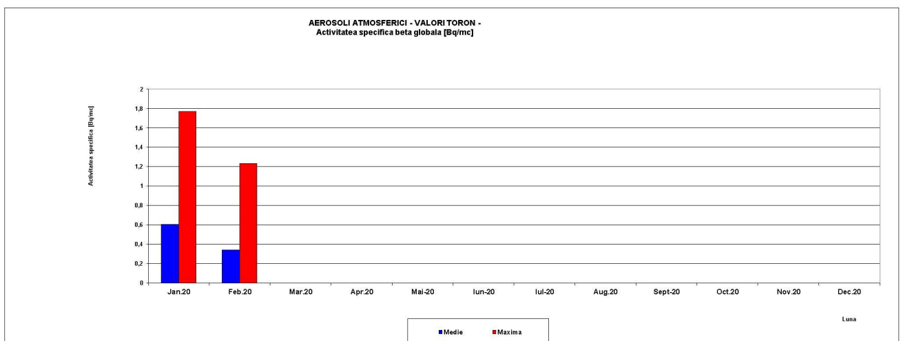
Fig.3.10 – Aerosoli atmosferici – Activitatea beta globală Toron – Luna Februarie 2020
