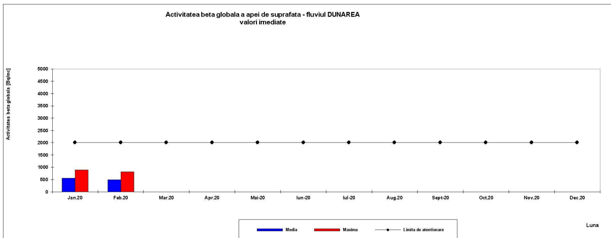
Fig.3.5 – Apa de suprafată (Dunăre) – măsurări imediate – Luna Februarie 2020
