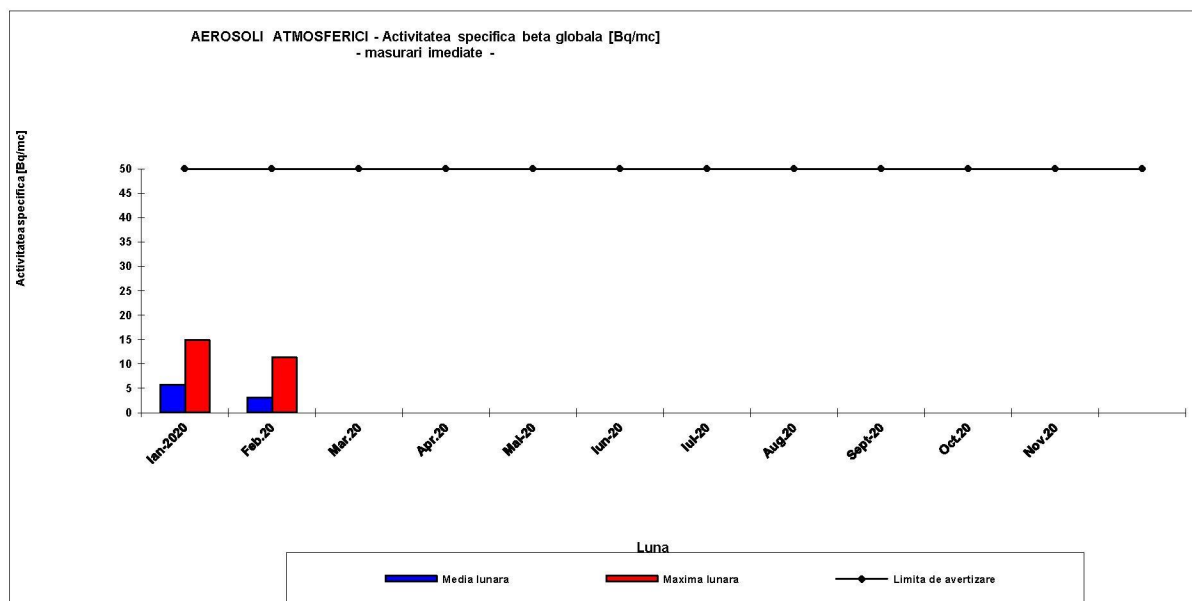
Fig.3.3 – Aerosoli atmosferici – măsurări imediate – Luna Februarie 2020
