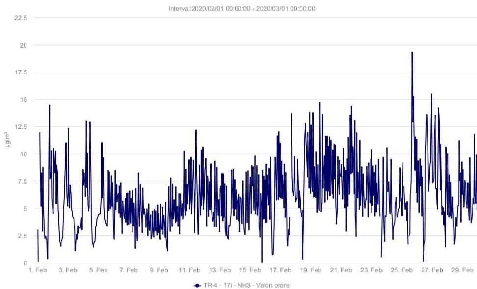
Fig. 1.7 – NH 3 (µg/m 3 ) – februarie 2020
