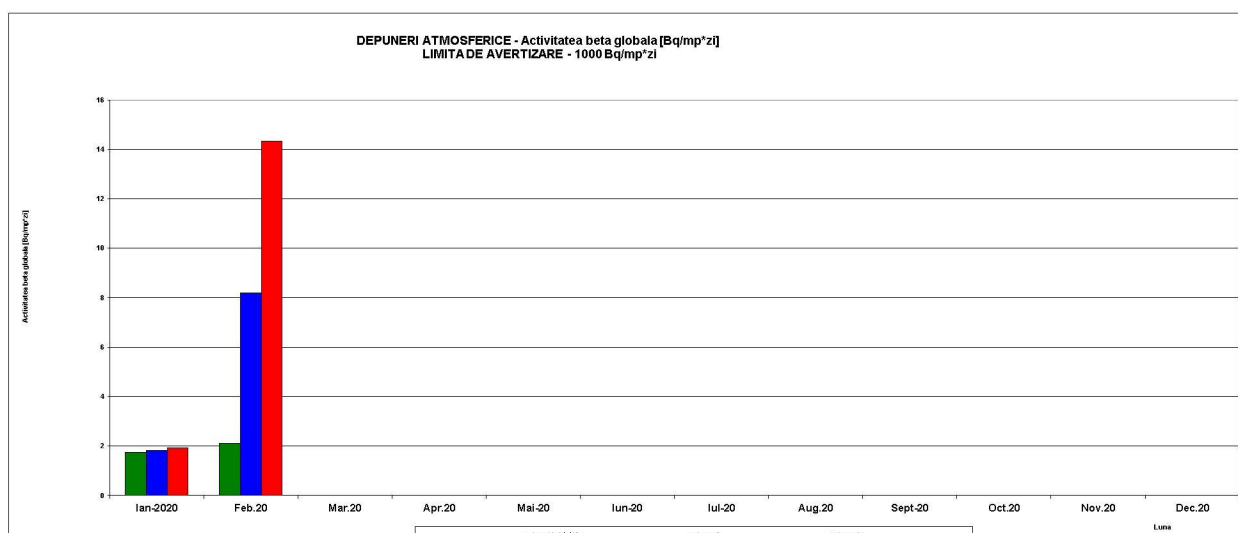
Fig.3.4 – Depuneri atmosferice – măsurări imediate – Luna Februarie 2020
