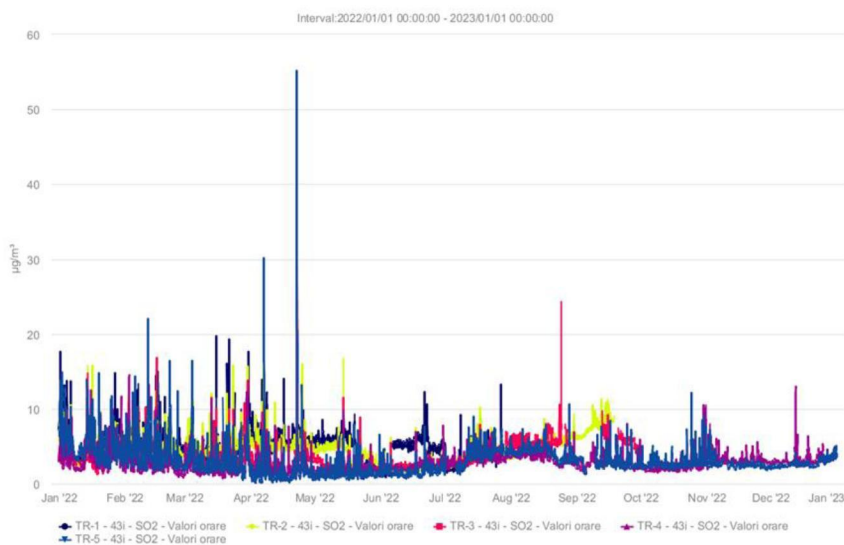
Fig. 1 Evoluția SO 2 în anul 2022 (concentrații medii orare)
