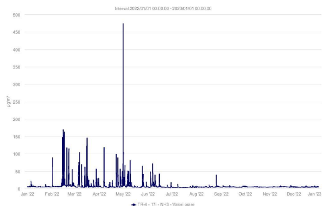
Fig. 6 Evoluția NH 3 în anul 2022 (concentrații medii orare)
