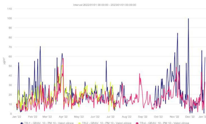
Fig. 7 Evoluția PM10 în anul 2022 (concentrații medii zilnice)
