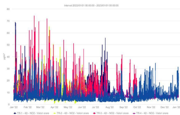
Fig. 2 Evoluția NO 2 în anul 2022 (concentrații medii orare)
