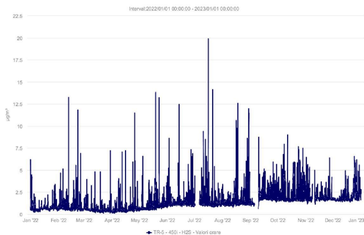
Fig. 5 Evoluția H 2 S în anul 2022 (concentrații medii orare)
