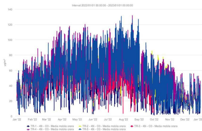
Fig. 4 Evoluția O 3 în anul 2022 (concentrații medii mobile)
