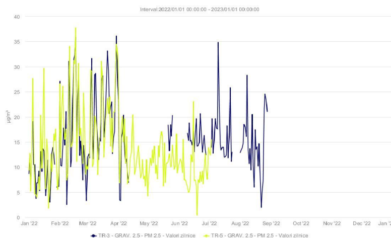
Fig. 8 Evoluția PM2.5 în anul 2022 (concentrații medii zilnice)
