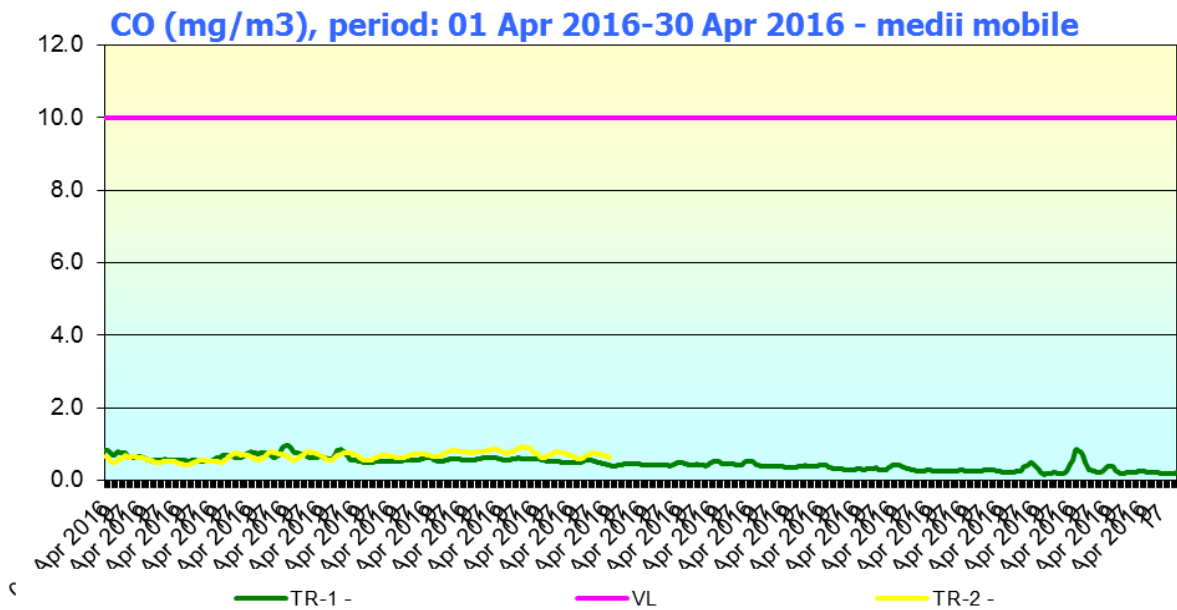
Fig. 1.3 - CO (mg/m 3 ), Aprilie 2016 - medii mobile
