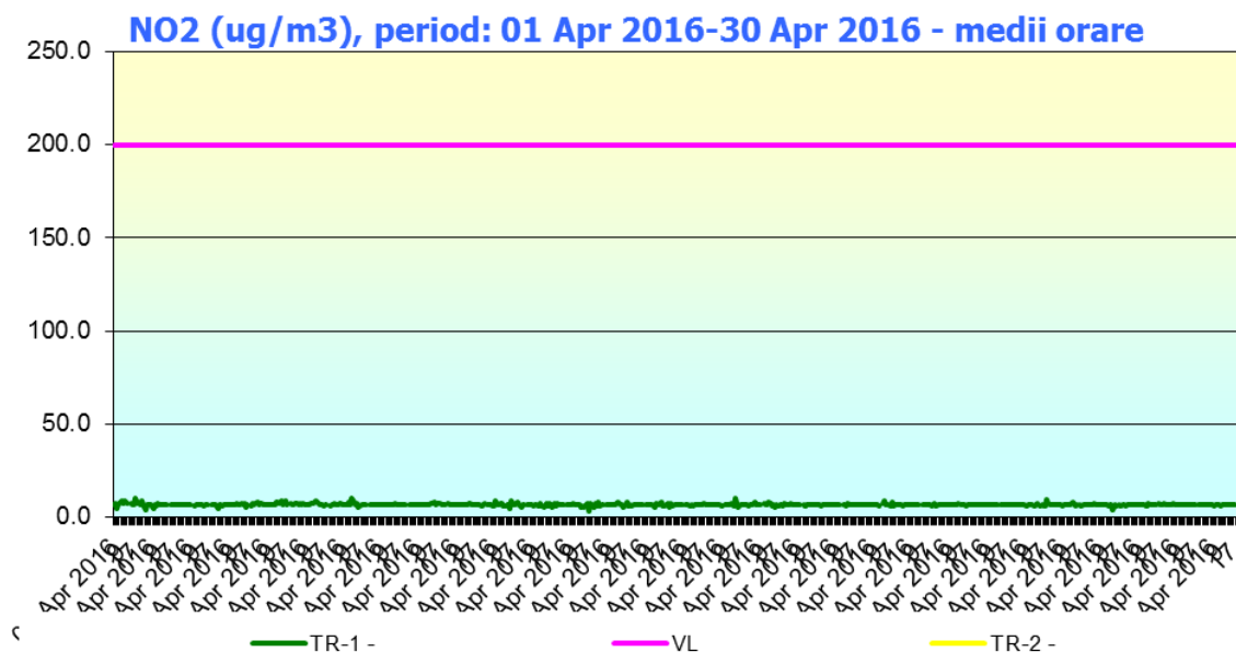
Fig. 1.1 - NO 2 (μg/m 3 ), Aprilie 2016 medii orare
