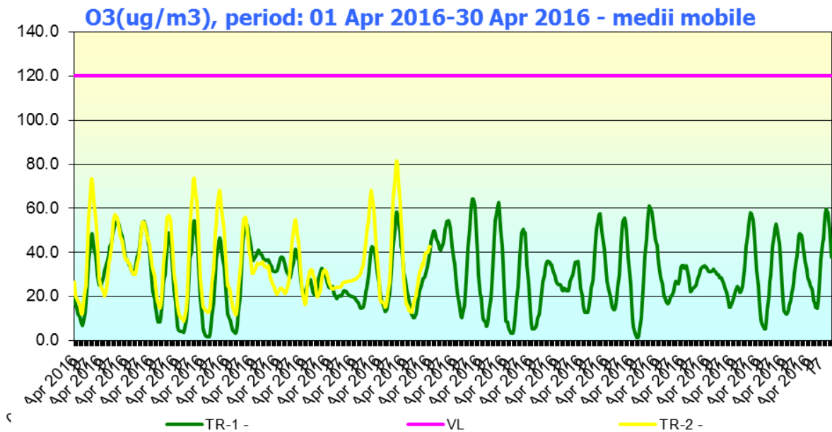
Fig. 1.2 - O 3 (µg/m 3 ), Aprilie 2016- medii mobile
