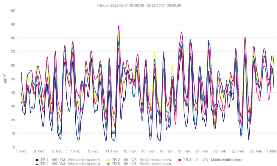
Fig. 1.3 - O 3 (µg/m 3 ) – Februarie2022
