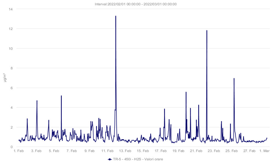
Fig. 1.5 – H 2 S (µg/m 3 ) – Februarie2022
