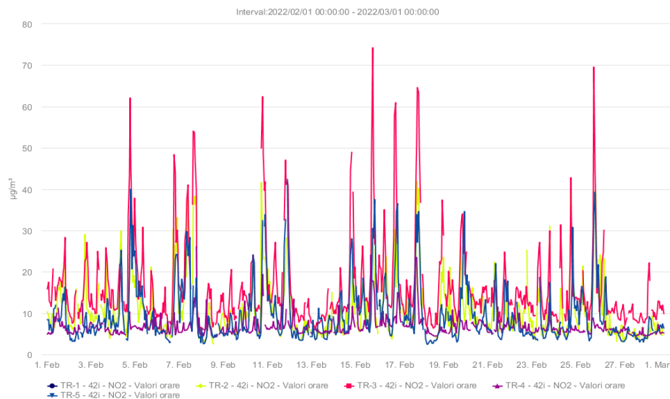
Fig. 1.2 - NO 2 (µg/m 3 ) – Februarie2022
