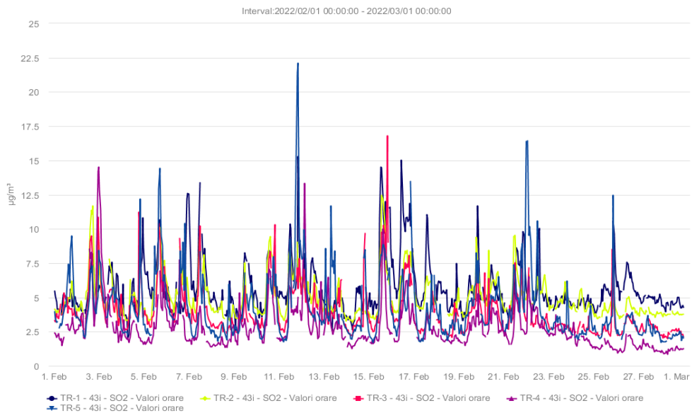
Fig. 1.1 - SO 2 (µg/m 3 ) – Februarie2022
