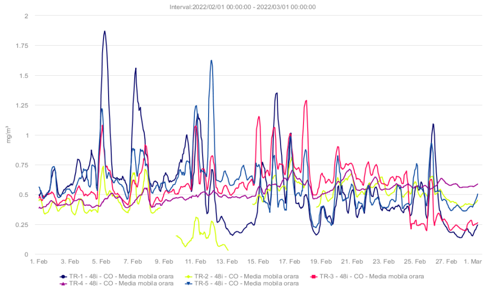
Fig. 1.4 - CO (mg/m 3 ) – Februarie2022
