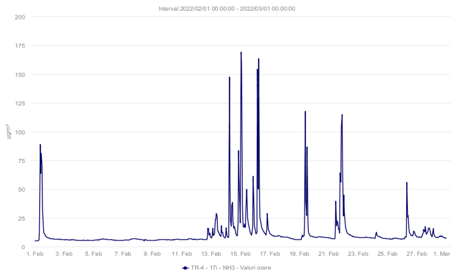
Fig. 1.6 – NH 3 (µg/m 3 ) – Februarie2022
