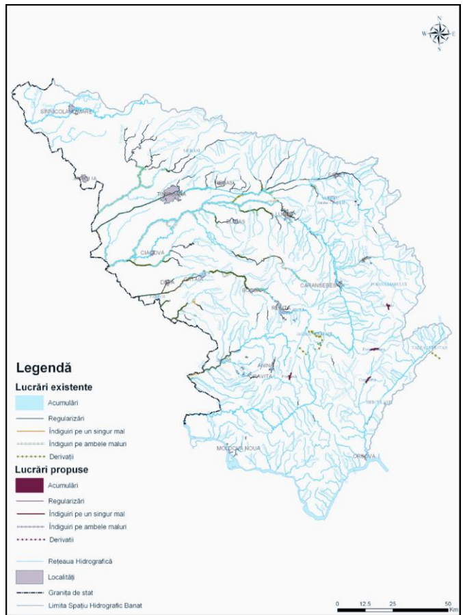
Figura II.1.1.4.1 - Lucrări hidrotehnice în Spațiul Hidrografic BANAT
