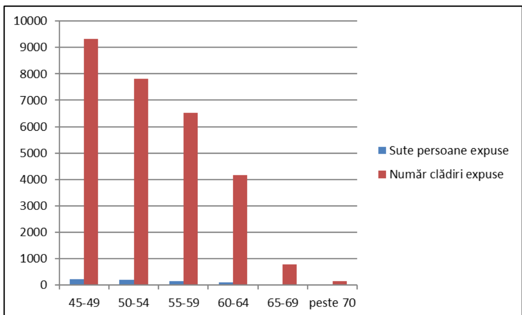
Fig. VIII.1.2.1.17. - Număr de persoane (sute) expuse și număr clădiri expuse la diferite intervale de valori ale indicatorului L_{noapte} pentru aglomerarea Timișoara, în total pentru toate tipurile de surse de zgomot trafic rutier, trafic feroviar, tramvai, industrie și trafic aerian
