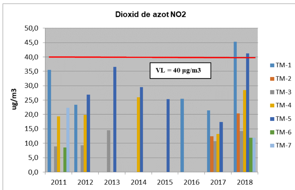
Figura nr. 1.12 – Concentrațiile medii anuale de dioxid de azot înregistrate în perioada 2011-2018
