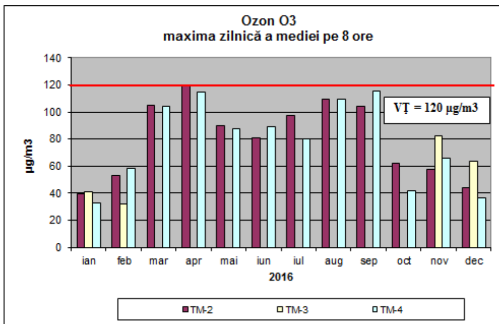
Figura nr. 7 – Concentrațiile maxime zilnice ale mediilor pe 8 de dioxid de ozon înregistrate în anul 2016
