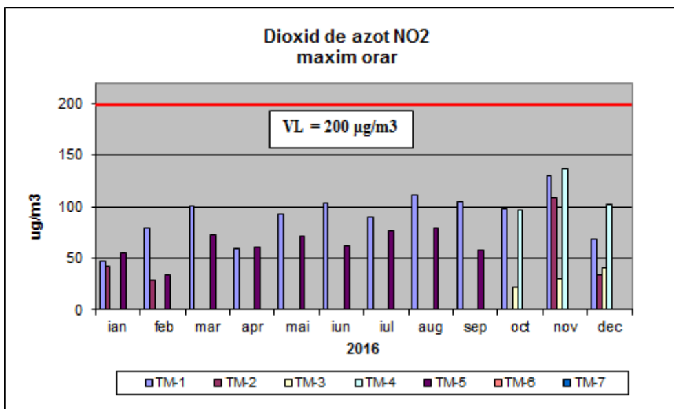
Figura nr. 3 – Concentrațiile maxime orare de dioxid de azot înregistrate în anul 2016
