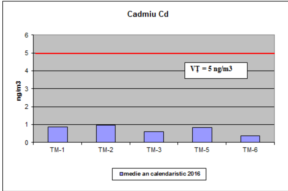
Figura nr. 13 – Concentrațiile medii anuale înregistrate în anul 2016
