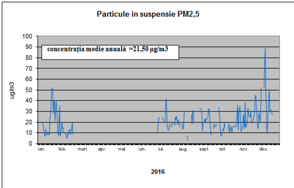
Figura nr. 10 – Concentrațiile medii pe 24 de ore de particule în suspensie PM 2,5 înregistrate în anul 2016
