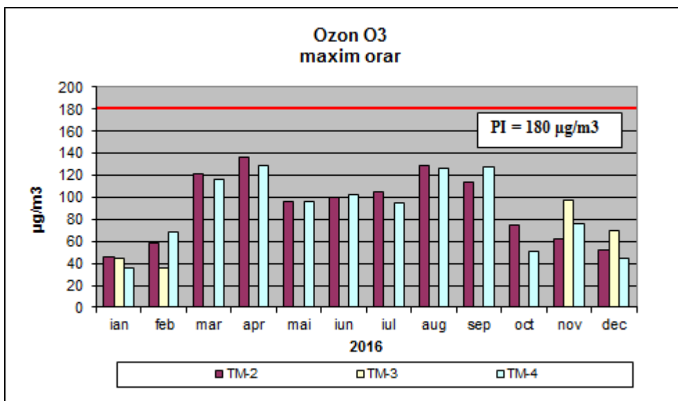
Figura nr. 6 – Concentrațiile maxime orare de ozon înregistrate în anul 2016
