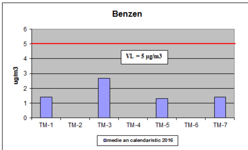
Figura nr. 8 – Concentrațiile medii anuale de benzen înregistrate în anul 2016
