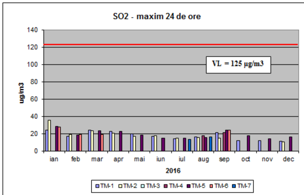
Figura nr. 2 – Concentrațiile maxime pe 24 de ore de dioxid de sulf înregistrate în anul 2016
