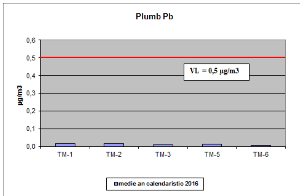
Figura nr. 11 – Concentrațiile medii anuale înregistrate în anul 2016
