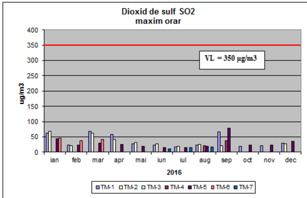
Figura nr. 1 – Concentrațiile maxime orare de dioxid de sulf înregistrate în anul 2016
