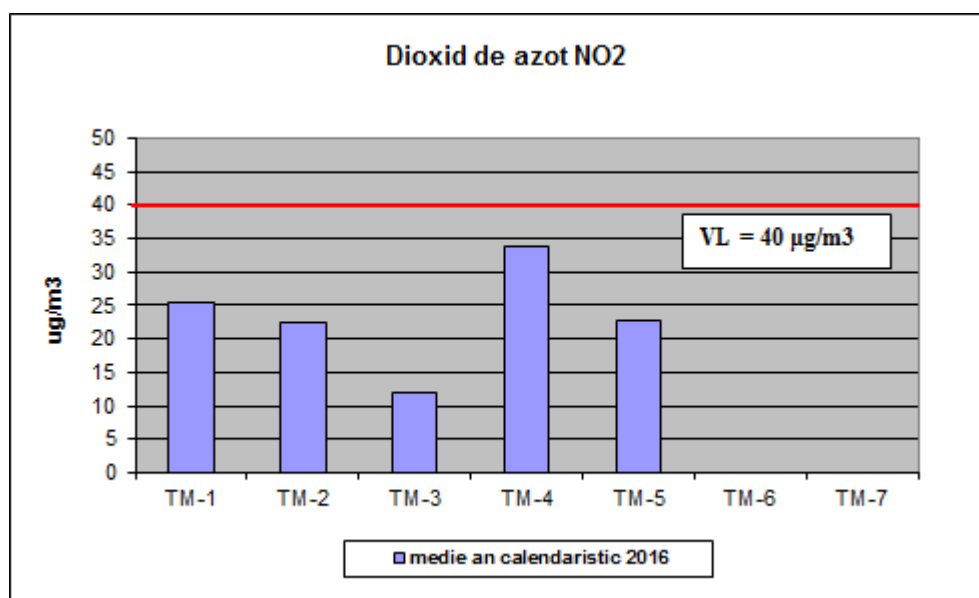
Figura nr. 4 – Concentrațiile medii anuale de dioxid de azot înregistrate în anul 2016
