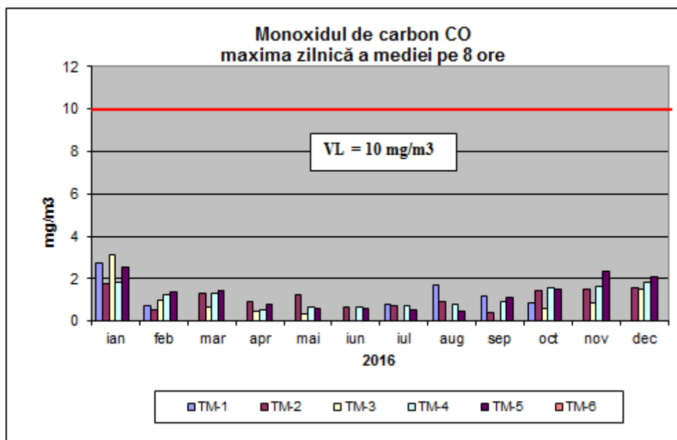
Figura nr. 5 – Concentrațiile maxime zilnice ale mediilor pe 8 de oxid de carbon înregistrate în anul 2016
