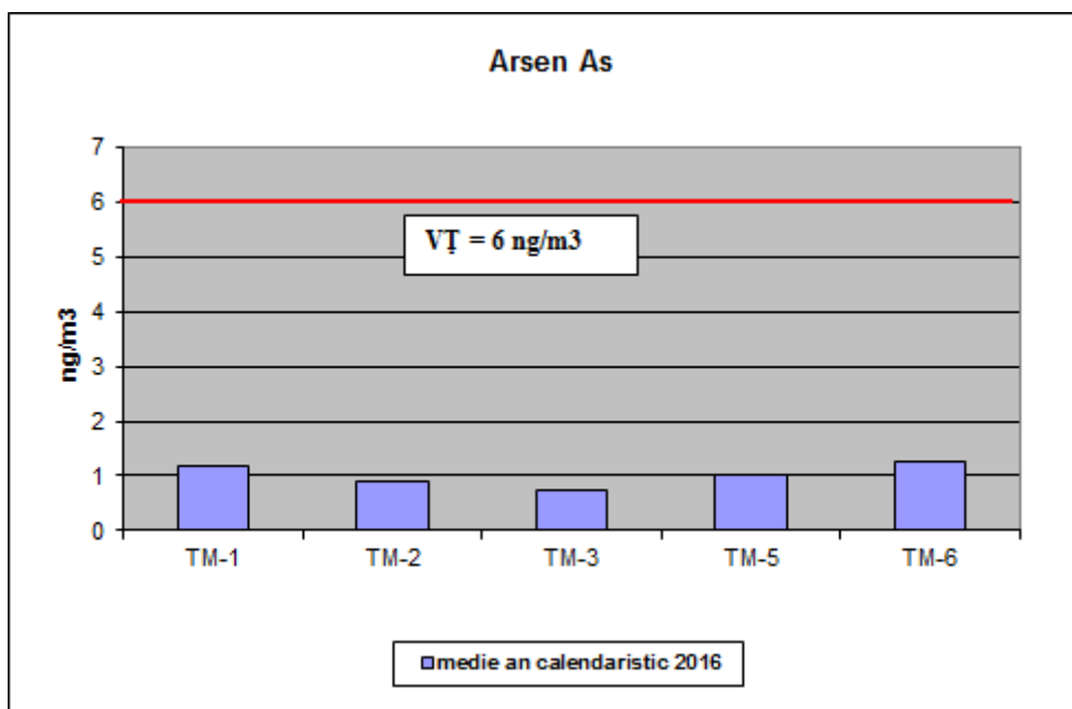
Figura nr. 14 – Concentrațiile medii anuale înregistrate în anul 2016
