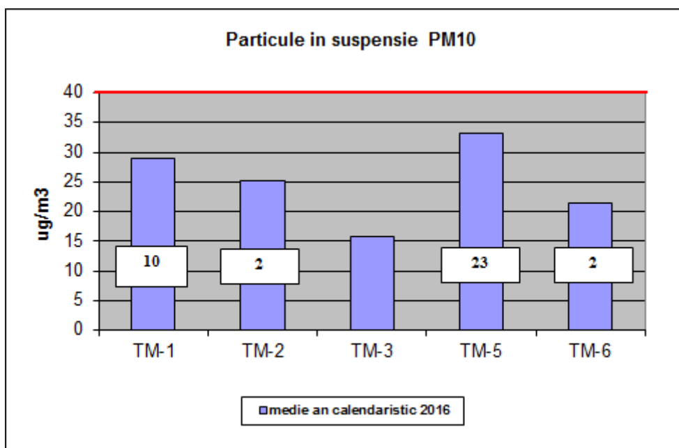
Figura nr. 9 – Concentrațiile medii anuale de PM 10 și numărul de determinări ce au depășit valoarea limită zilnică înregistrate în anul 2016
