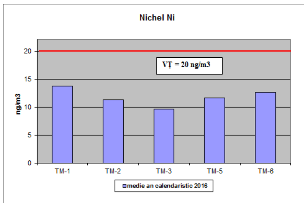
Figura nr. 12 – Concentrațiile medii anuale înregistrate în anul 2016
