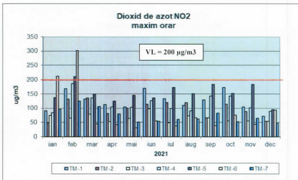
Figura nr. 3 – Concentrațiile maxime orare de dioxid de azot înregistrate în anul 2021
