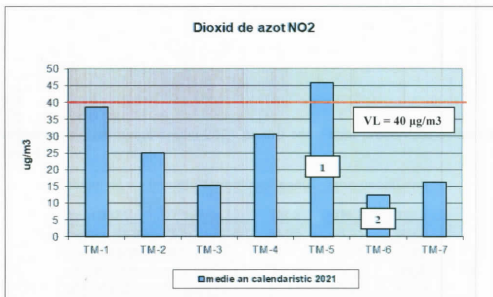
Figura nr. 4 – Concentrațiile medii anuale de dioxid de azot și numărul de determinări ce au depășit valoarea limită orară înregistrate în anul 2021
