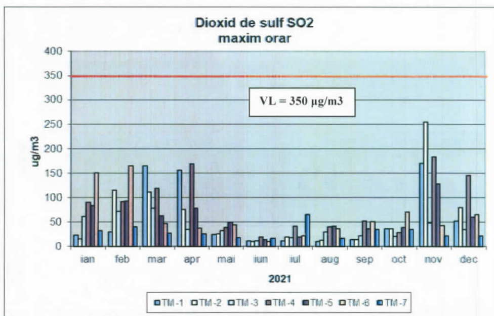
Figura nr. 1 – Concentrațiile maxime orare de dioxid de sulf înregistrate în anul 2021
