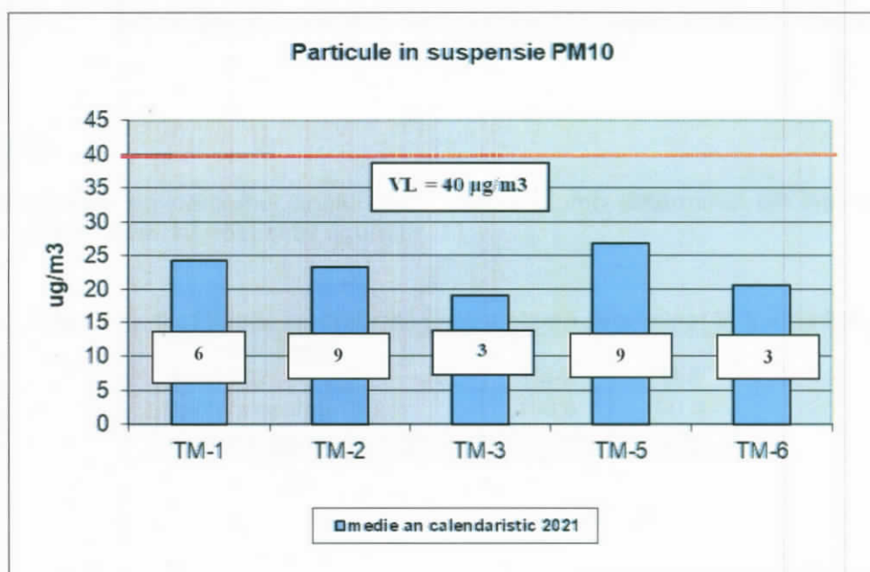
Figura nr. 9 – Concentrațiile medii anuale de PM 10 și numărul de determinări ce au depășit valoarea limită zilnică înregistrate în anul 2021
