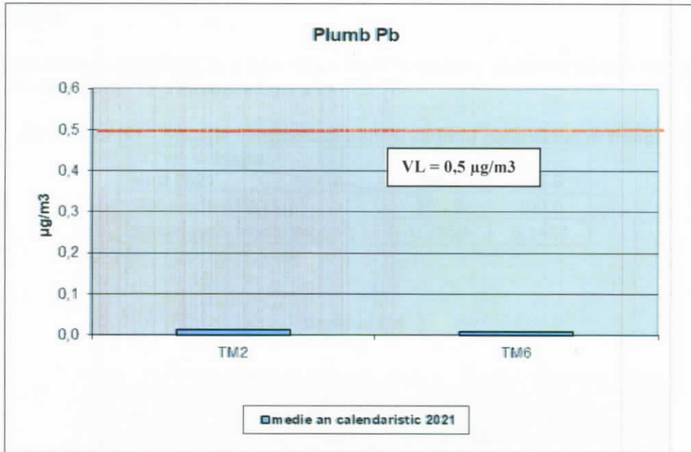
Figura nr. 11 – Concentrațiile medii anuale înregistrate în anul 2021
