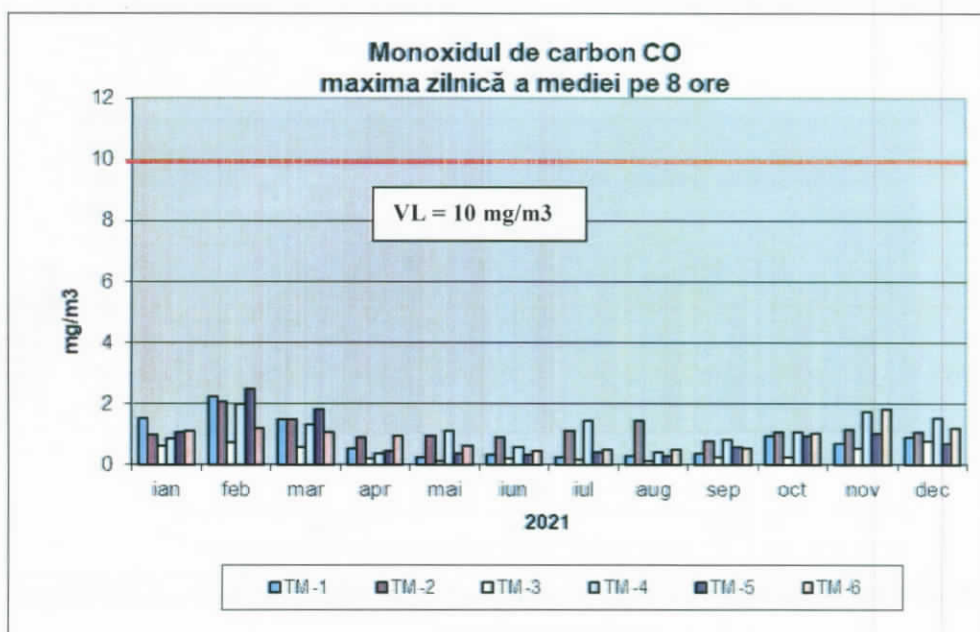
Figura nr. 5 – Concentrațiile maxime zilnice ale mediilor pe 8 ore de oxid de carbon înregistrate în anul 2021
