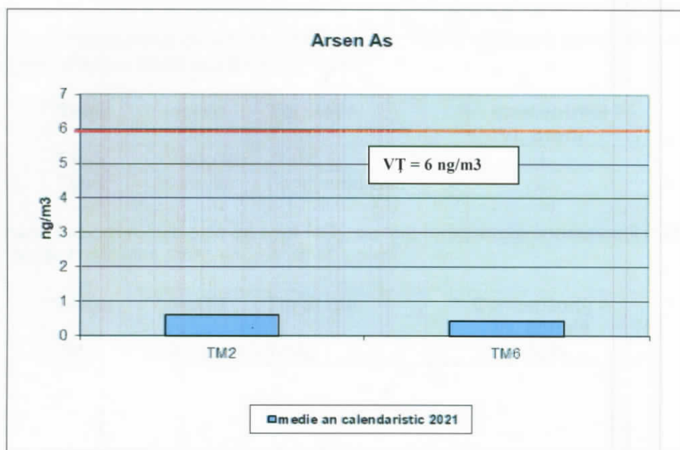
Figura nr. 14 – Concentrațiile medii anuale înregistrate în anul 2021
