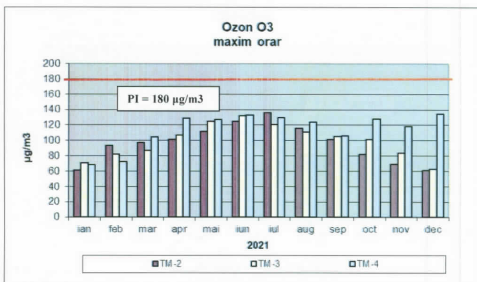
Figura nr. 6 – Concentrațiile maxime orare de ozon înregistrate în anul 2021
