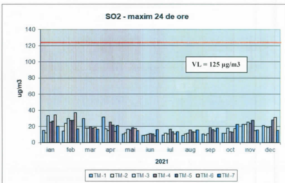
Figura nr. 2 – Concentrațiile maxime pe 24 de ore de dioxid de sulf înregistrate în anul 2021
