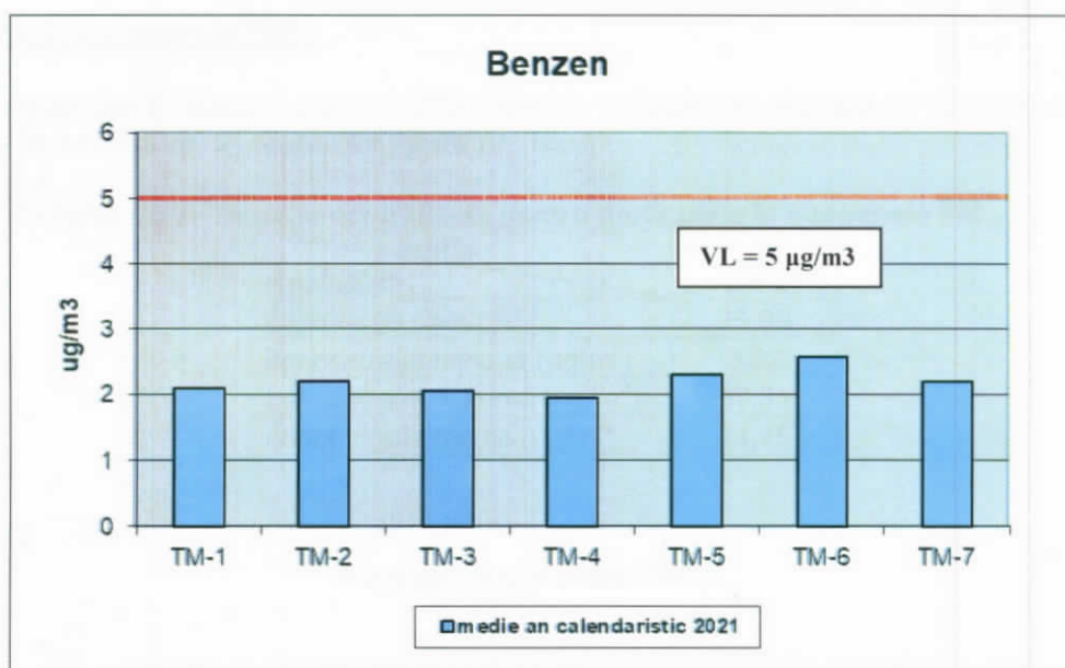
Figura nr. 8 – Concentrațiile medii anuale de benzen înregistrate în anul 2021
