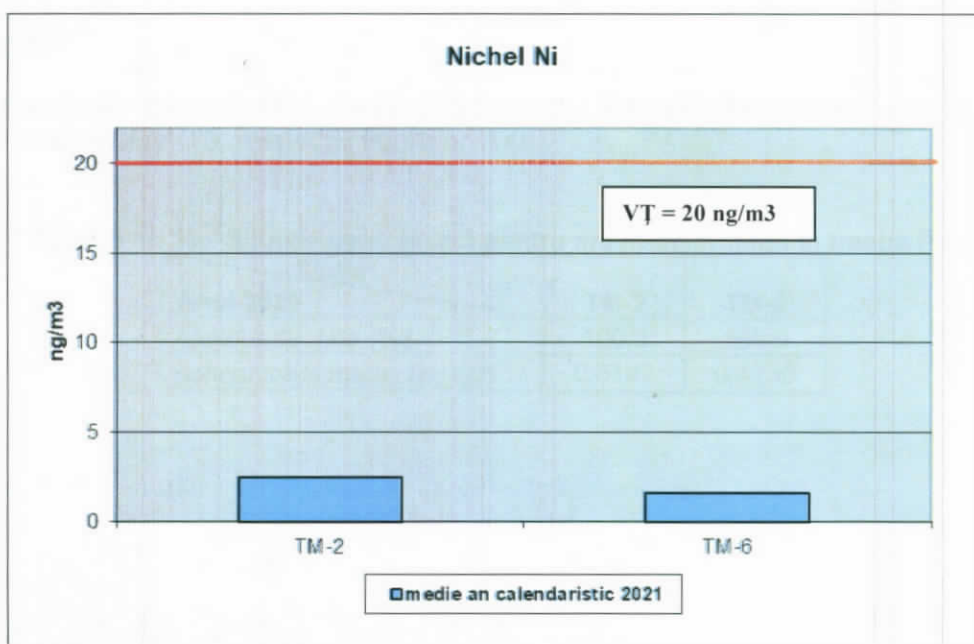
Figura nr. 12 – Concentrațiile medii anuale înregistrate în anul 2021
