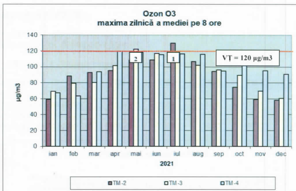
Figura nr. 7 – Concentrațiile maxime zilnice ale mediilor pe 8 ore de dioxid de ozon și numărul de determinări ce au depășit valoarea țintă înregistrate în anul 2021
