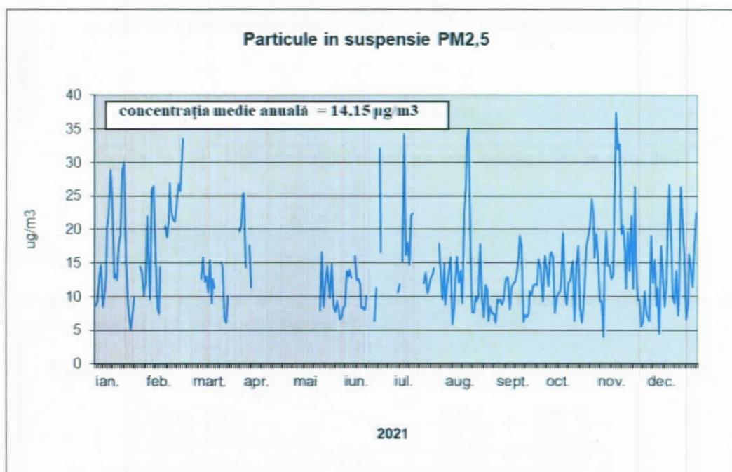
Figura nr. 10 – Concentrațiile medii pe 24 de ore de particule în suspensie PM 2,5 înregistrate în anul 2021
