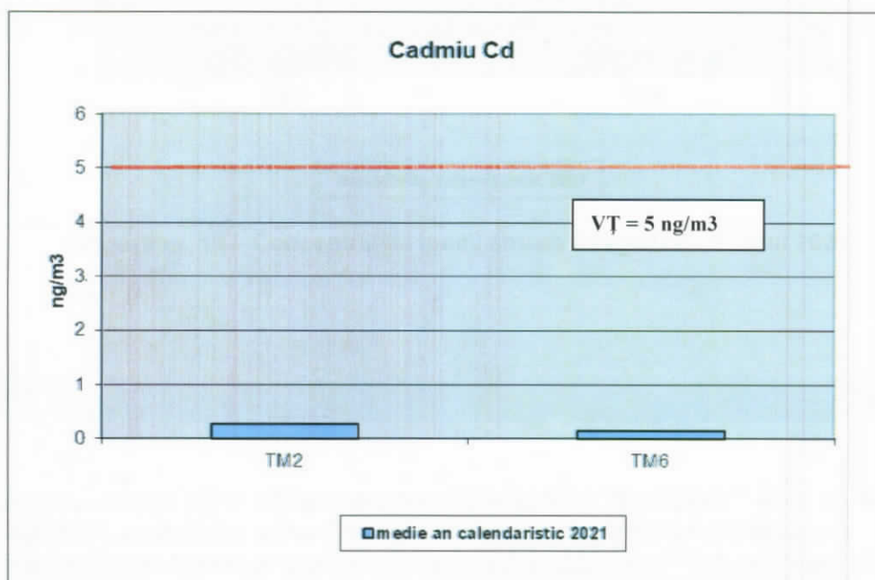
Figura nr. 13 – Concentrațiile medii anuale înregistrate în anul 2021
