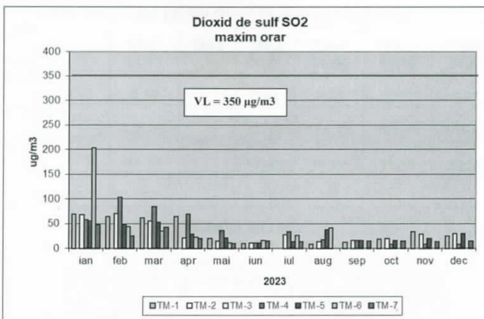
Figura nr. 1 - Concentrațiile maxime orare de dioxid de sulf înregistrate în anul 2023
