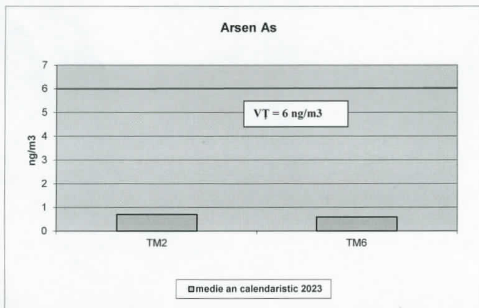
Figura nr. 14 - Concentrațiile medii anuale înregistrate în anul 2023
