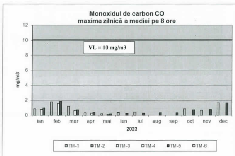
Figura nr. 5 - Concentrațiile maxime zilnice ale mediilor pe 8 ore de oxid de carbon înregistrate în anul 2023
