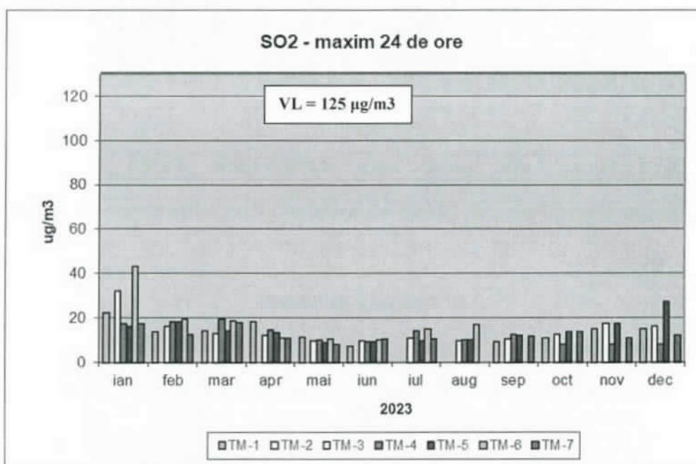
Figura nr. 2 - Concentrațiile maxime pe 24 de ore de dioxid de sulf înregistrate în anul 2023
