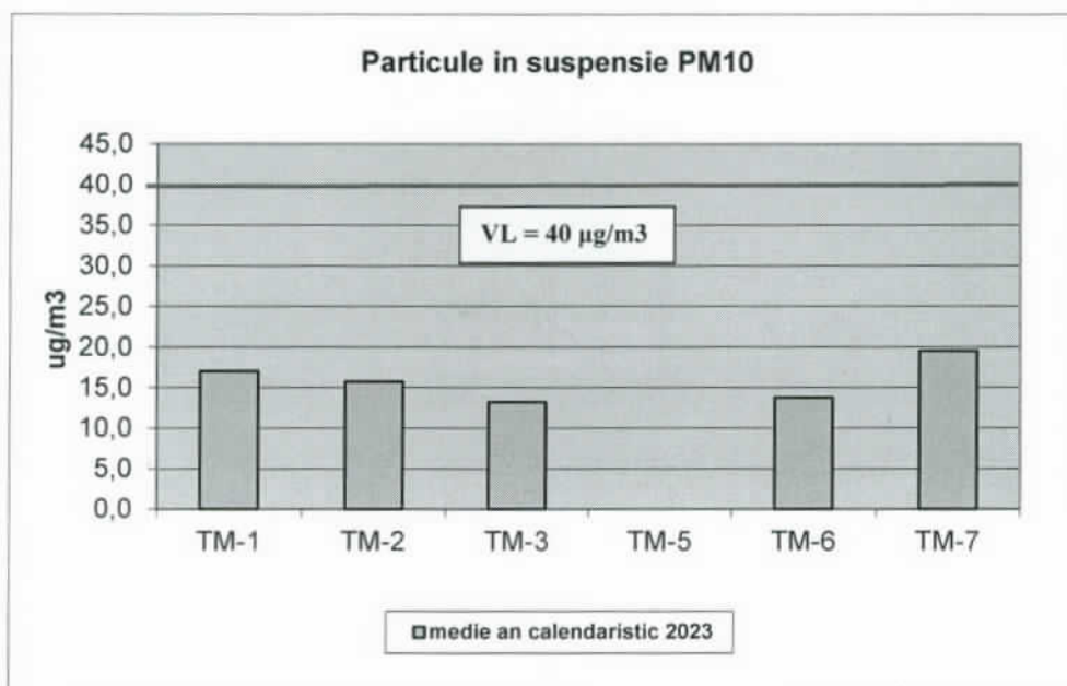
Figura nr. 9 - Concentrațiile medii anuale de PM 10 și numărul de determinări ce au depășit valoarea limită zilnică înregistrate în anul 2023
