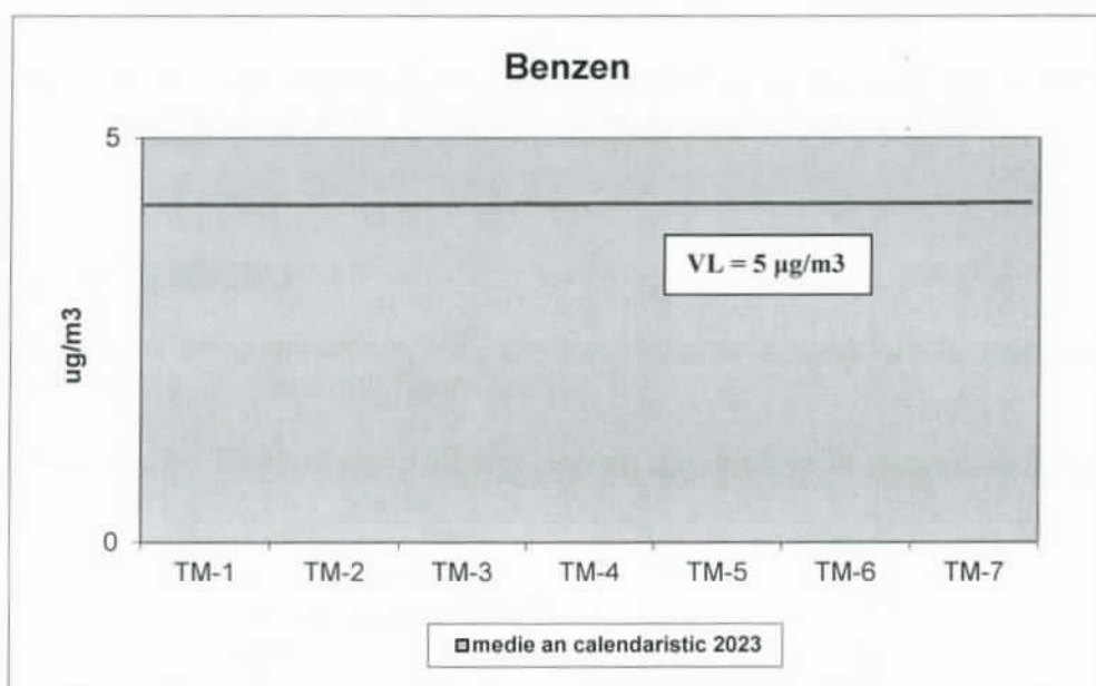
Figura nr. 8 - Concentrațiile medii anuale de benzen înregistrate în anul 2023
