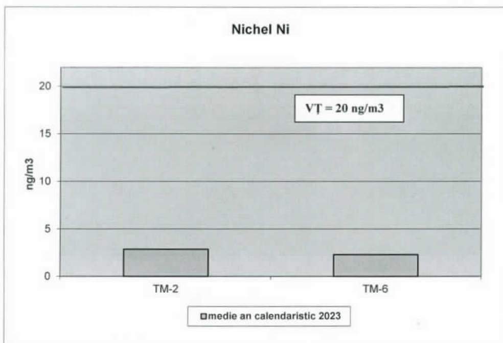
Figura nr. 12 - Concentrațiile medii anuale înregistrate în anul 2023
