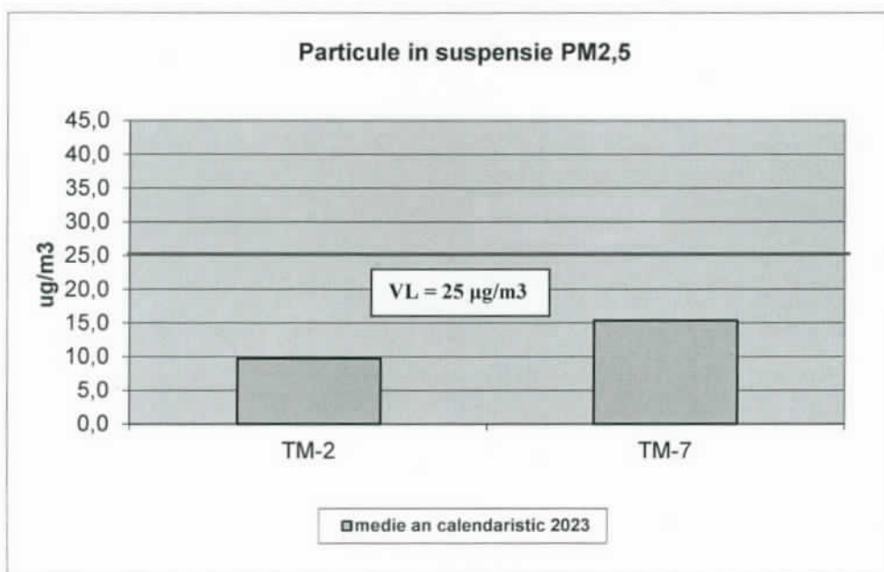
Figura nr. 10 - Concentrații medii anuale de PM 2,5 înregistrate în anul 2023
