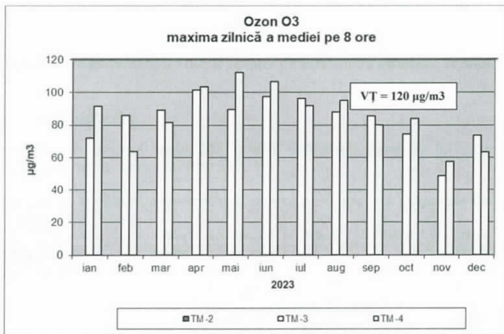
Figura nr. 7 - Concentrațiile maxime zilnice ale mediilor pe 8 ore de dioxid de ozon și numărul de determinări ce au depășit valoarea țintă înregistrate în anul 2023
