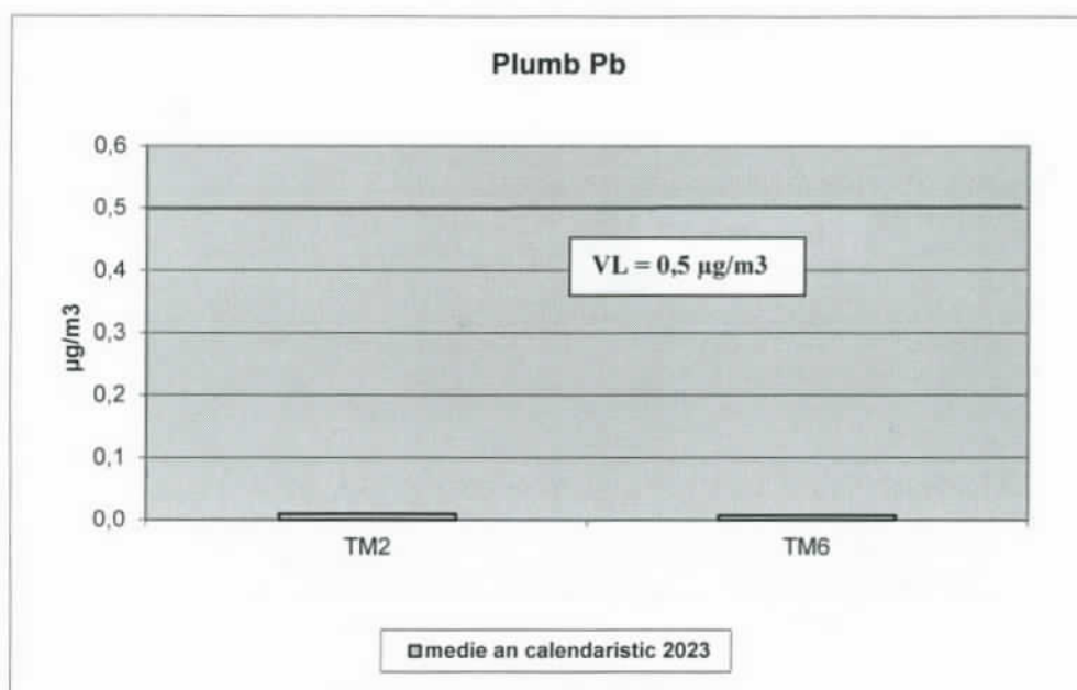
Figura nr. 11 - Concentrațiile medii anuale înregistrate în anul 2023
