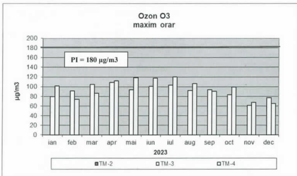
Figura nr. 6 - Concentrațiile maxime orare de ozon înregistrate în anul 2023
