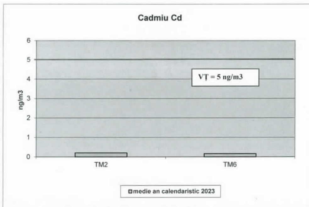
Figura nr. 13 - Concentrațiile medii anuale înregistrate în anul 2023
