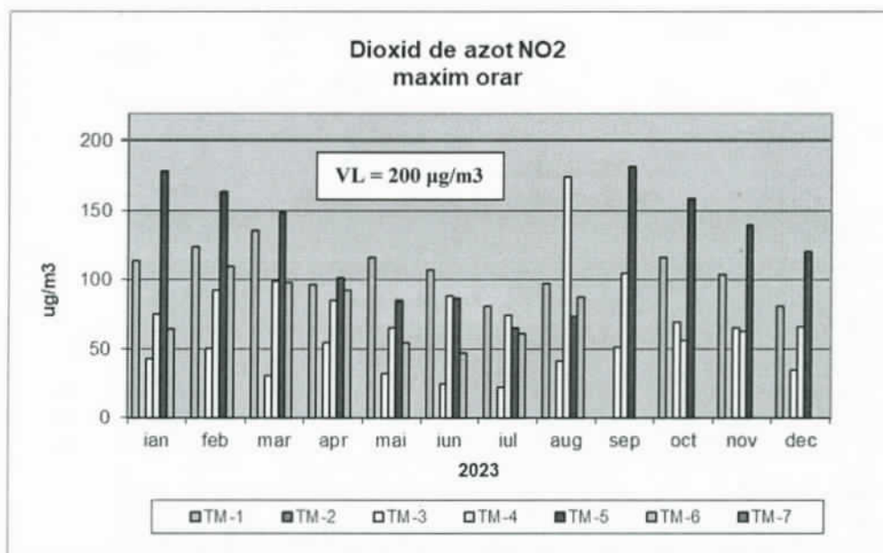
Figura nr. 3 - Concentrațiile maxime orare de dioxid de azot înregistrate în anul 2023
