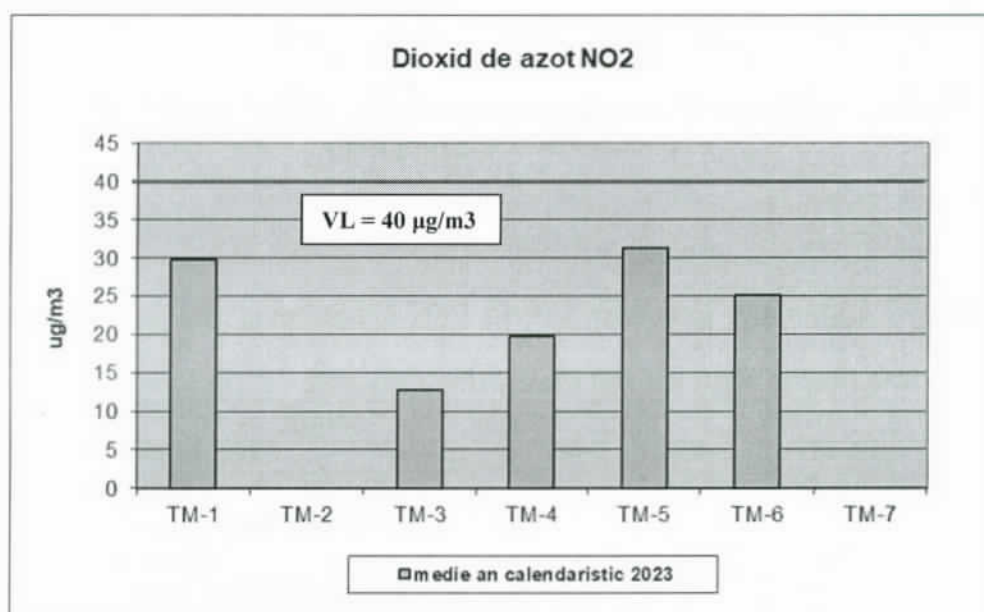
Figura nr. 4 - Concentrațiile medii anuale de dioxid de azot și numărul de determinări ce au depășit valoarea limită orară înregistrate în anul 2023
